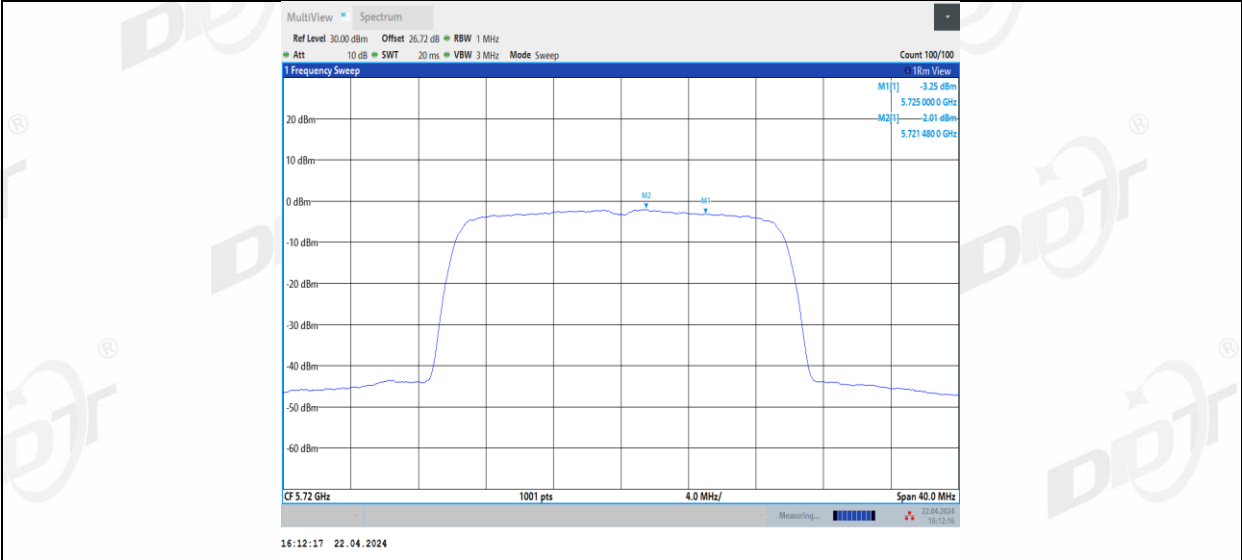
11BE20MIMO_Ant1_5720_UNII-3
