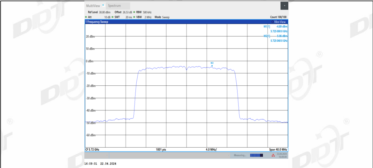
11BE20MIMO_Ant2_5720_UNII-3
