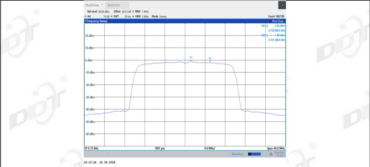
11BE20MIMO_Ant3_5720_UNII-2C
