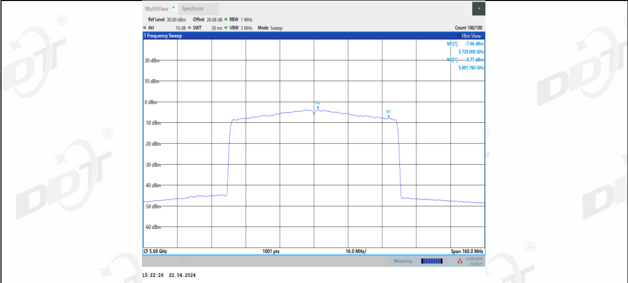
11AX80MIMO_Ant3_5690_UNII-2C
