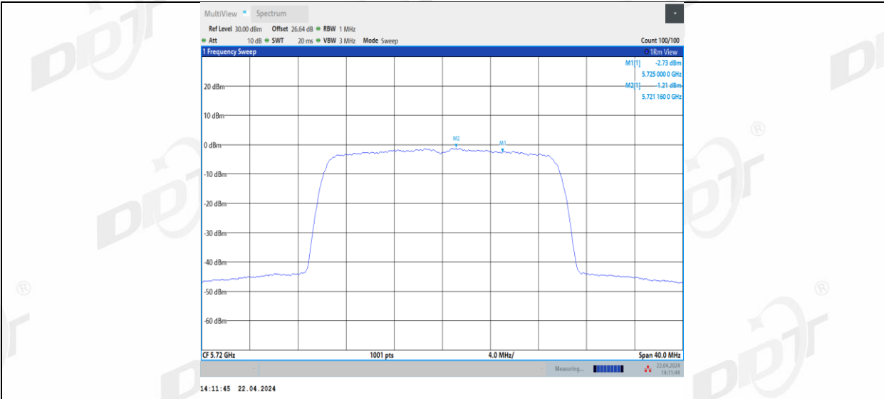
11AX20MIMO_Ant2_5720_UNII-2C
