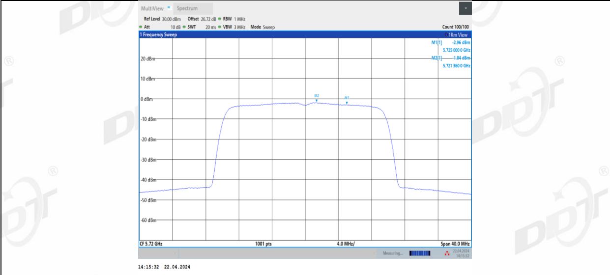
11AX20MIMO_Ant1_5720_UNII-3
