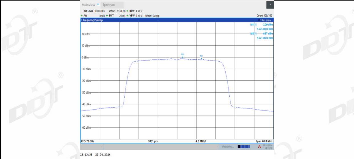
11AX20MIMO_Ant3_5720_UNII-2C
