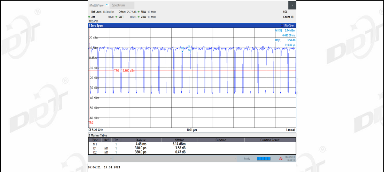
11AX20MIMO_Ant3_5240
