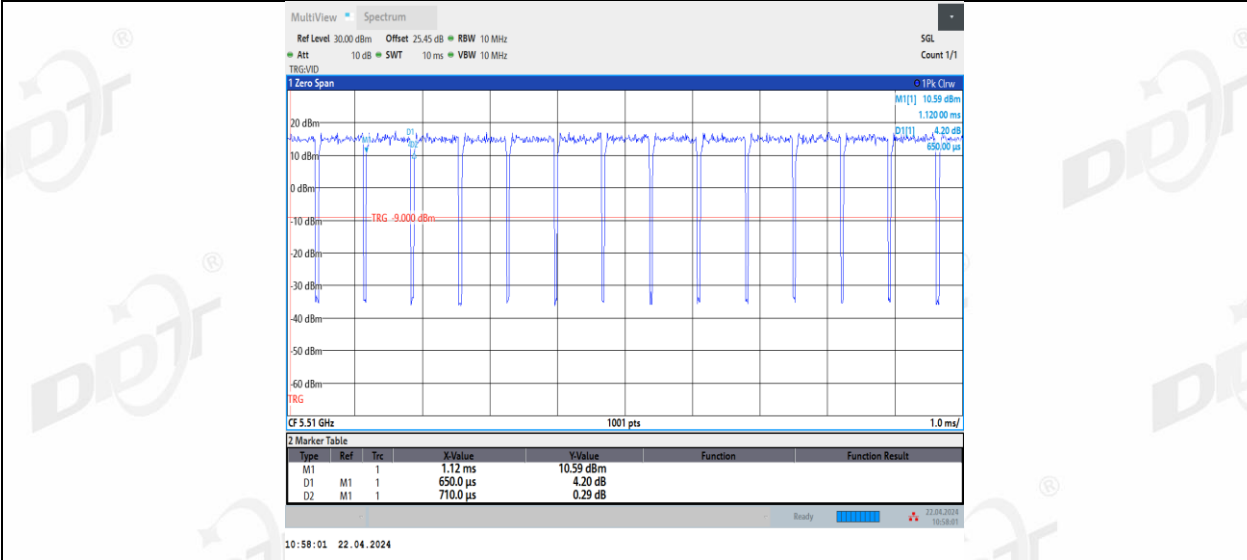
11AC40MIMO_Ant3_5510
