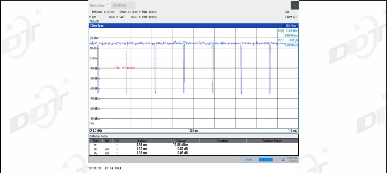
11AC20MIMO_Ant3_5700
