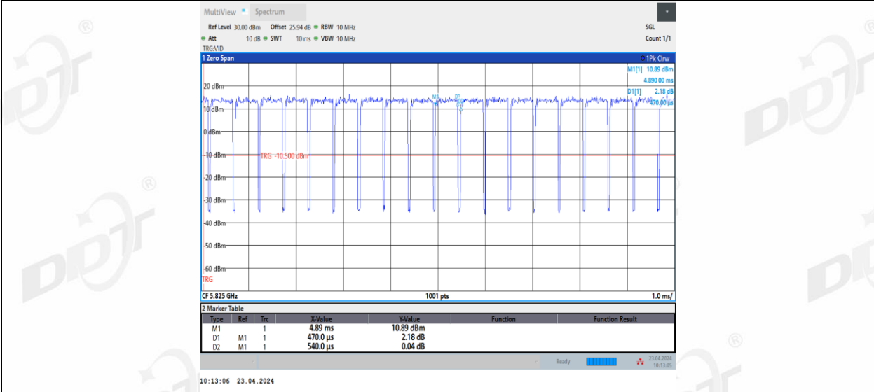
11N20MIMO_Ant3_5825
