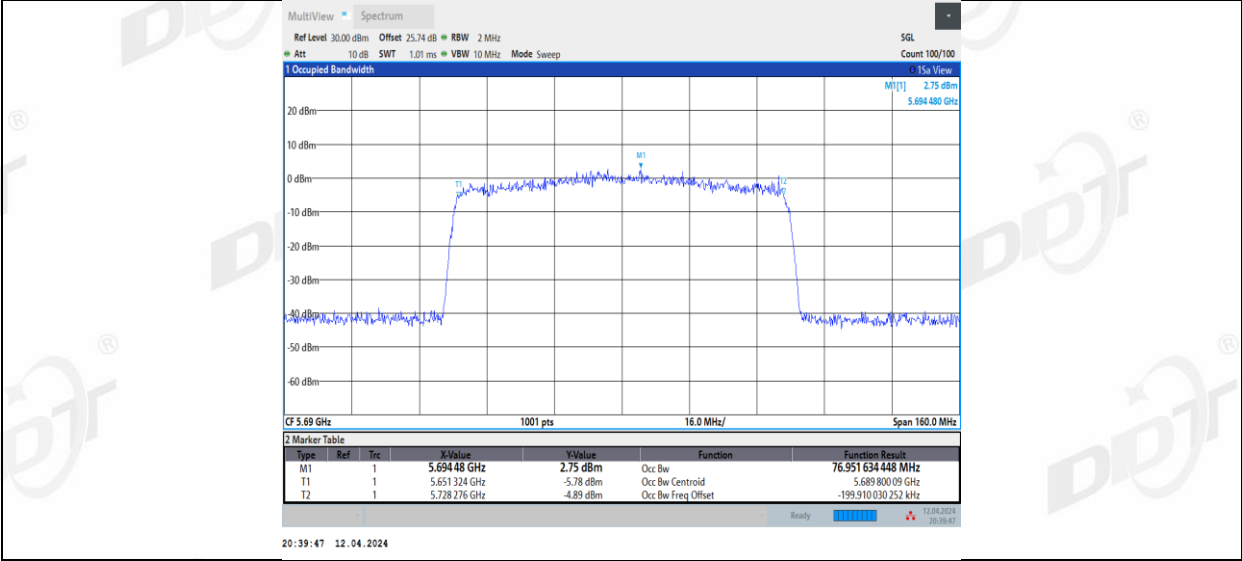
11BE80MIMO_Ant2_5690
