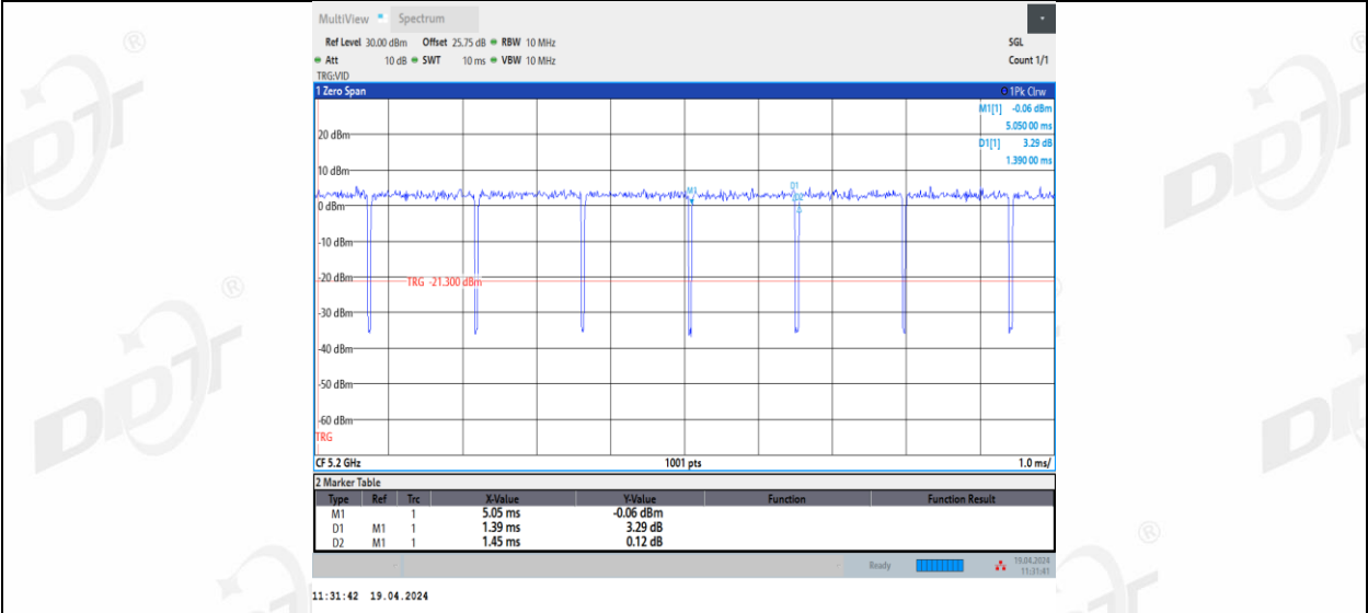
11A-CDD_Ant3_5200
