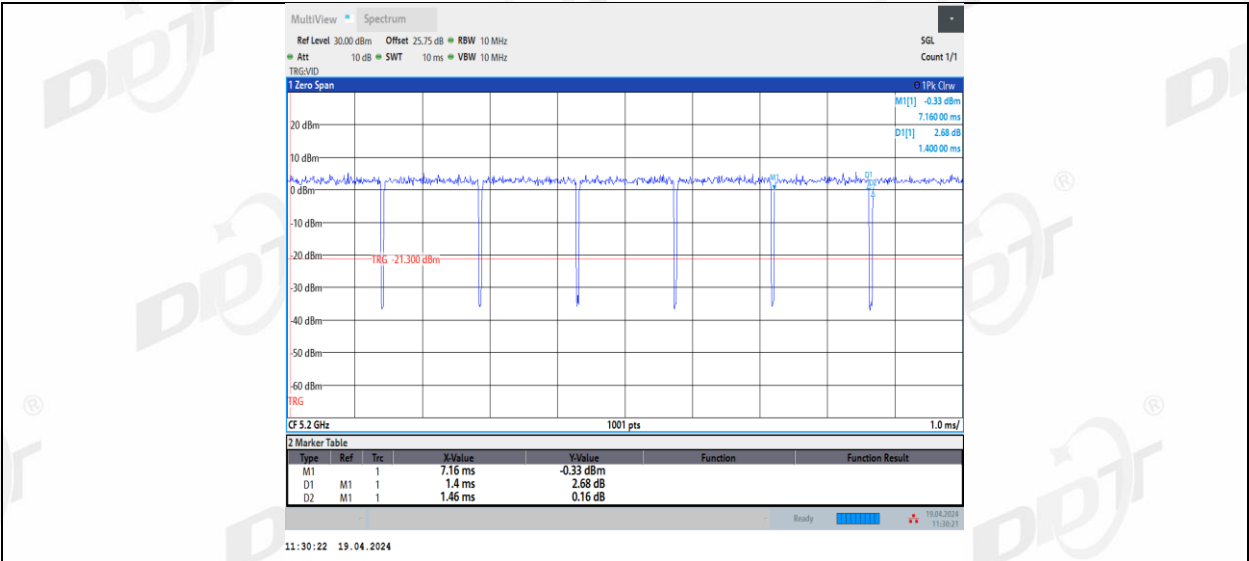
11A-CDD_Ant2_5200
