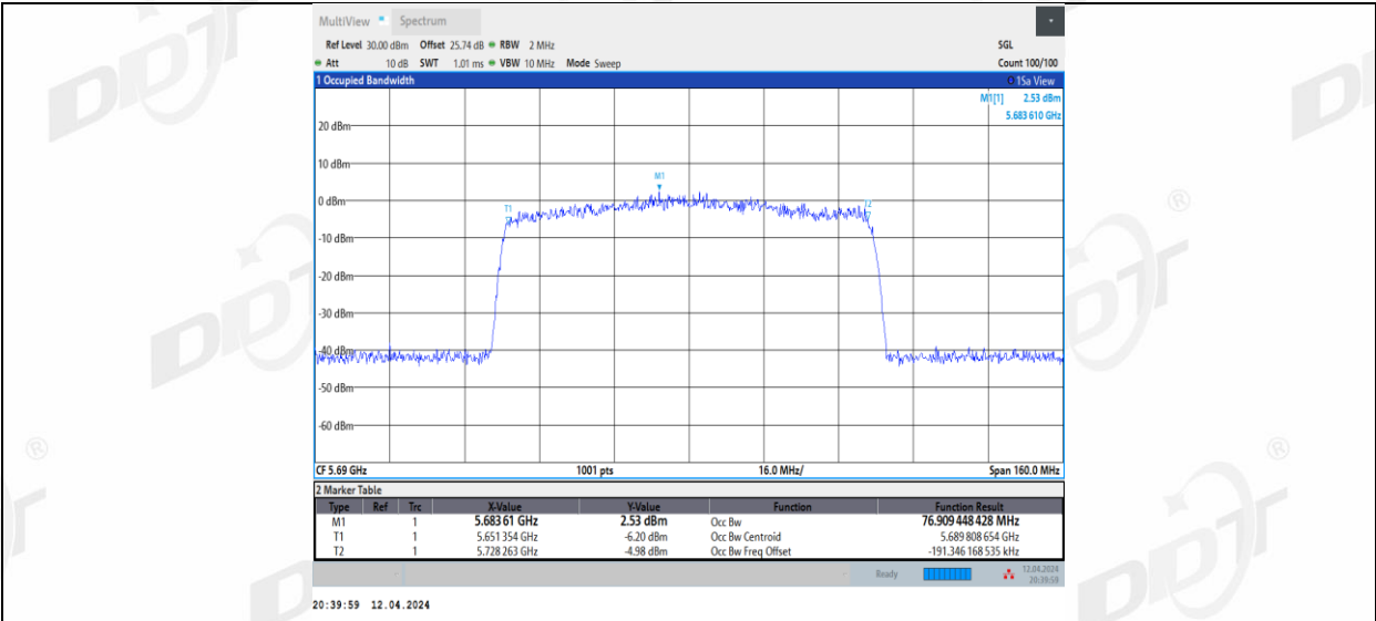
11BE80MIMO_Ant3_5690
