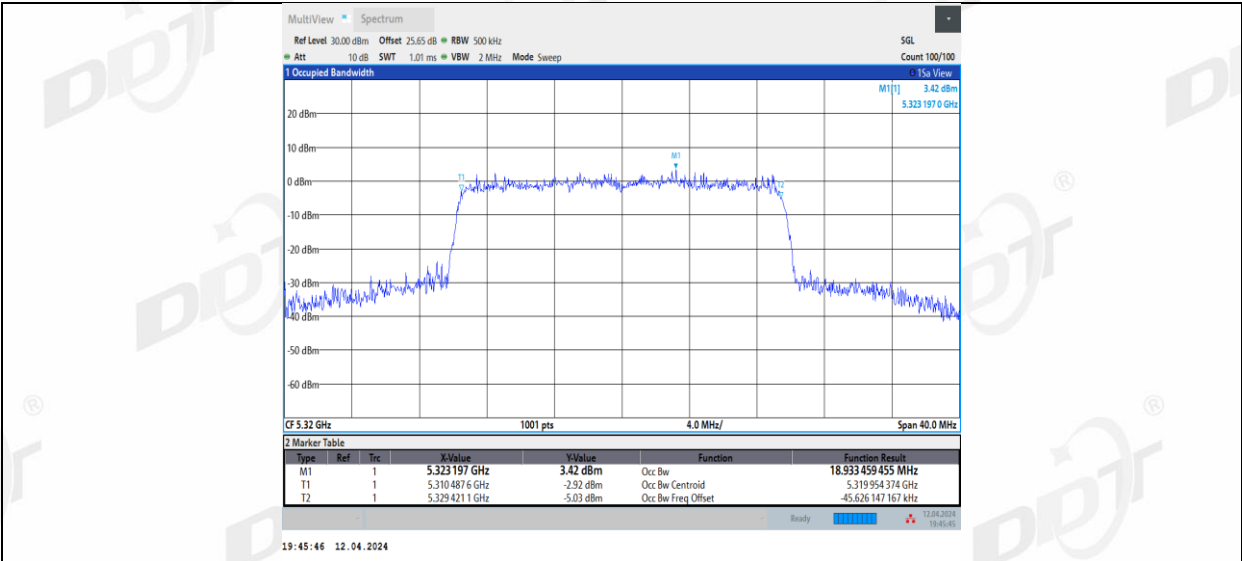
11AX20MIMO_Ant3_5320
