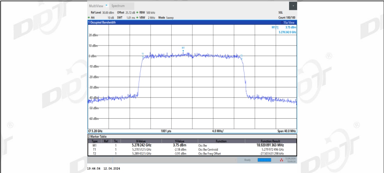
11AX20MIMO_Ant3_5280
