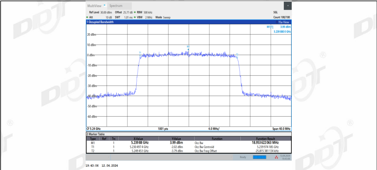
11AX20MIMO_Ant3_5240
