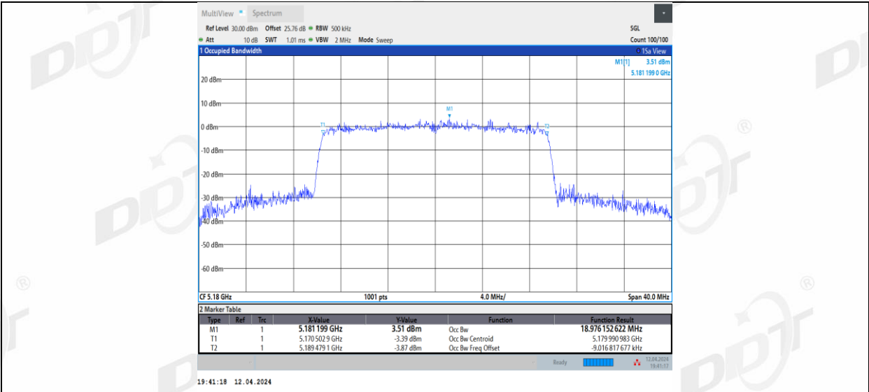
11AX20MIMO_Ant3_5180
