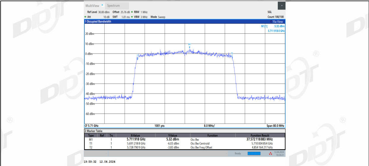
11AX40MIMO_Ant3_5710
