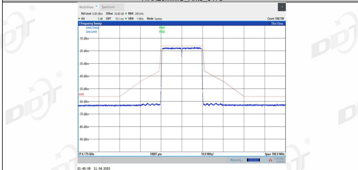
11AX20MIMO_Ant4_6175
