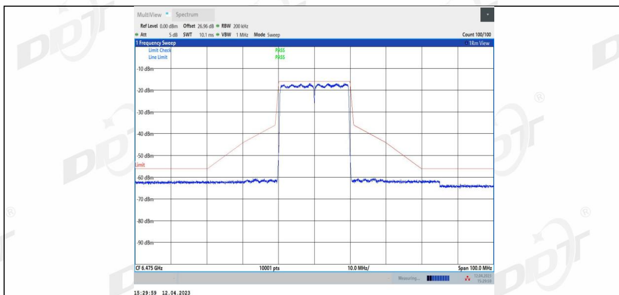
11AX20MIMO_Ant3_6475
