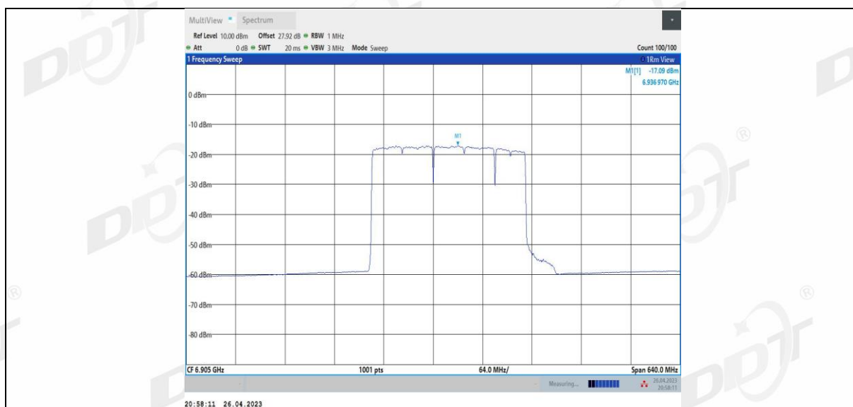
11BE320MIMO_Ant4_6905_3*996_1
