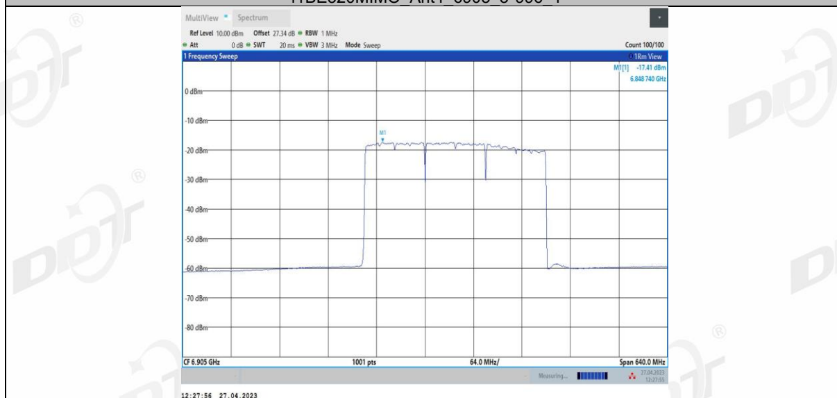
11BE320MIMO_Ant4_6905_3*996_2
