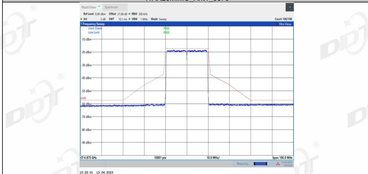
11AX20MIMO_Ant2_6875
