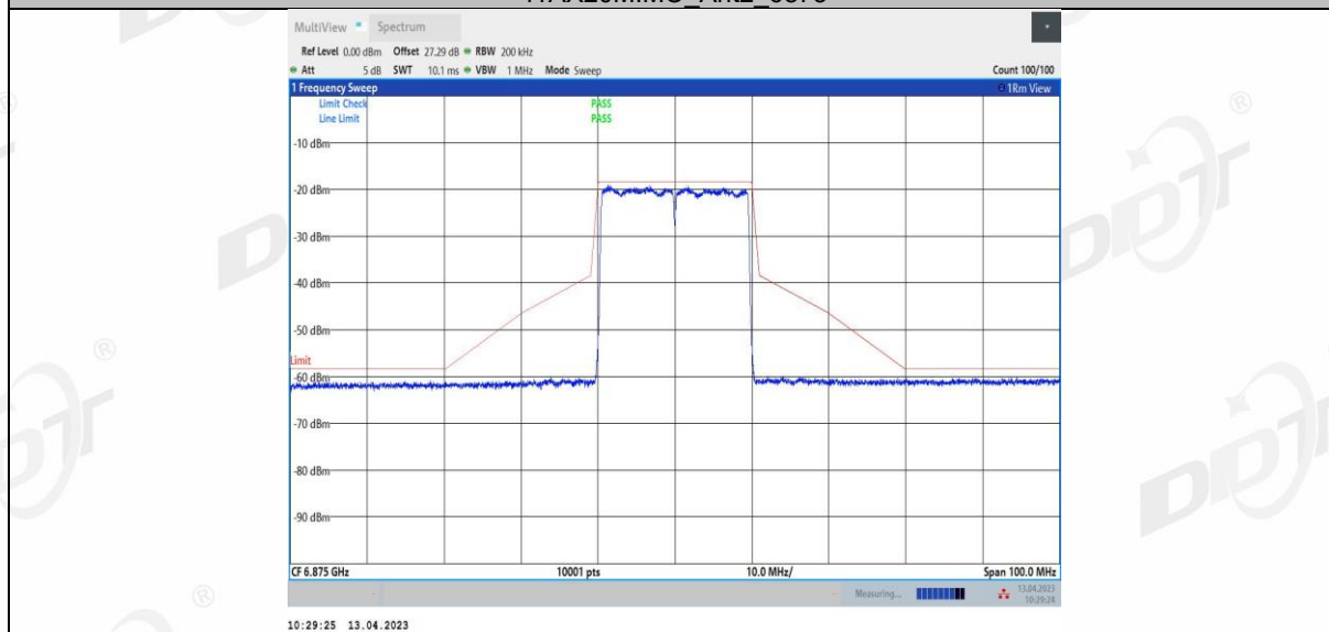
11AX20MIMO_Ant3_6875
