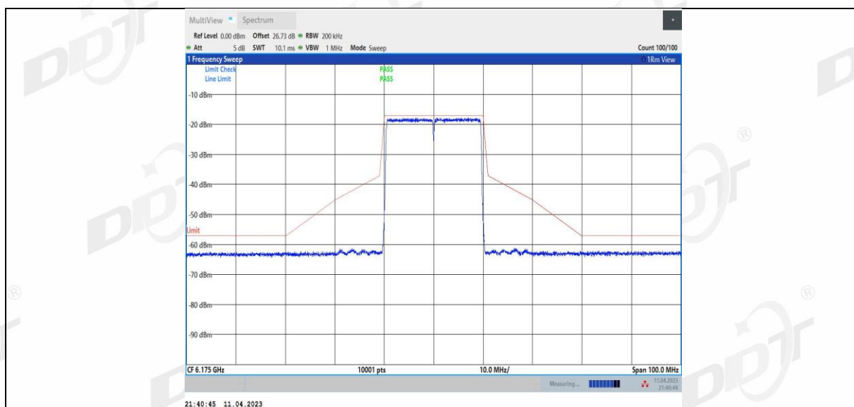
11AX20MIMO_Ant3_6175
