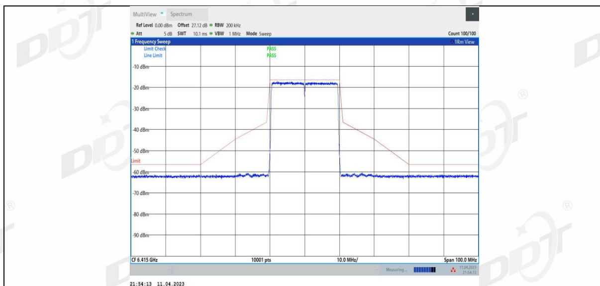
11AX20MIMO_Ant2_6415
