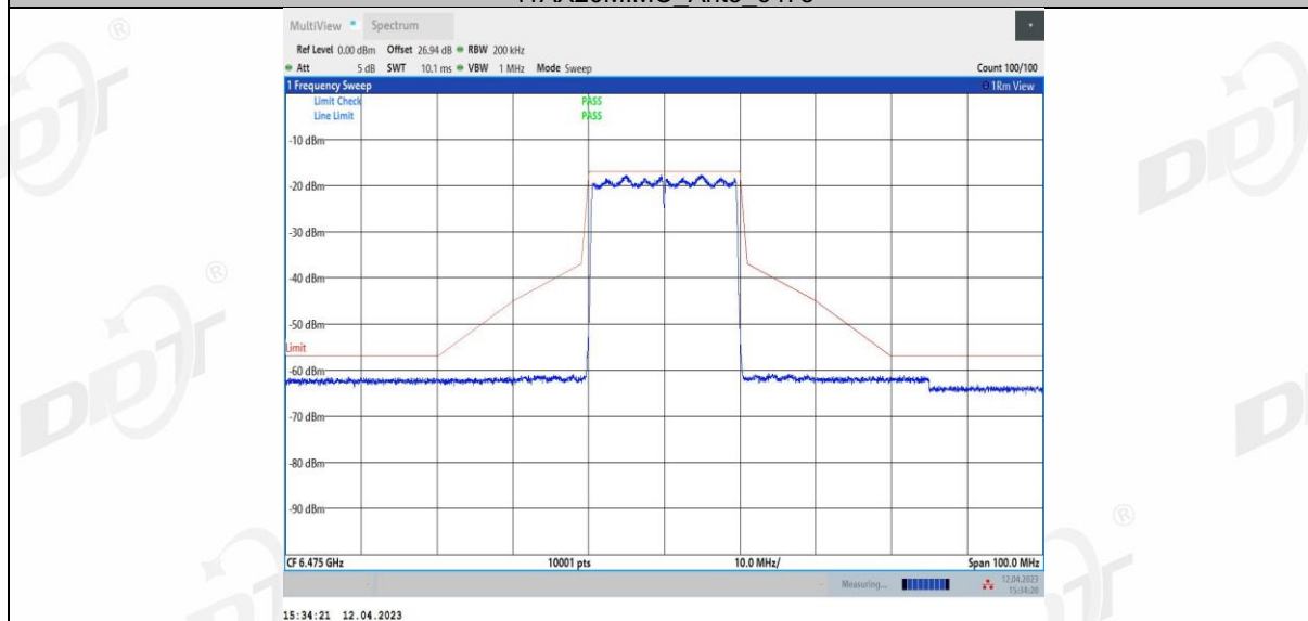
11AX20MIMO_Ant4_6475
