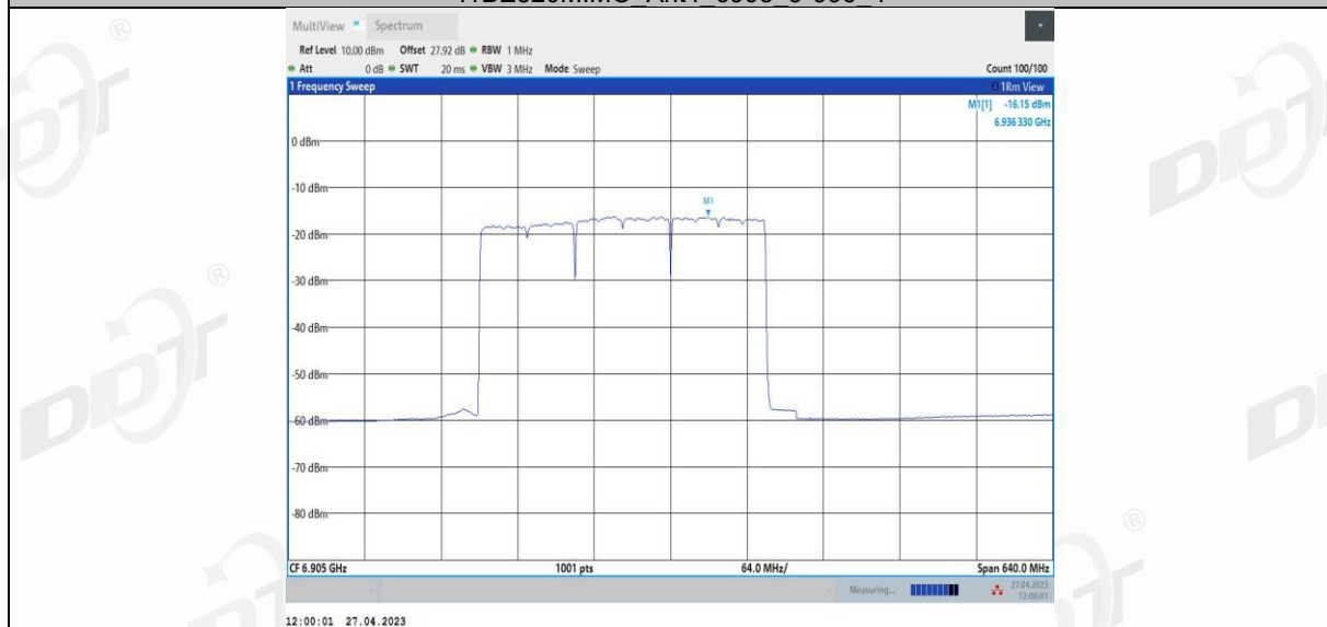
11BE320MIMO Ant4 6905 3*996+484 5
