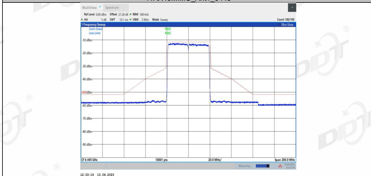
11AX40MIMO_Ant2_6445
