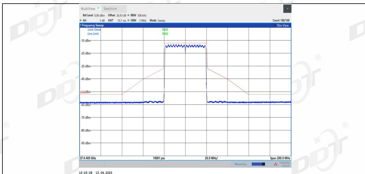
11AX40MIMO_Ant4_6405
