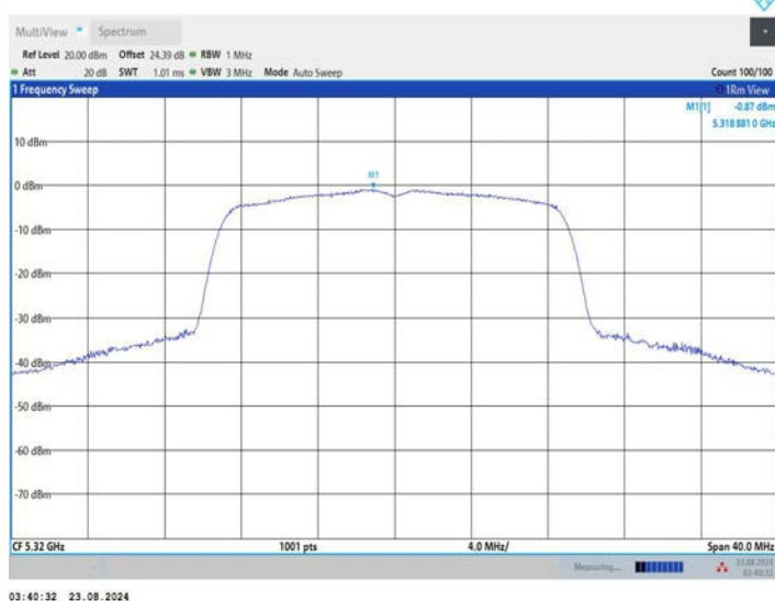
11AC20MIMO_Ant3_5320
