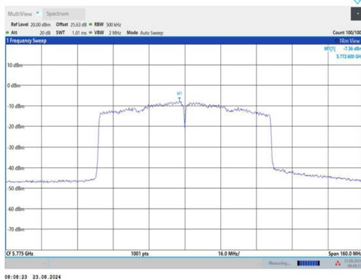
11AC80MIMO_Ant3_5775
