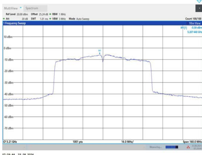
11AC80MIMO_Ant3_5210
