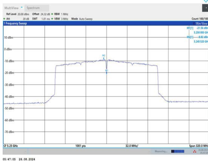
11AX160MIMO_Ant3_5250_UNII-1
