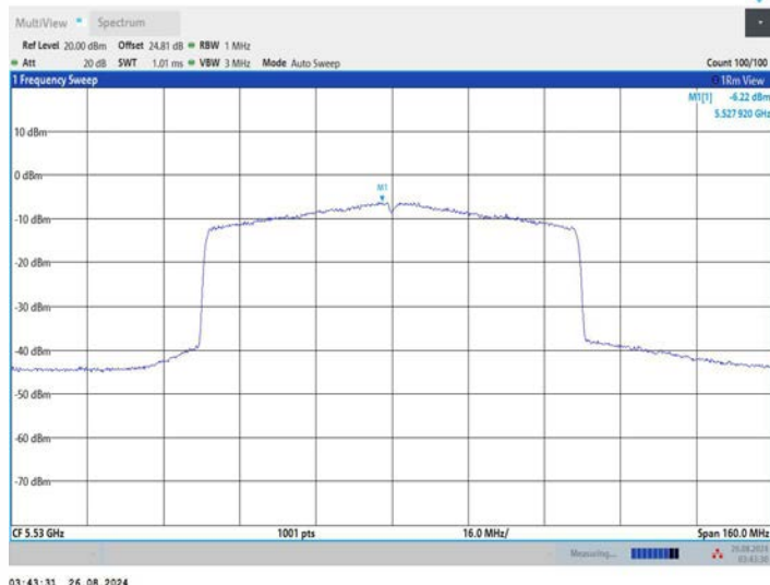
11AX80MIMO_Ant3_5530
