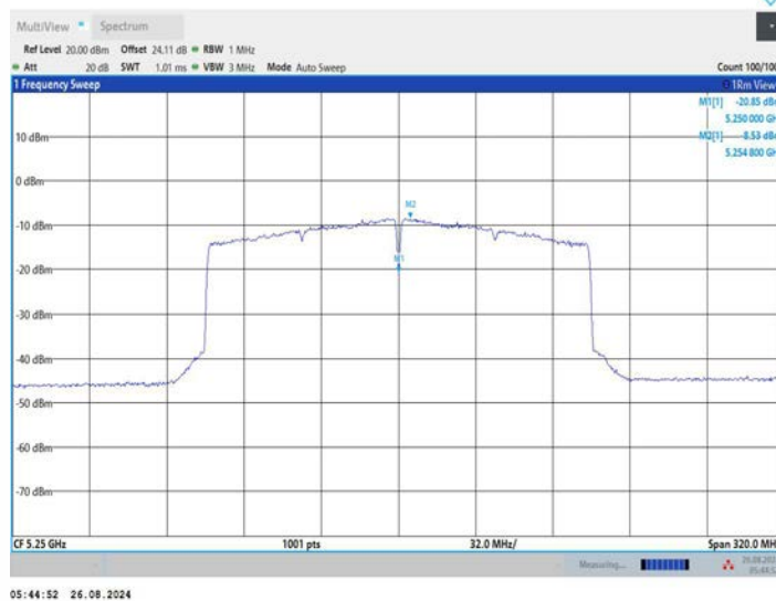
11AX160MIMO_Ant2_5250_UNII-2A
