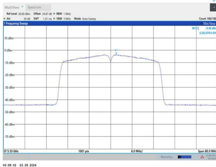
11AC40MIMO_Ant3_5550
