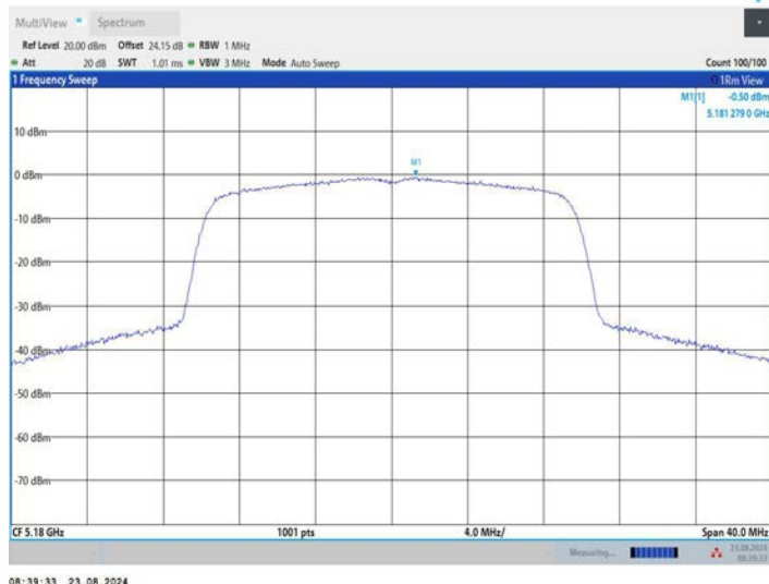
11AX20MIMO_Ant2_5180
