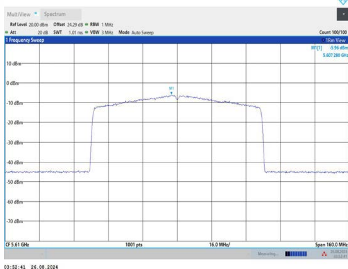
11AX80MIMO_Ant3_5610
