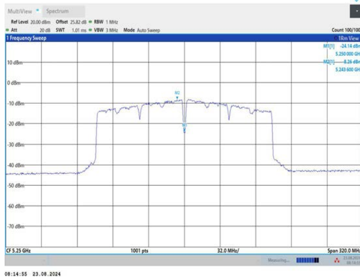
11AC160MIMO_Ant2_5250_UNII-1
