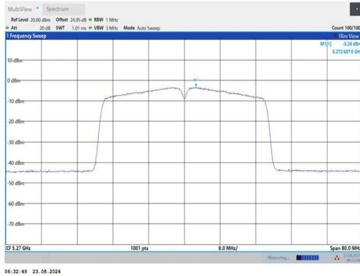
11AC40MIMO_Ant3_5270
