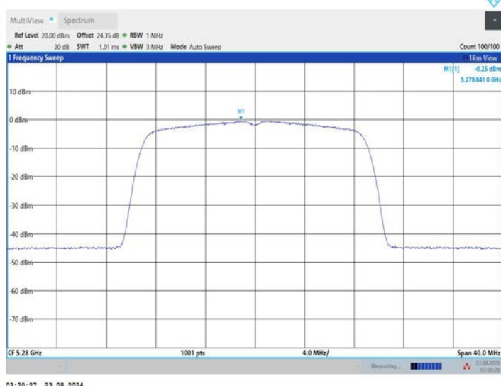
11AC20MIMO_Ant2_5280
