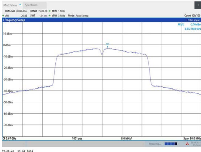
11AC40MIMO_Ant3_5670
