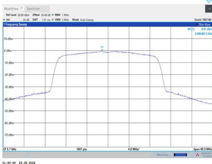
11AX20MIMO_Ant3_5700
