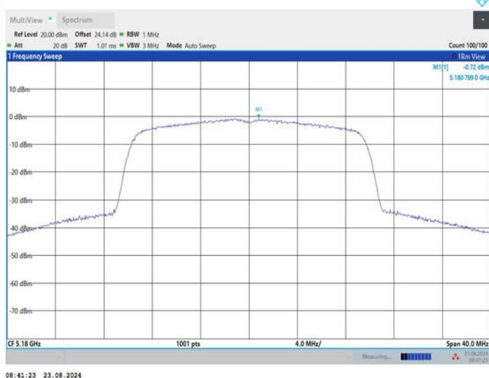
11AX20MIMO_Ant3_5180
