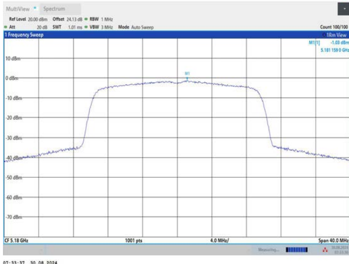
11BE20MIMO_Ant3_5180
