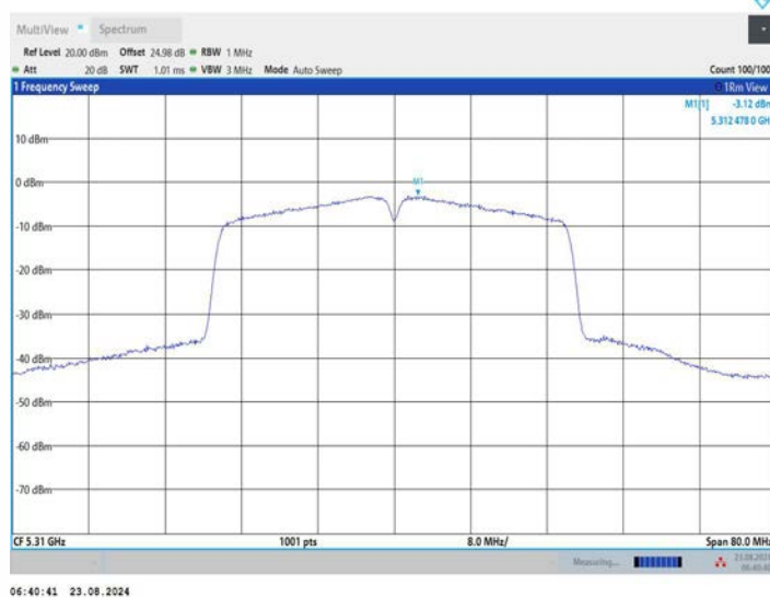
11AC40MIMO_Ant3_5310
