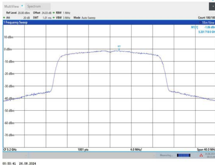
11AX20MIMO_Ant3_5200
