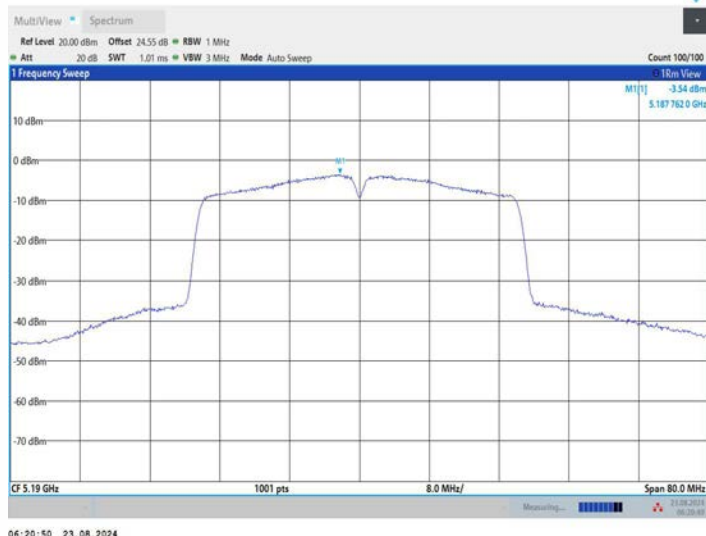
11AC40MIMO_Ant3_5190
