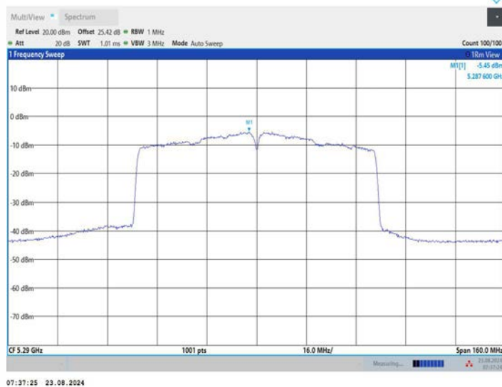
11AC80MIMO_Ant2_5290
