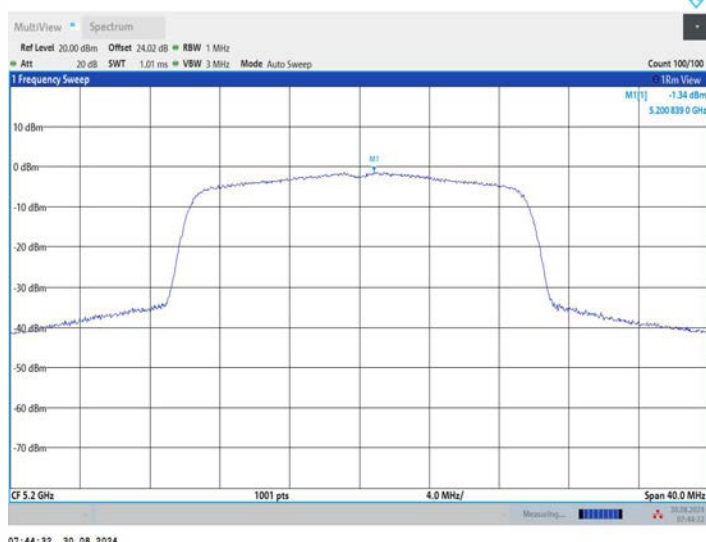
11BE20MIMO_Ant3_5200
