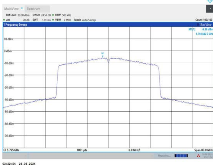
11AX40MIMO_Ant3_5795
