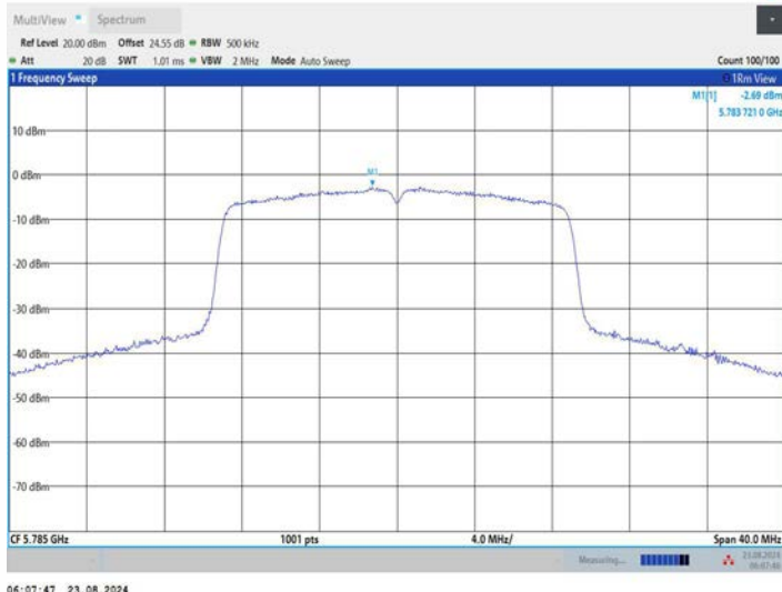
11AC20MIMO_Ant3_5785
