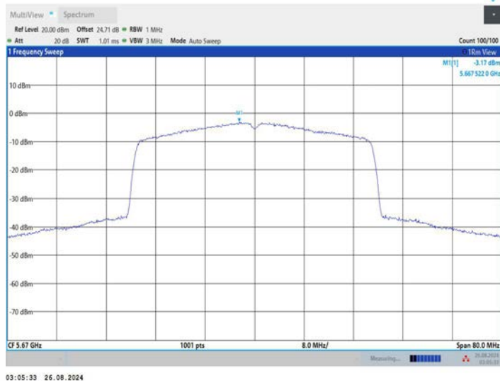
11AX40MIMO_Ant2_5670
