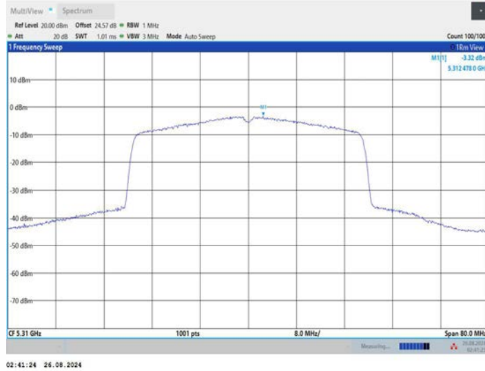
11AX40MIMO_Ant3_5310
