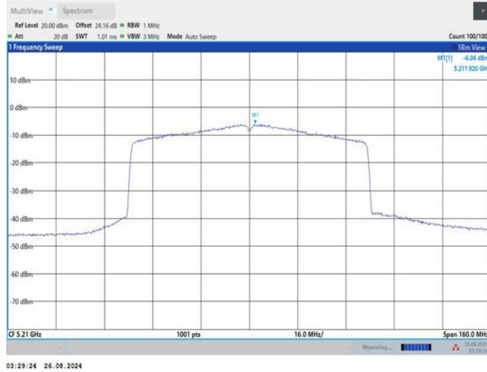
11AX80MIMO_Ant3_5210
