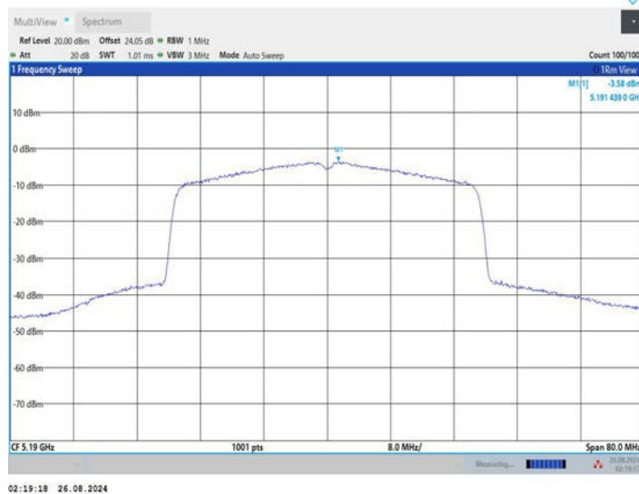
11AX40MIMO_Ant3_5190
