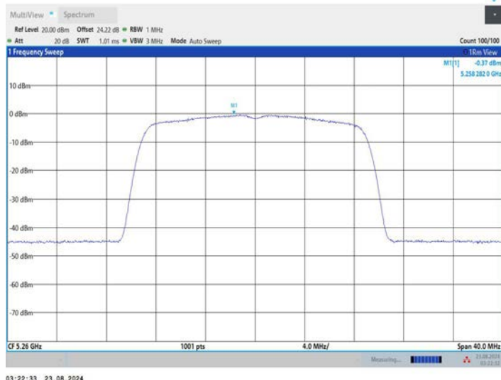
11AC20MIMO_Ant2_5260
