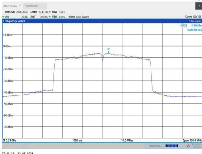
11AC80MIMO_Ant3_5290
