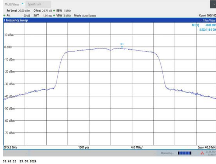
11AC20MIMO_Ant3_5500
