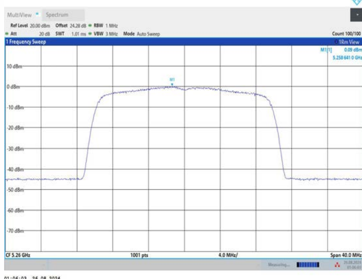
11AX20MIMO_Ant2_5260
