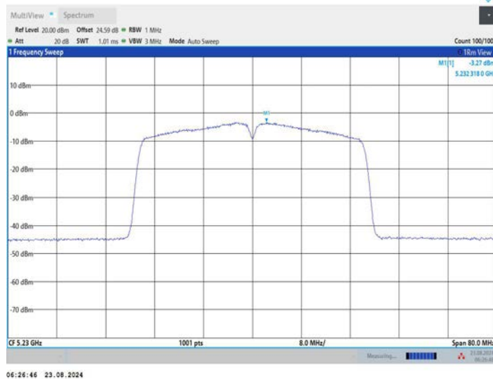
11AC40MIMO_Ant3_5230
