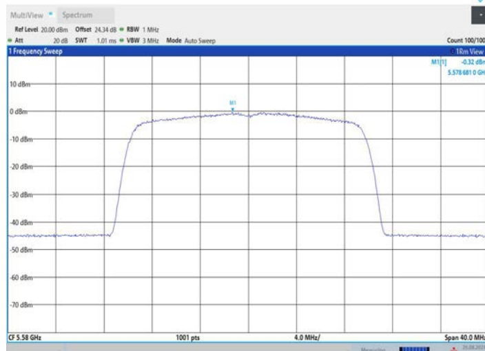
11AX20MIMO_Ant2_5580
