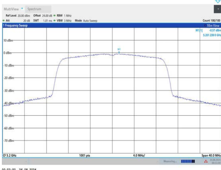
11AX20MIMO_Ant2_5200
