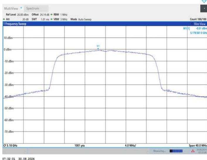
11BE20MIMO_Ant2_5180
