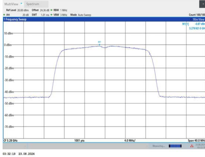
11AC20MIMO_Ant3_5280
