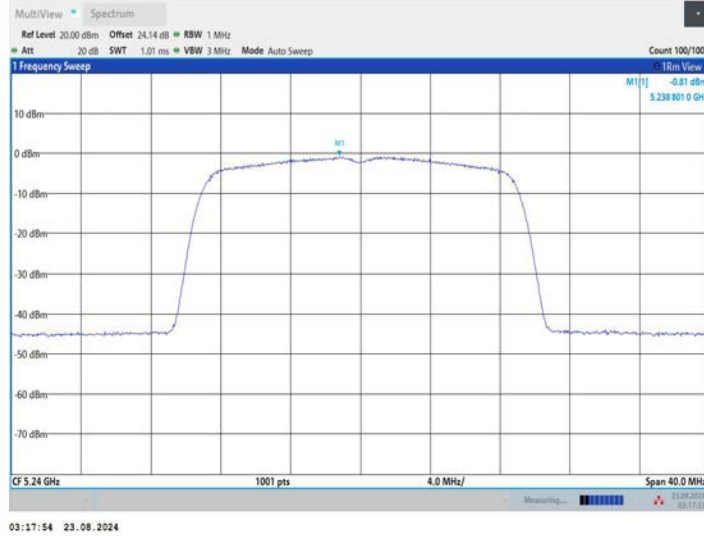
11AC20MIMO_Ant3_5240
