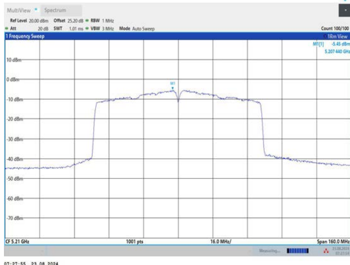
11AC80MIMO_Ant2_5210
