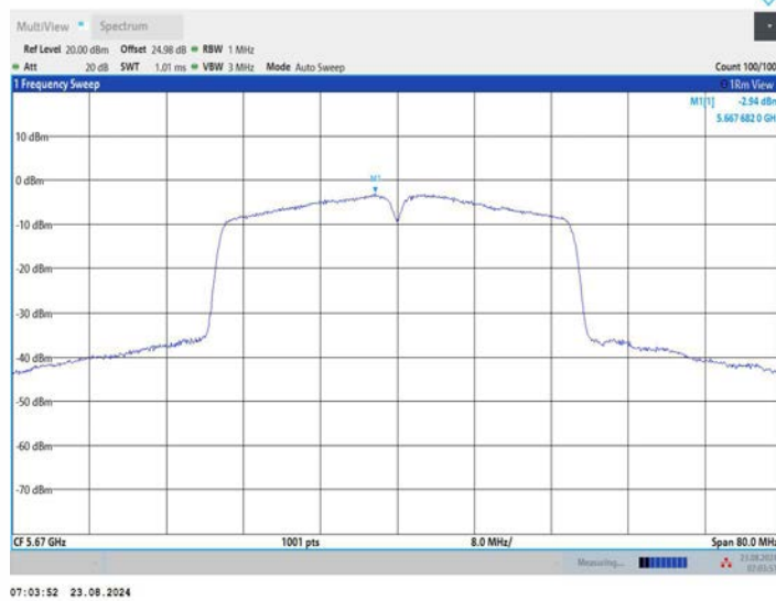
11AC40MIMO_Ant2_5670
