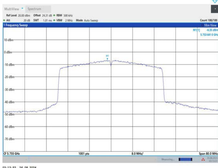
11AX40MIMO_Ant2_5755
