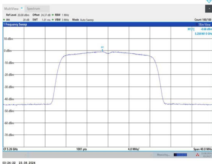
11AC20MIMO_Ant3_5260
