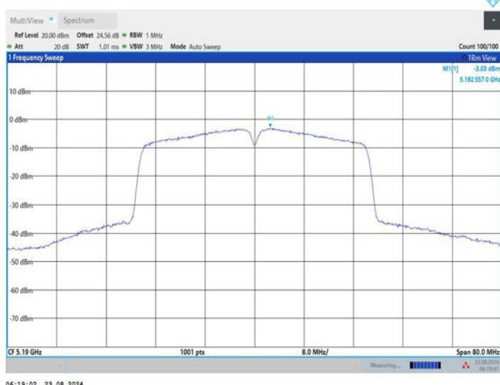
11AC40MIMO_Ant2_5190
