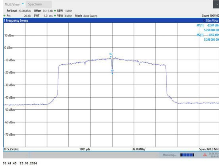
11AX160MIMO_Ant2_5250_UNII-1
