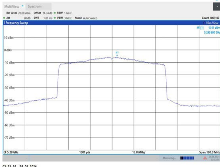
11AX80MIMO_Ant2_5290
