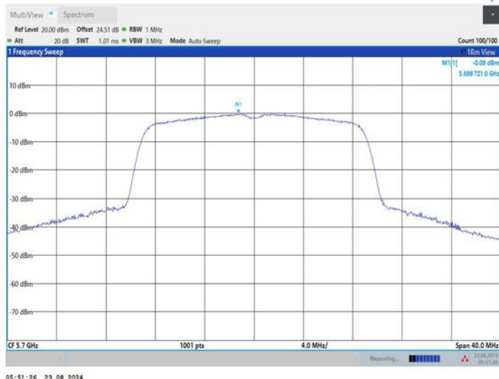
11AC20MIMO_Ant3_5700
