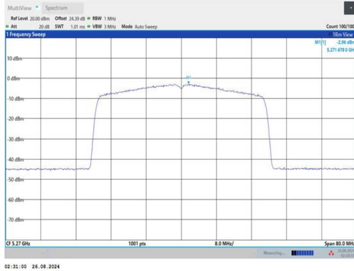
11AX40MIMO_Ant2_5270
