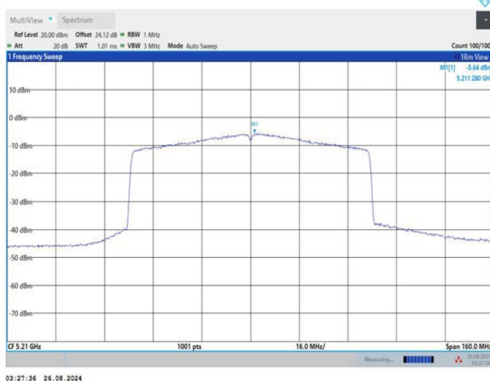
11AX80MIMO_Ant2_5210
