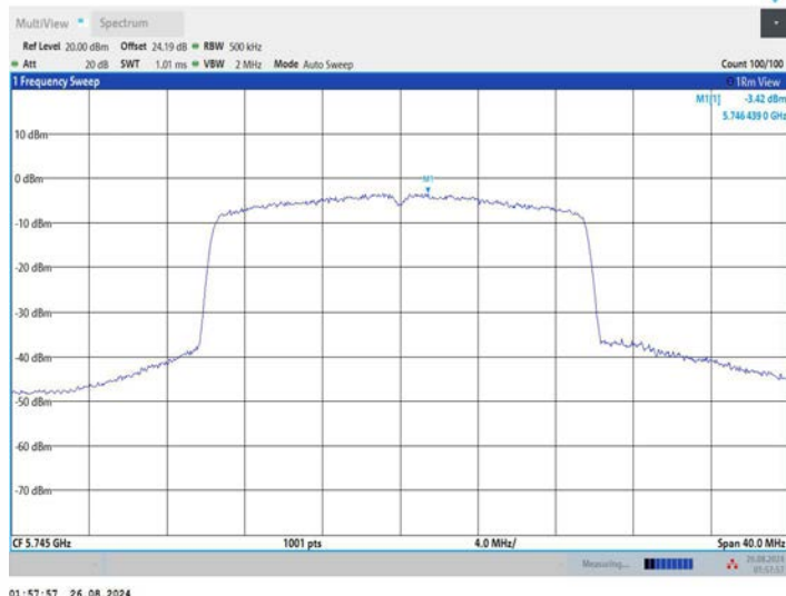
11AX20MIMO_Ant3_5745
