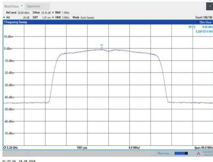
11AX20MIMO_Ant3_5260
