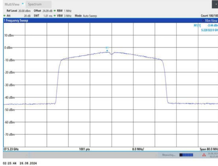
11AX40MIMO_Ant3_5230
