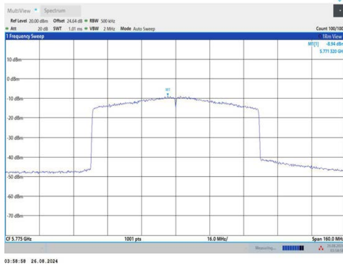
11AX80MIMO_Ant2_5775
