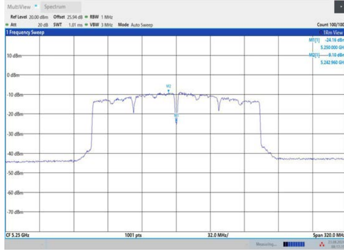
11AC160MIMO_Ant3_5250_UNII-1
