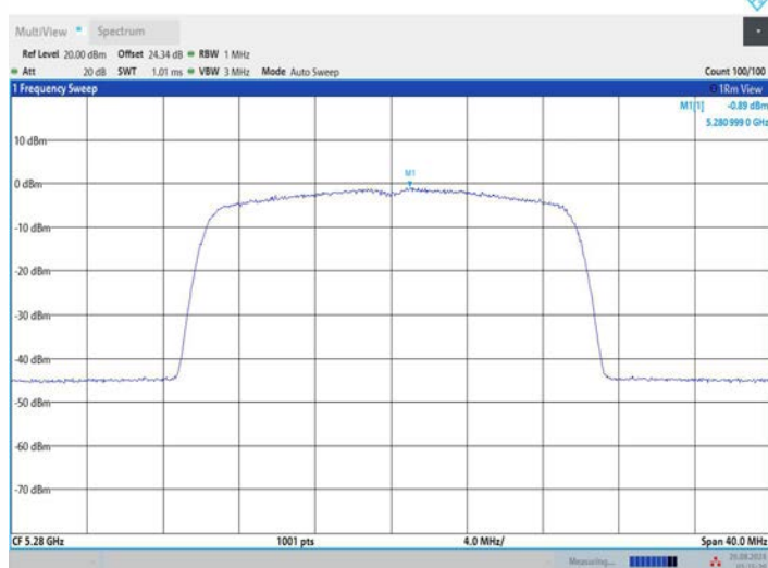
11AX20MIMO_Ant3_5280
