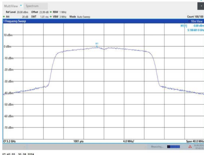
11BE20MIMO_Ant2_5200
