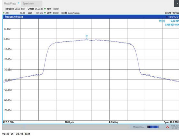
11AX20MIMO_Ant2_5500
