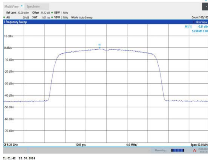
11AX20MIMO_Ant3_5240
