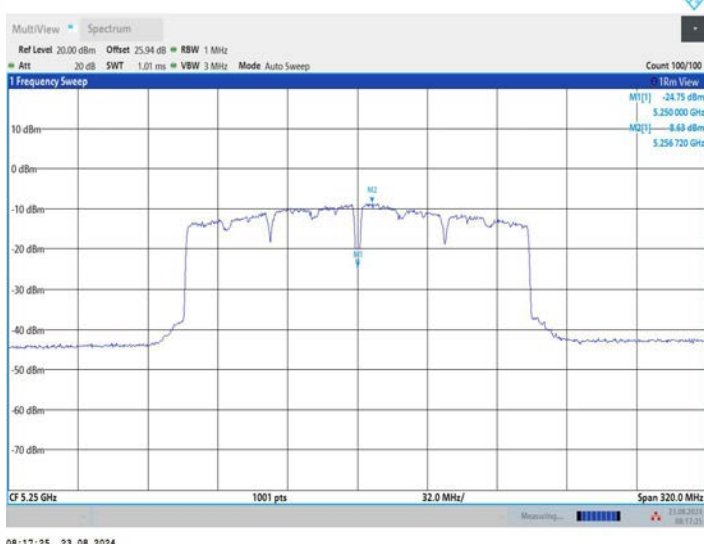
11AC160MIMO_Ant3_5250_UNII-2A
