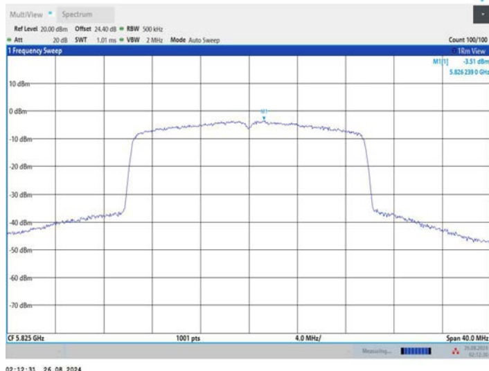
11AX20MIMO_Ant3_5825
