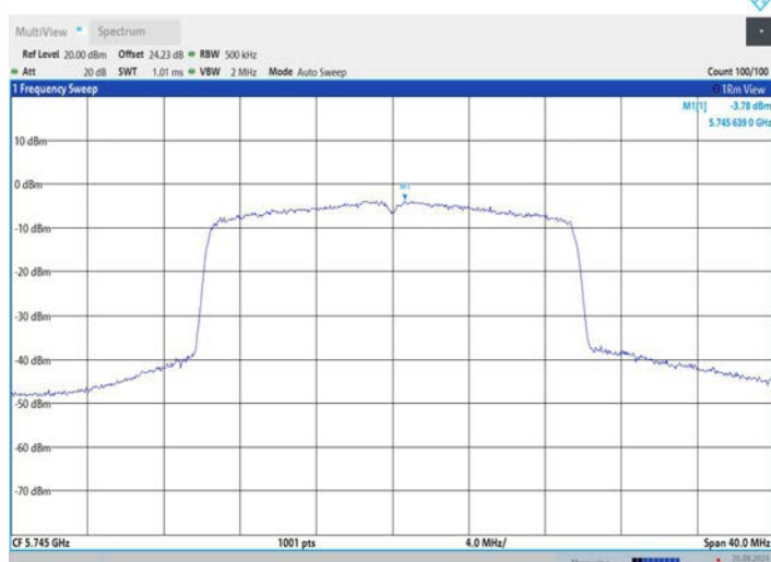
11AX20MIMO_Ant2_5745
