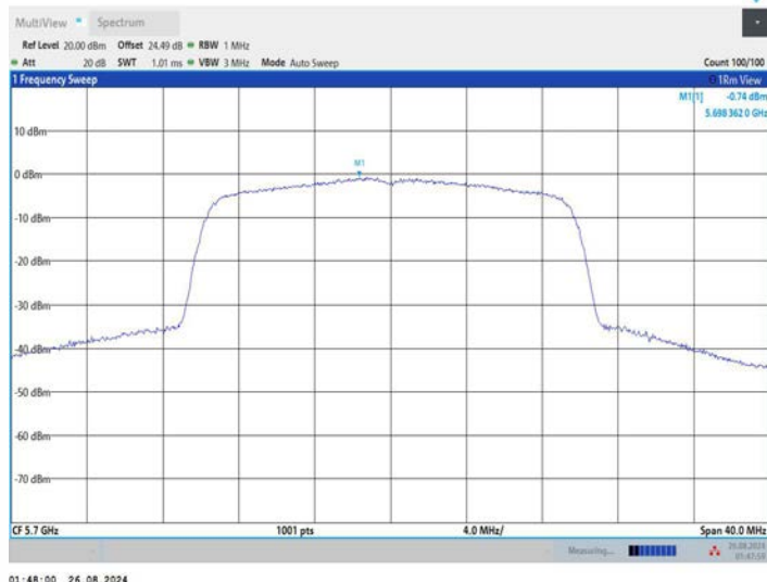
11AX20MIMO_Ant2_5700
