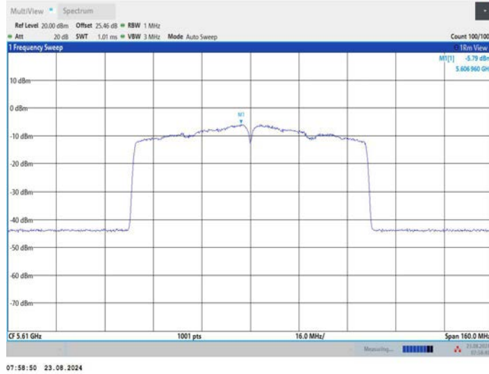
11AC80MIMO_Ant3_5610
