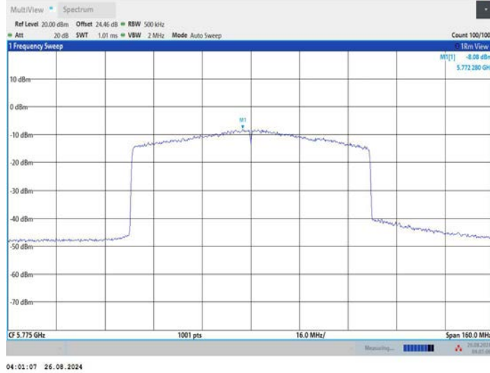
11AX80MIMO_Ant3_5775
