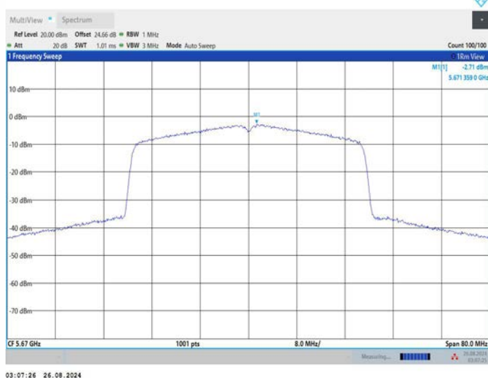
11AX40MIMO_Ant3_5670
