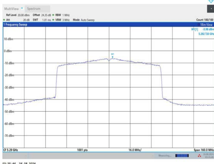
11AX80MIMO_Ant3_5290
