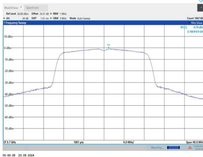
11AC20MIMO_Ant2_5700
