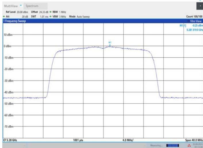
11AX20MIMO_Ant2_5280
