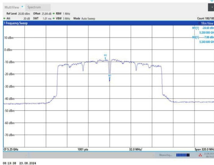
11AC160MIMO_Ant1_5250_UNII-2A
