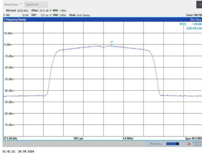
11AX20MIMO_Ant3_5580
