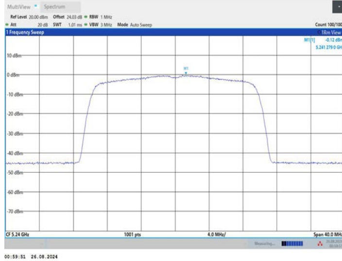
11AX20MIMO_Ant2_5240
