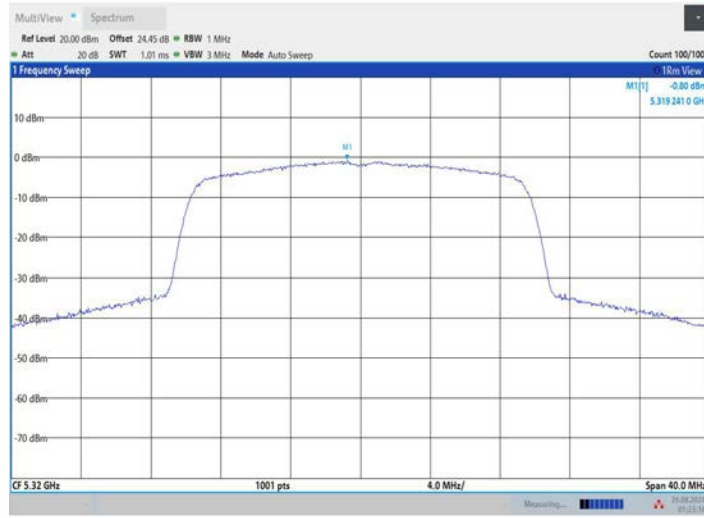
11AX20MIMO_Ant3_5320
