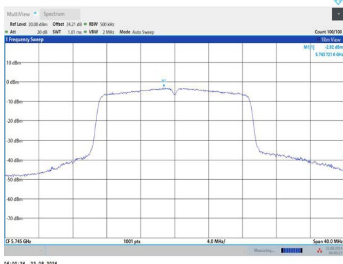
11AC20MIMO_Ant3_5745
