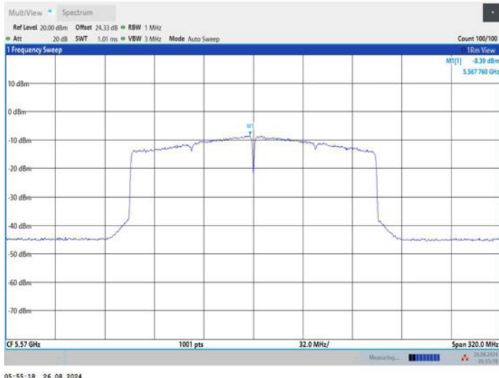
11AX160MIMO_Ant2_5570
