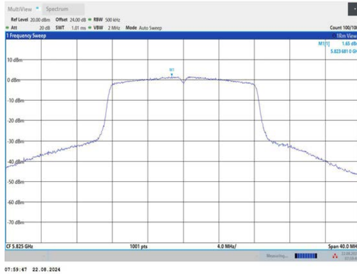
11A_Ant3_5825
