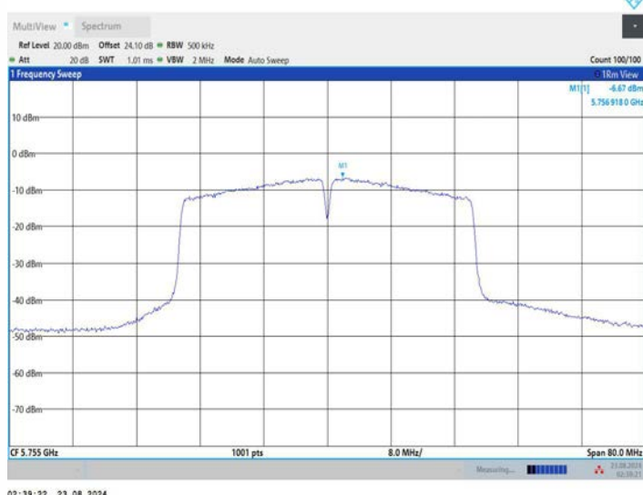
11N40MIMO_Ant2_5755
