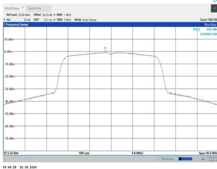
11N20MIMO_Ant2_5320
