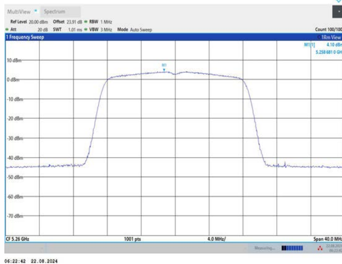
11A_Ant2_5260
