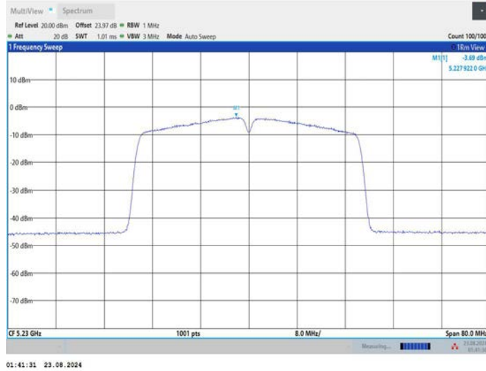
11N40MIMO_Ant3_5230
