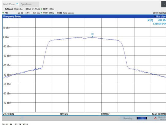
11N20MIMO_Ant1_5200
