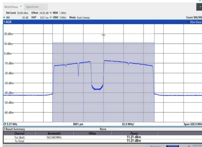
11BE160MIMO_Ant2_5570_996+484+242_OFDMA_5
