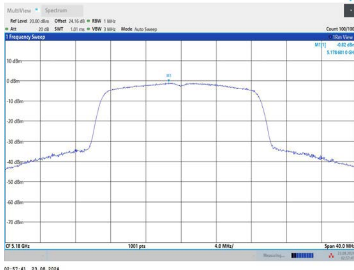
11AC20MIMO_Ant3_5180
