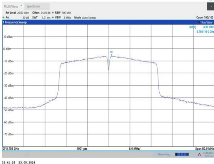
11N40MIMO_Ant3_5755
