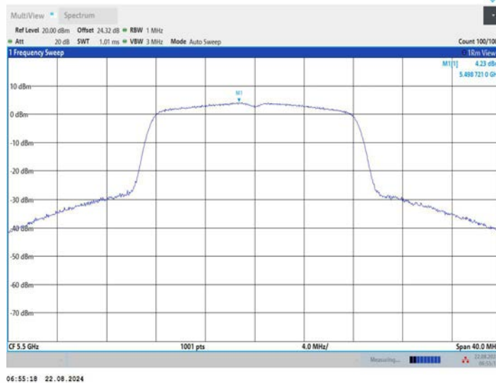
11A_Ant3_5500
