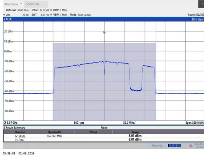
11BE160MIMO_Ant3 5570 996+484+242 OFDMA 7
