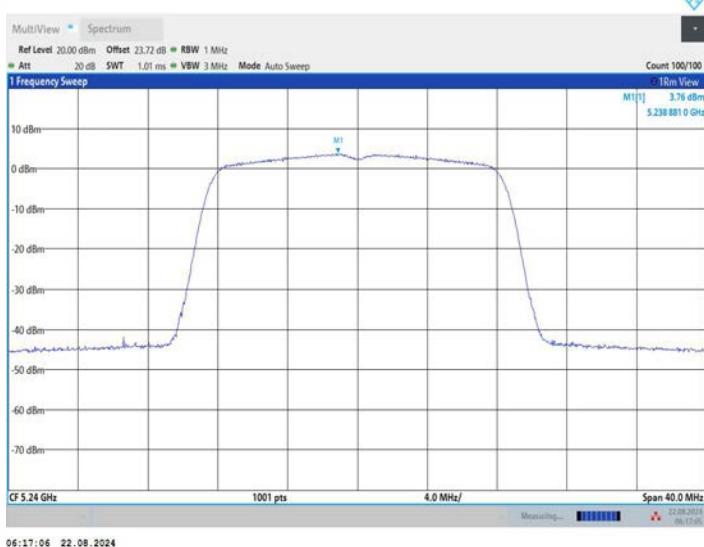
11A_Ant3_5240
