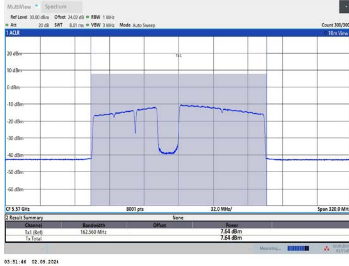
11BE160MIMO_Ant3_5570_996+484+242_OFDMA_4
