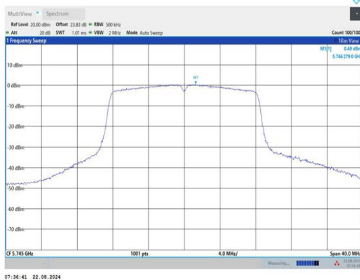
11A_Ant2_5745
