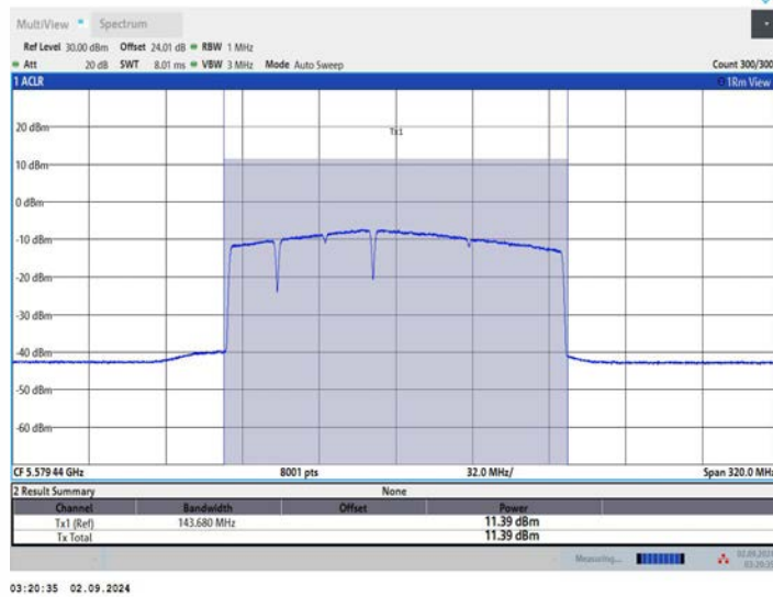
11BE160MIMO_Ant2_5570_996+484+242_OFDMA_2
