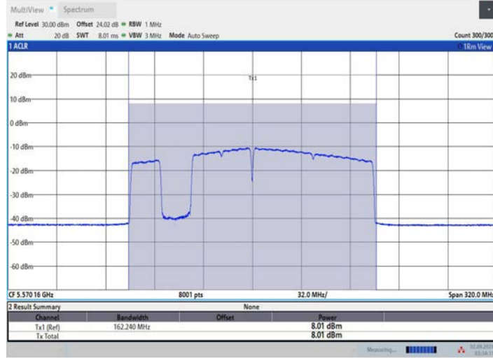
11BE160MIMO_Ant3 5570_996+484+242_OFDMA 2
