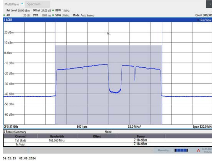
11BE160MIMO_Ant2_5570_996+484+242_OFDMA_5
