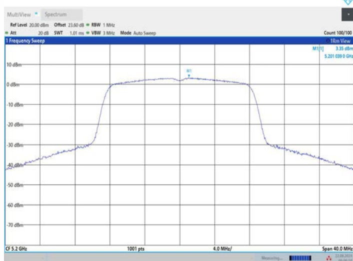
11A_Ant2_5200
