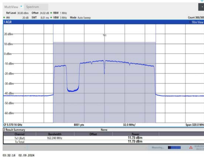
11BE160MIMO_Ant3 5570_996+484+242_OFDMA 3
