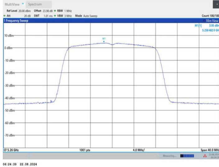
11A_Ant3_5260
