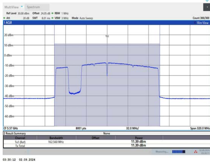
11BE160MIMO_Ant2_5570_996+484+242_OFDMA_3
