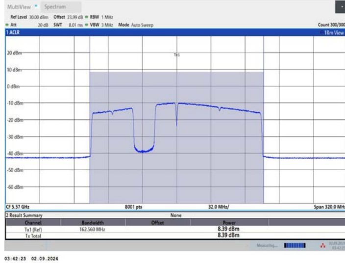
11BE160MIMO_Ant1 5570 996+484+242 OFDMA 3
