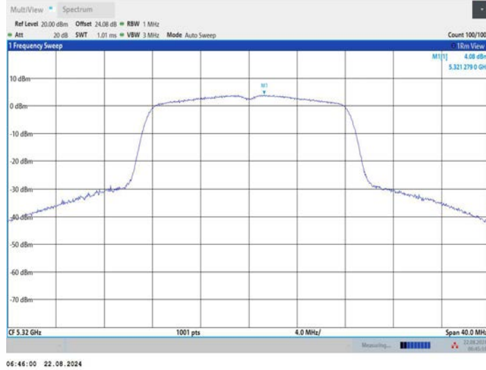
11A_Ant3_5320
