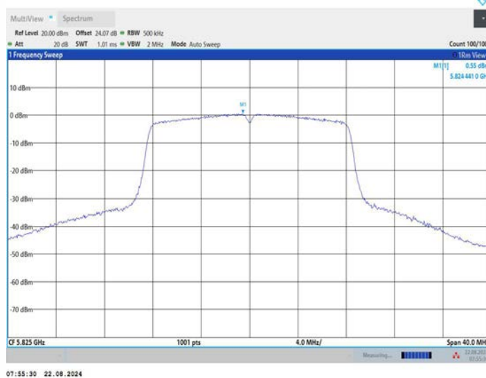
11A_Ant2_5825
