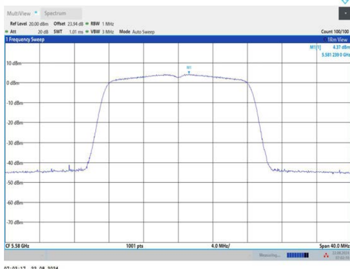
11A_Ant2_5580
