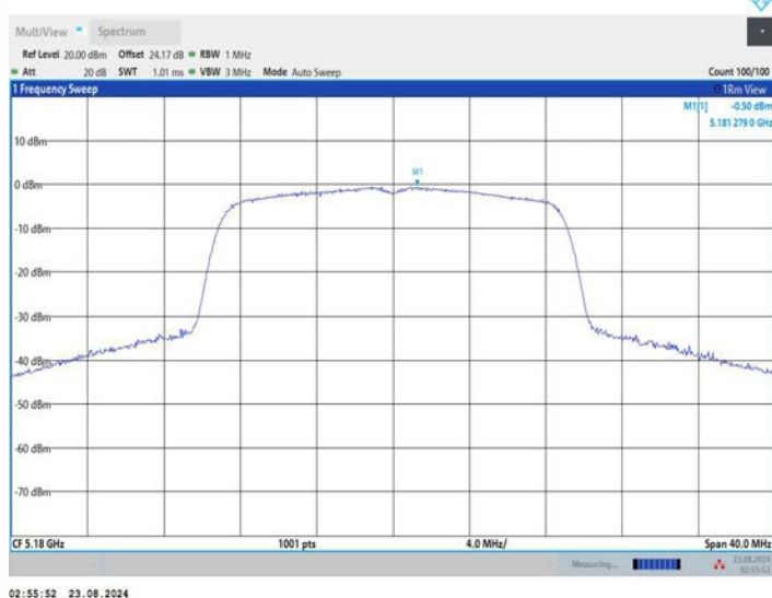
11AC20MIMO_Ant2_5180
