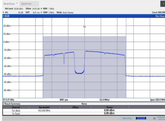
11BE160MIMO_Ant2_5570_996+484+242_OFDMA_4
