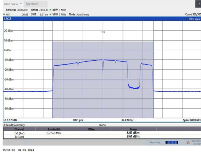
11BE160MIMO_Ant1 5570_996+484+242_OFDMA 7
