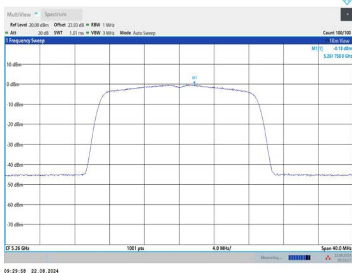
11N20MIMO_Ant2_5260
