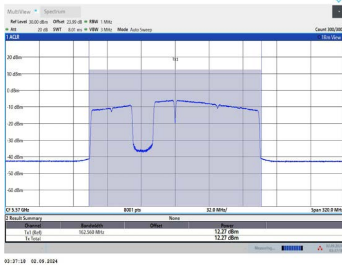
11BE160MIMO_Ant1 5570 996+484+242 OFDMA 4
