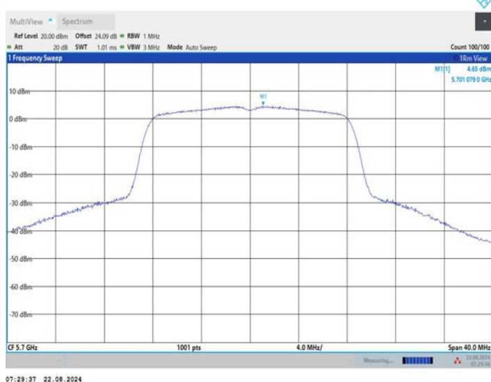
11A_Ant3_5700
