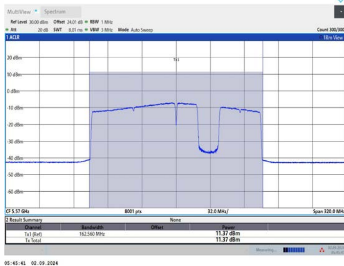
11BE160MIMO_Ant2_5570_996+484+242_OFDMA_7
