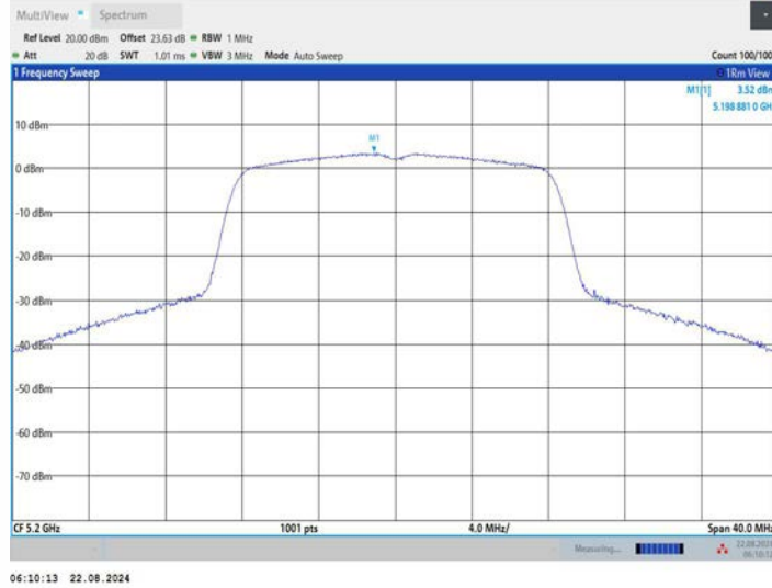
11A_Ant3_5200
