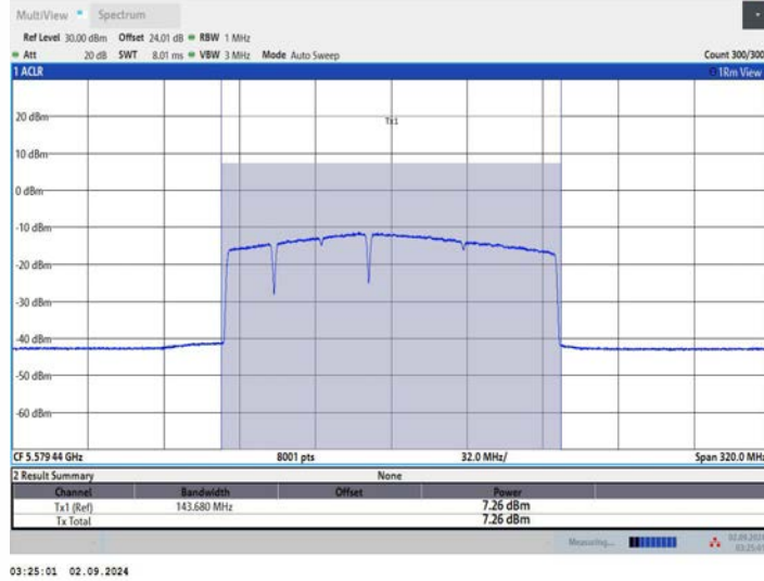
11BE160MIMO_Ant2_5570_996+484+242_OFDMA_1
