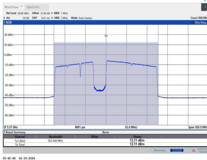
11BE160MIMO_Ant1 5570 996+484+242 OFDMA 5
