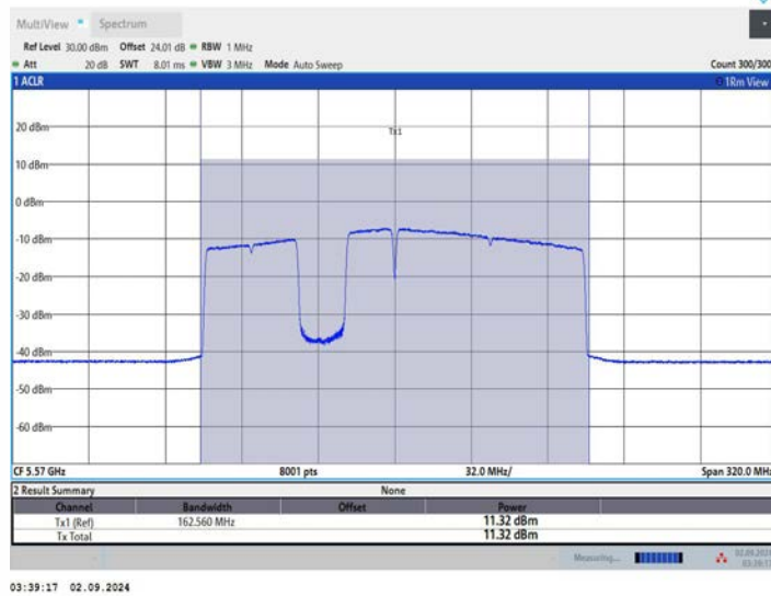
11BE160MIMO_Ant2_5570_996+484+242_OFDMA_4
