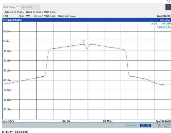
11N40MIMO_Ant2_5310
