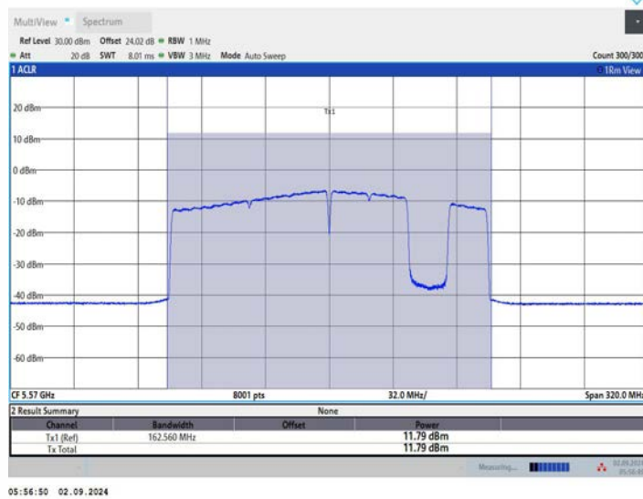
11BE160MIMO_Ant3 5570 996+484+242 OFDMA 8
