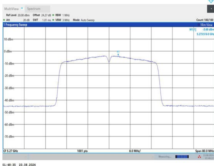
11N40MIMO_Ant3_5270
