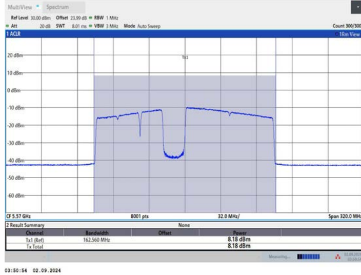
11BE160MIMO_Ant1 5570 996+484+242 OFDMA 4
