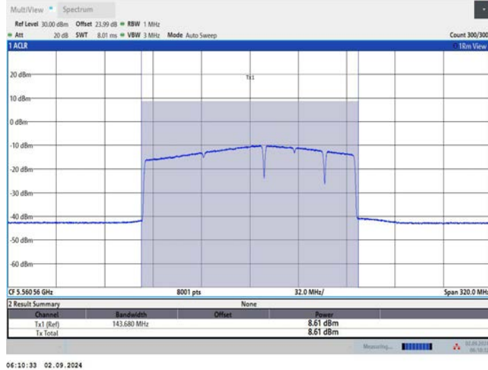
11BE160MIMO_Ant1 5570 996+484+242 OFDMA 8
