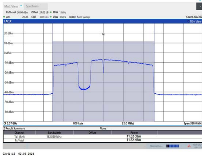
11BE160MIMO_Ant3_5570_996+484+242_OFDMA_4
