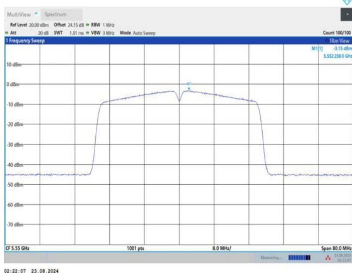
11N40MIMO_Ant2_5550
