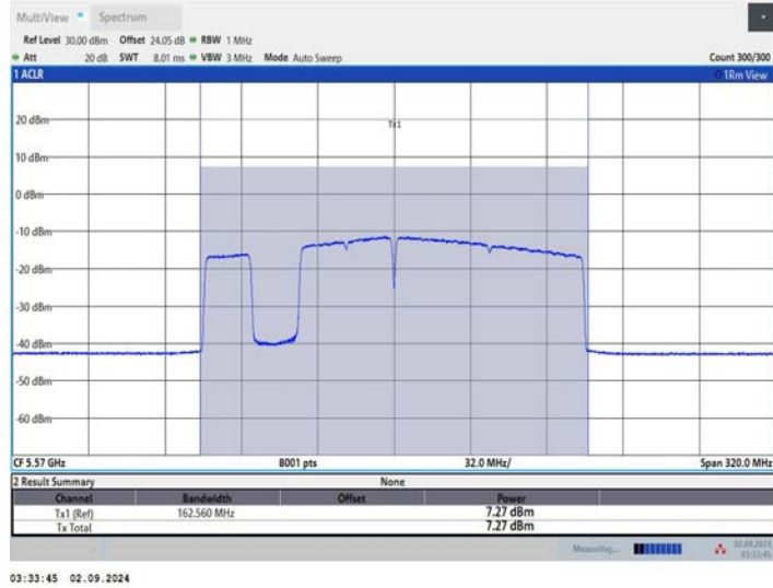
11BE160MIMO_Ant2_5570_996+484+242_OFDMA_2
