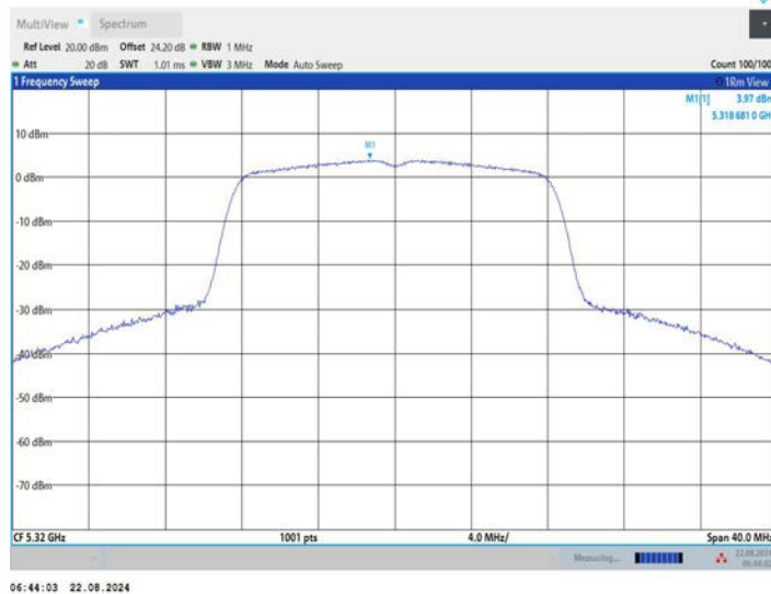
11A_Ant2_5320
