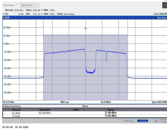
11BE160MIMO_Ant2_5570_996+484+242_OFDMA_6
