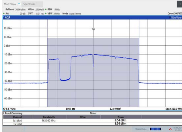
11BE160MIMO_Ant1 5570 996+484+242 OFDMA 2
