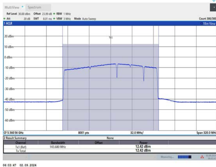
11BE160MIMO_Ant2 5570 996+484 OFDMA 1
