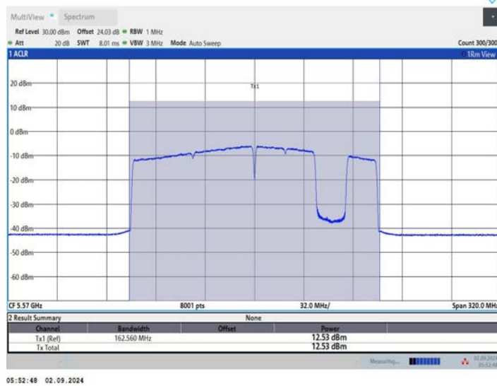
11BE160MIMO_Ant1 5570_996+484+242_OFDMA 8
