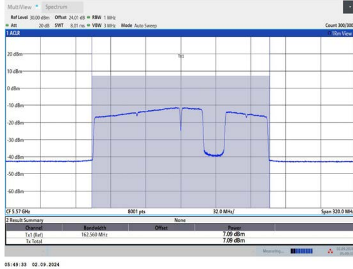
11BE160MIMO_Ant2_5570_996+484+242_OFDMA_6
