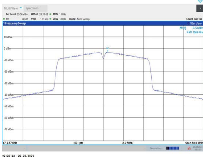
11N40MIMO_Ant3_5670
