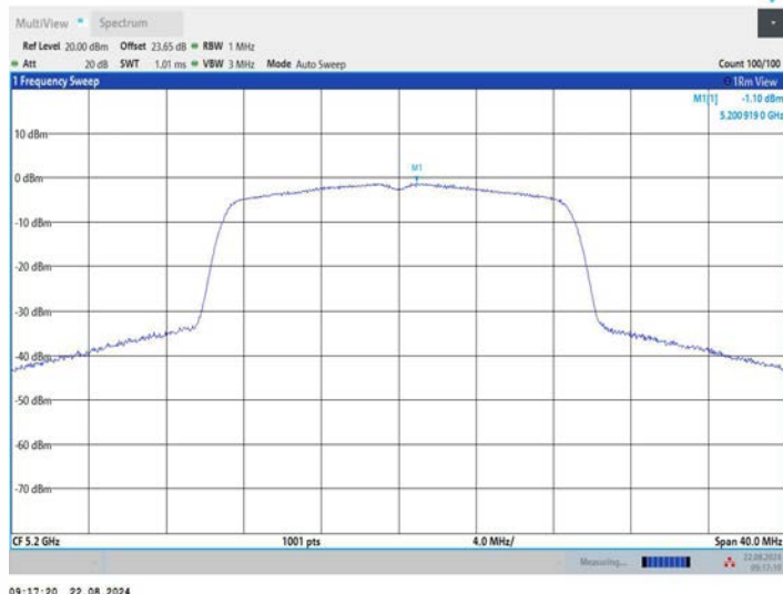
11N20MIMO_Ant3_5200
