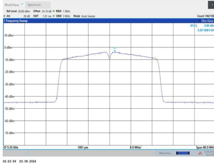
11N40MIMO_Ant3_5550
