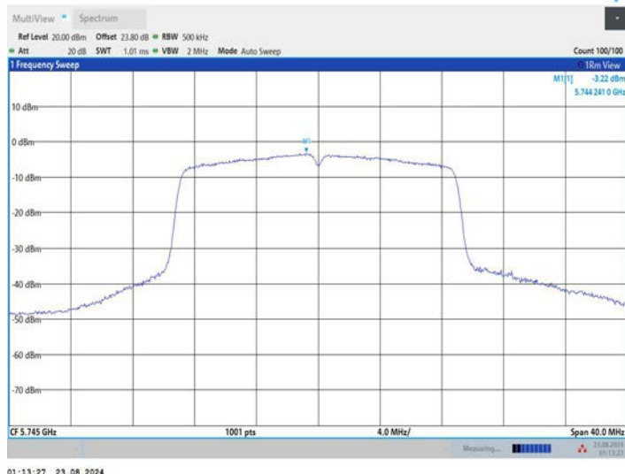
11N20MIMO_Ant3_5745
