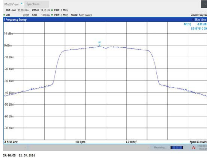
11N20MIMO_Ant3_5320
