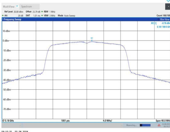
11N20MIMO_Ant3_5180
