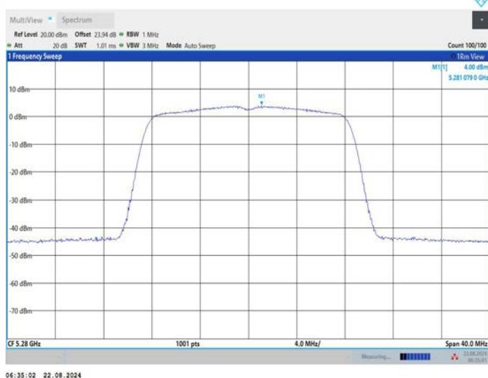
11A_Ant3_5280
