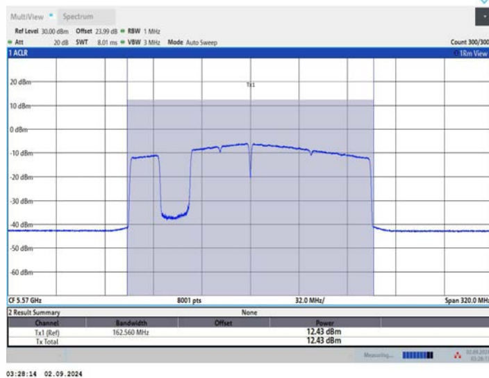
11BE160MIMO_Ant1 5570 996+484+242 OFDMA 3
