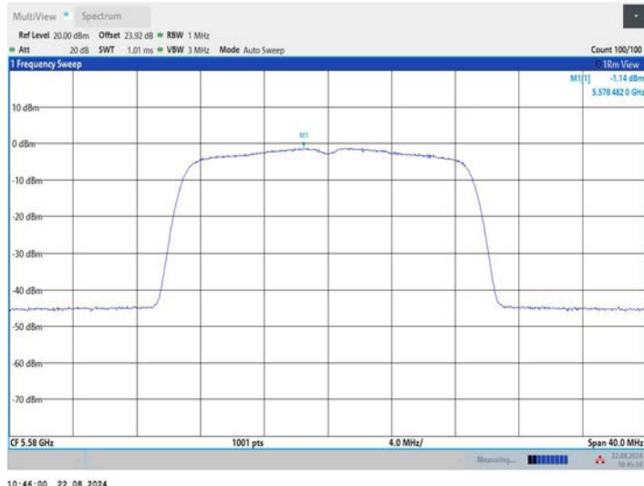
11N20MIMO_Ant3_5580
