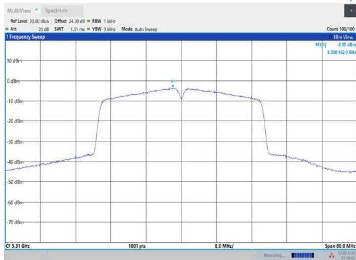
11N40MIMO_Ant3_5310
