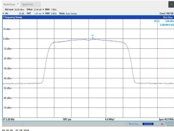
11N20MIMO_Ant2_5280
