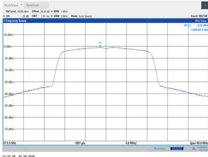
11N20MIMO_Ant2_5500
