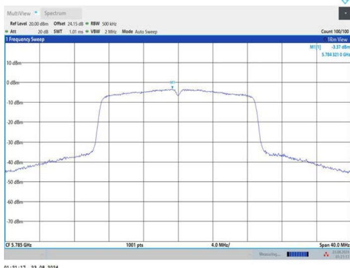
11N20MIMO_Ant3_5785
