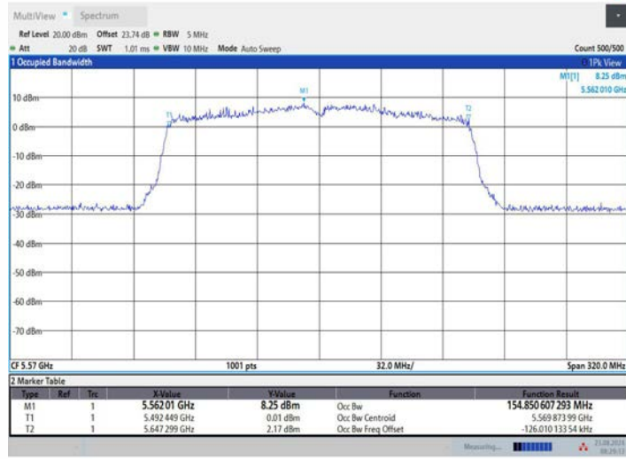
11AC160MIMO_Ant2_5570
