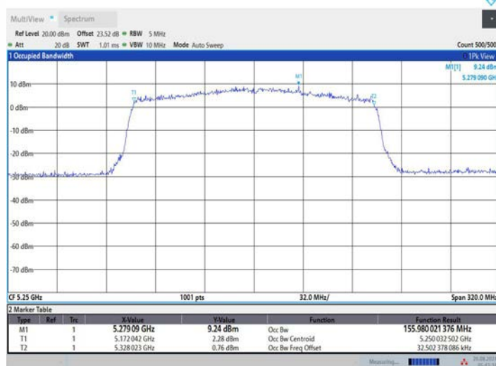
11AX160MIMO_Ant2_5250
