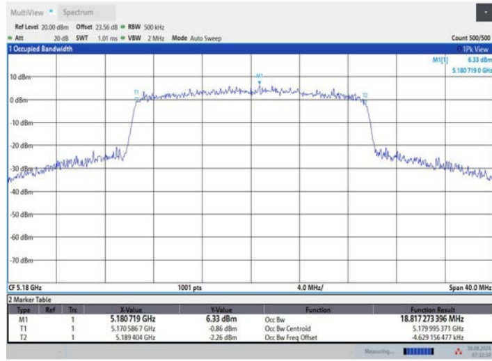
11BE20MIMO_Ant3_5180
