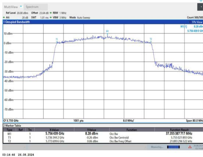
11AX40MIMO_Ant3_5755
