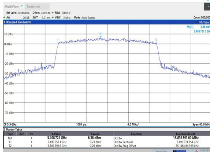
11AX20MIMO_Ant2_5500
