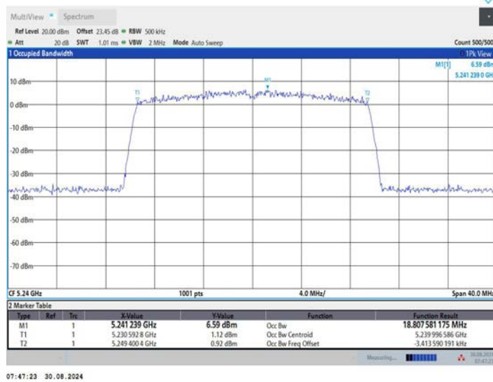
11BE20MIMO_Ant2_5240
