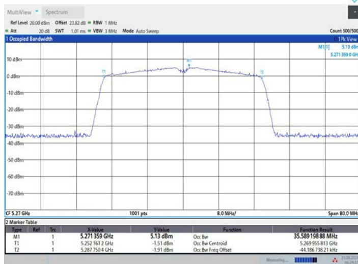
11AC40MIMO_Ant2_5270
