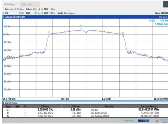
11AC40MIMO_Ant3_5795
