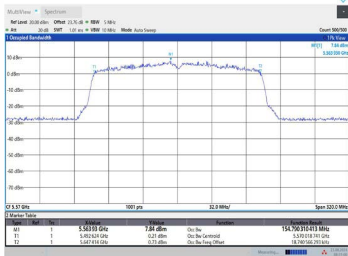
11AC160MIMO_Ant3_5570
