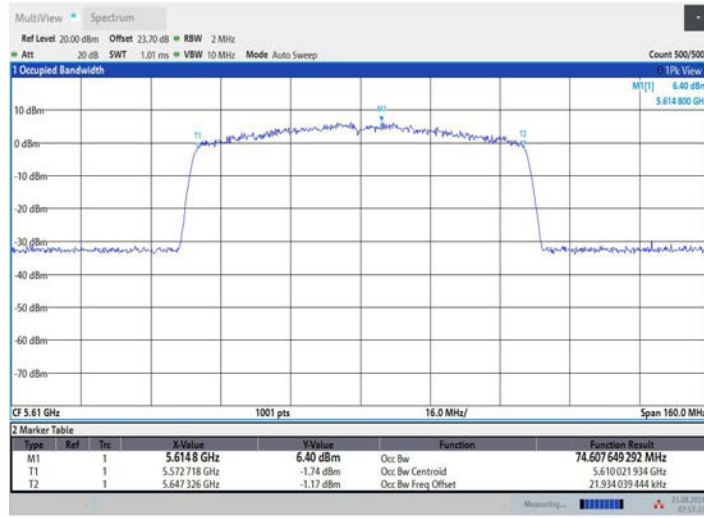
11AC80MIMO_Ant3_5610
