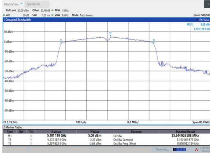
11AC40MIMO_Ant3_5190
