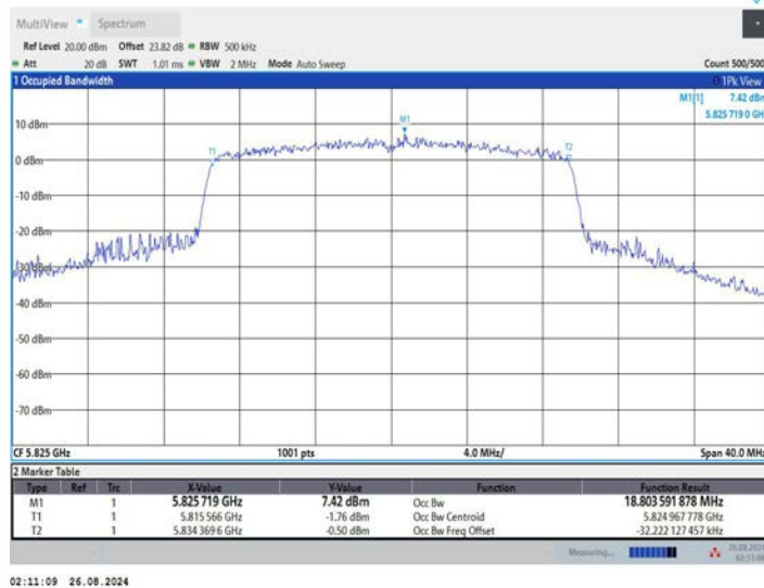
11AX20MIMO_Ant3_5825
