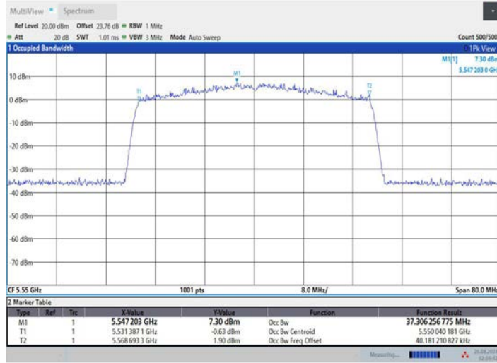
11AX40MIMO_Ant2_5550
