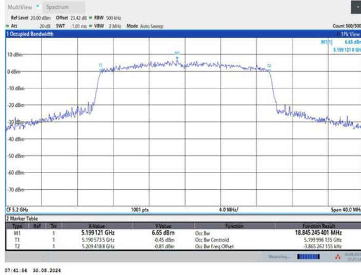
11BE20MIMO_Ant2_5200
