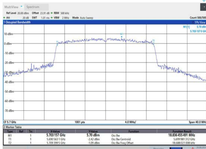
11AX20MIMO_Ant2_5700
