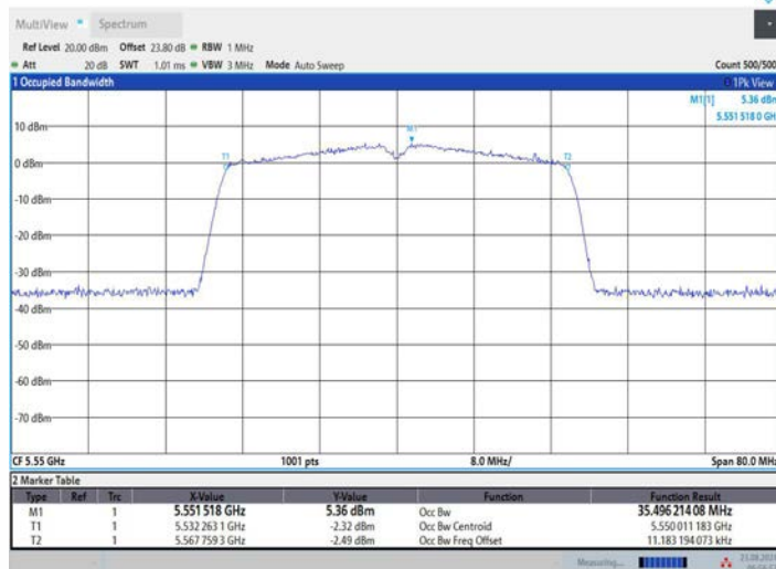
11AC40MIMO_Ant3_5550
