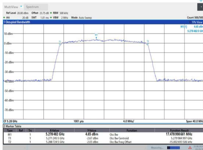
11AC20MIMO_Ant2_5280
