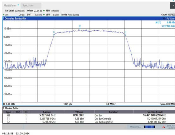
11A_Ant3_5240
