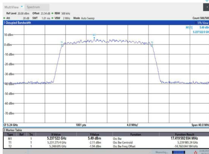
11N20MIMO_Ant3_5240
