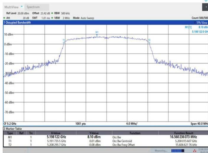
11A_Ant2_5200
