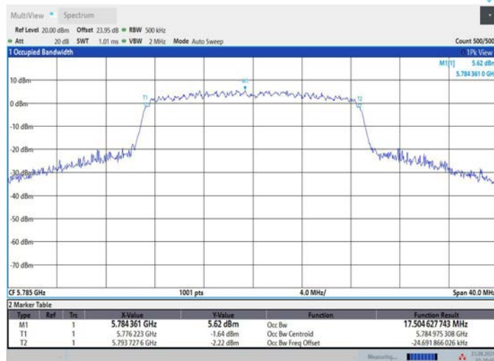
11N20MIMO_Ant3_5785
