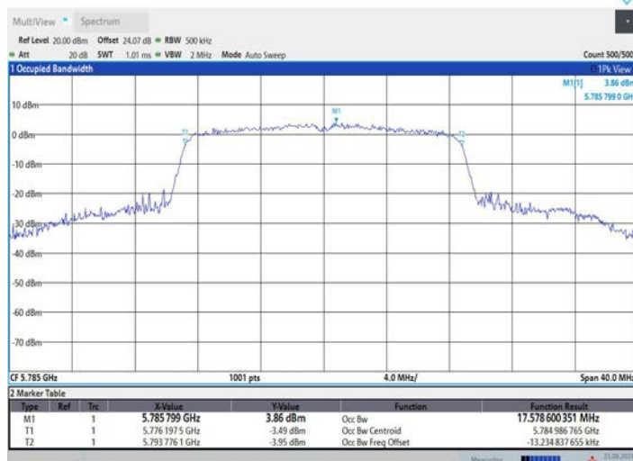
11AC20MIMO_Ant2_5785
