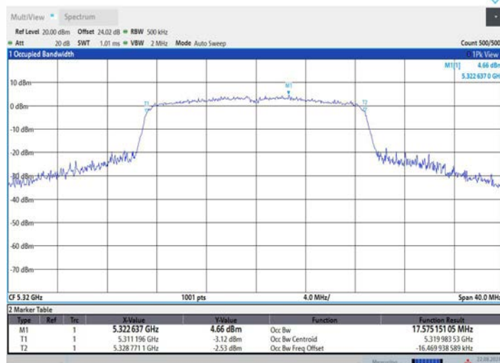
11N20MIMO_Ant2_5320
