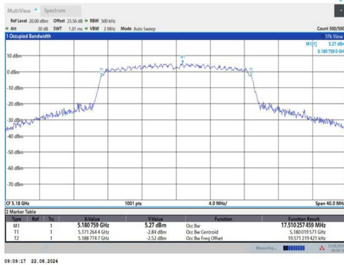
11N20MIMO_Ant3_5180
