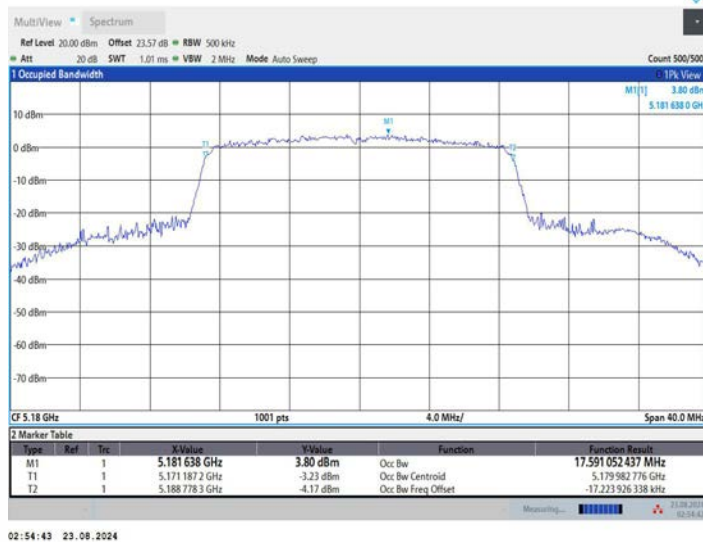
11AC20MIMO_Ant2_5180
