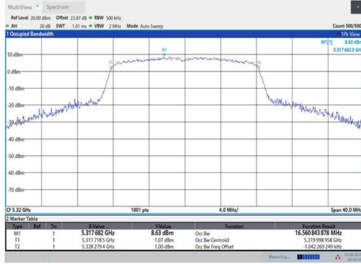
11A_Ant3_5320
