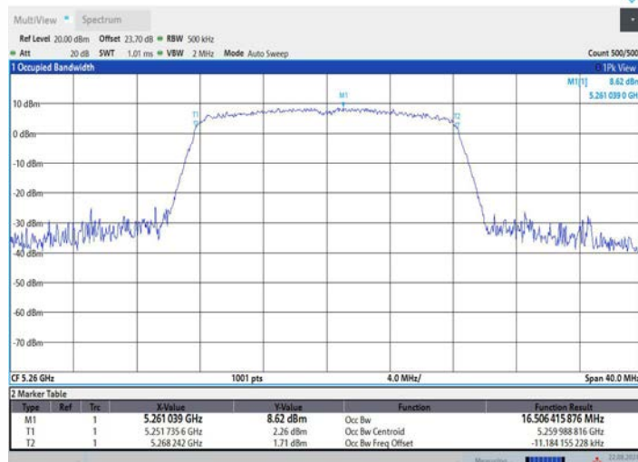
11A_Ant2_5260
