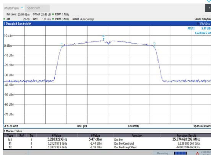
11N40MIMO_Ant2_5230
