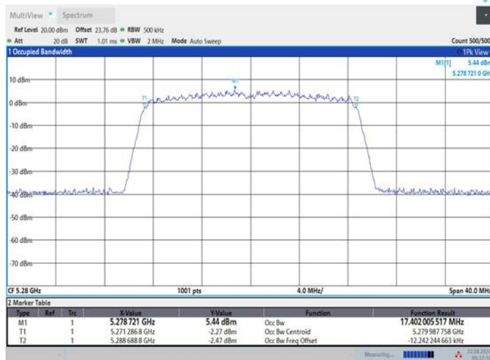
11N20MIMO_Ant3_5280
