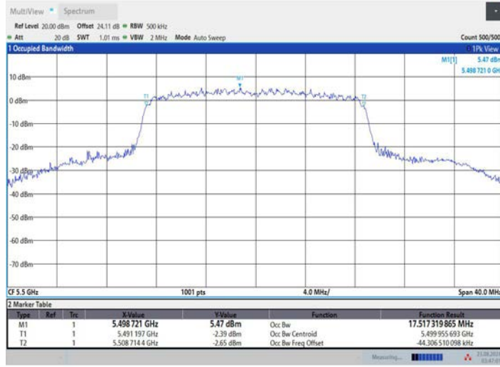
11AC20MIMO_Ant3_5500
