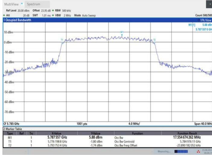
11AC20MIMO_Ant3_5785
