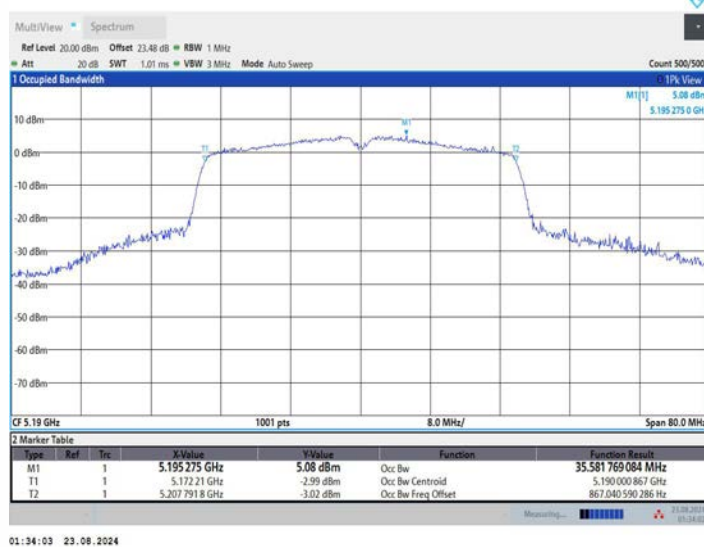
11N40MIMO_Ant3_5190
