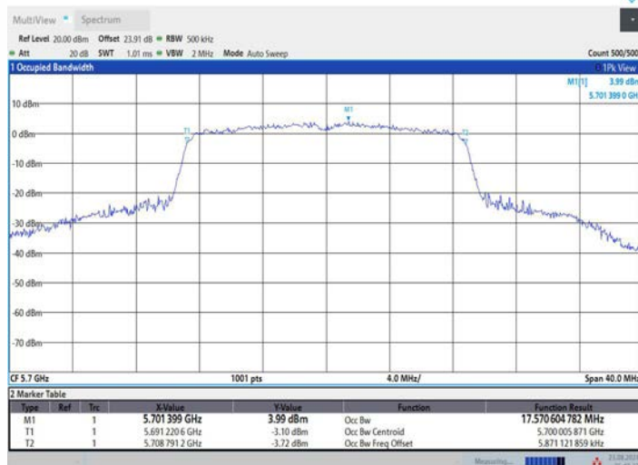
11AC20MIMO_Ant2_5700
