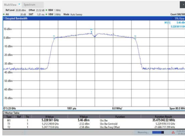
11N40MIMO_Ant3_5230
