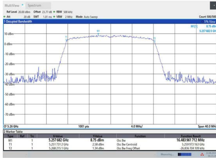
11A_Ant3_5260
