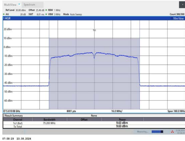
11AC80MIMO_Ant3_5610
