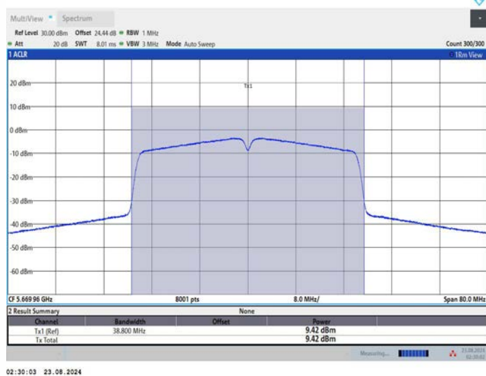
11N40MIMO_Ant2_5670
