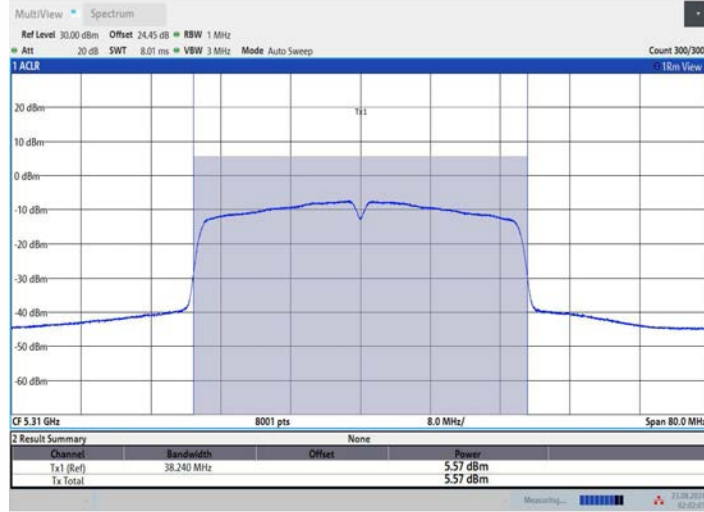
11N40MIMO_Ant3_5310
