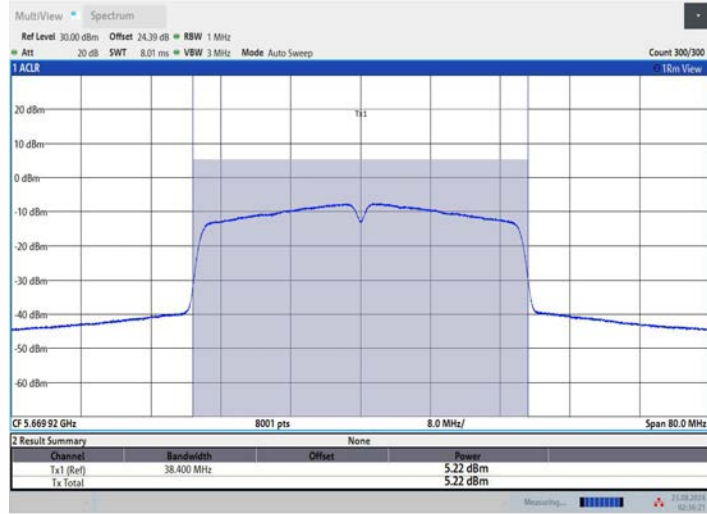
11N40MIMO_Ant2_5670
