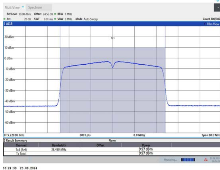
11AC40MIMO_Ant2_5230
