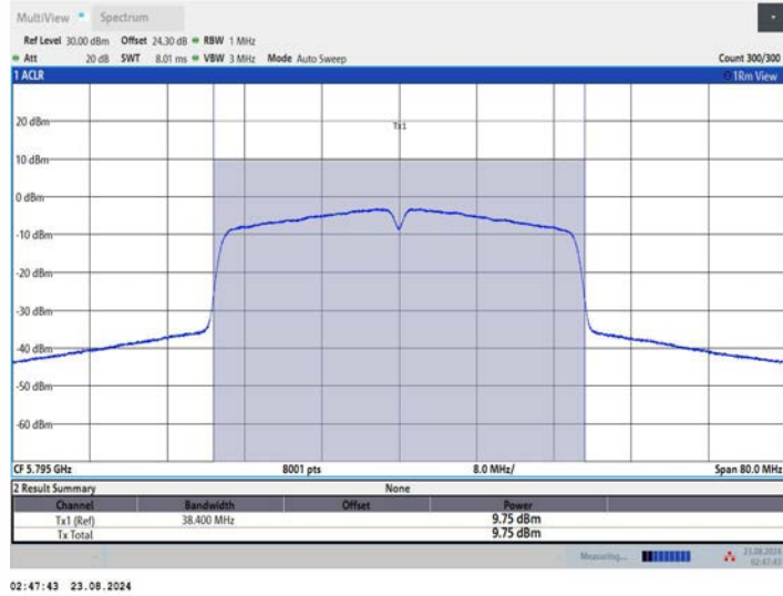
11N40MIMO_Ant3_5795
