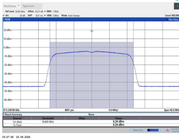
11AC20MIMO_Ant3_5260
