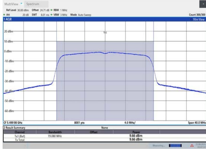
11AC20MIMO_Ant3_5500
