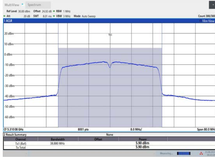
11AC40MIMO_Ant1_5310
