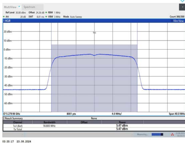
11AC20MIMO_Ant2_5280
