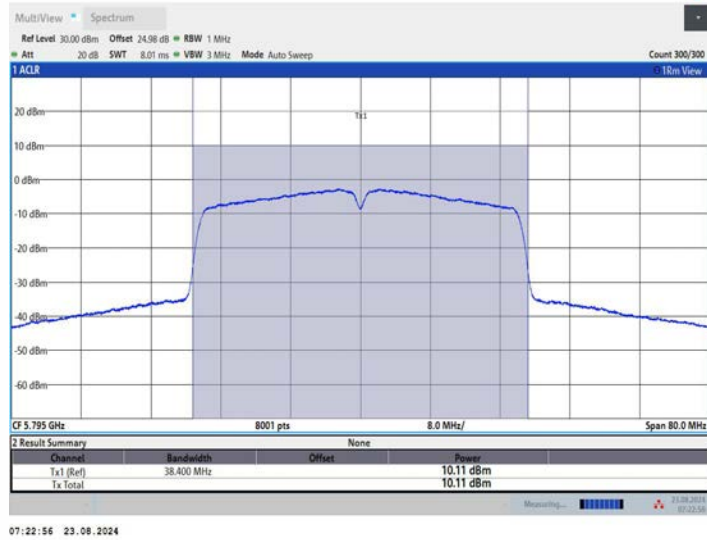
11AC40MIMO_Ant3_5795
