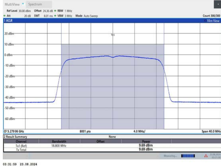
11AC20MIMO_Ant3_5280
