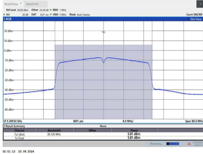
11N40MIMO_Ant1_5310
