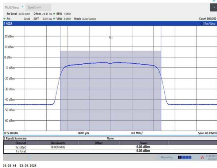
11AC20MIMO_Ant3_5280
