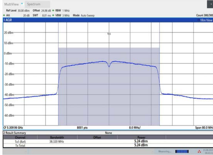
11AC40MIMO_Ant2_5310
