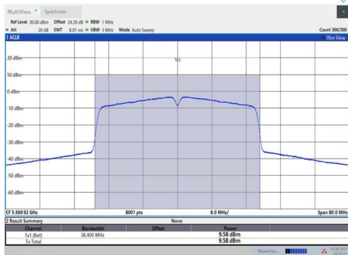
11N40MIMO_Ant3_5670
