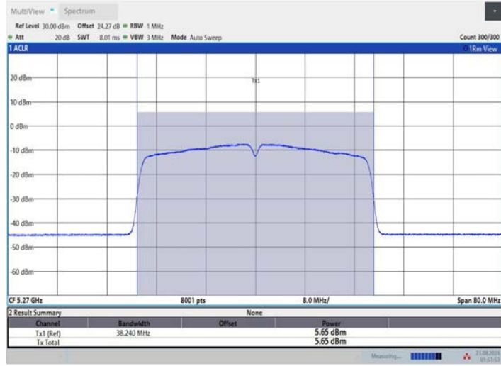
11N40MIMO_Ant3_5270
