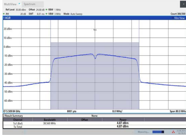
11N40MIMO_Ant2_5510
