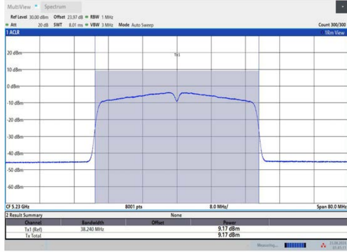
11N40MIMO_Ant3_5230
