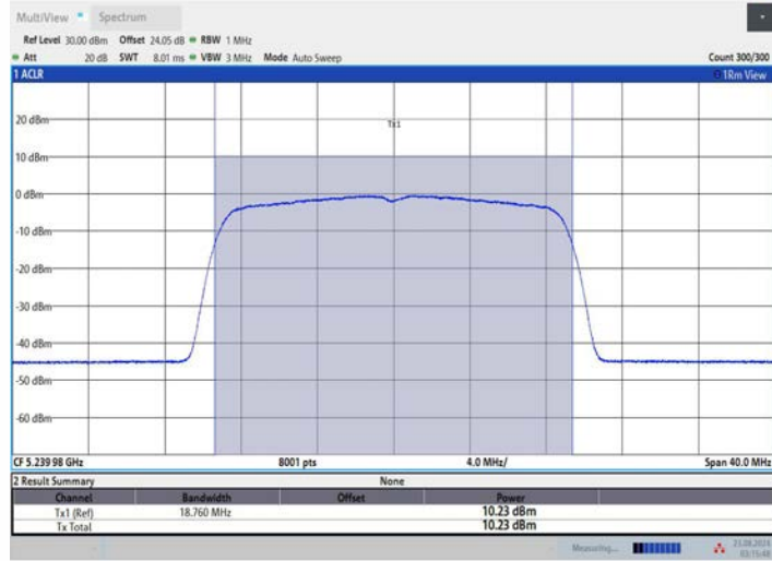
11AC20MIMO_Ant2_5240
