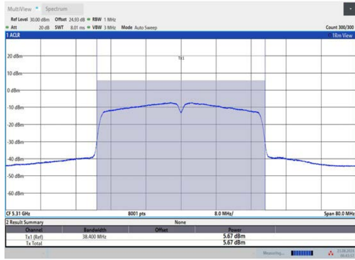
11AC40MIMO_Ant3_5310
