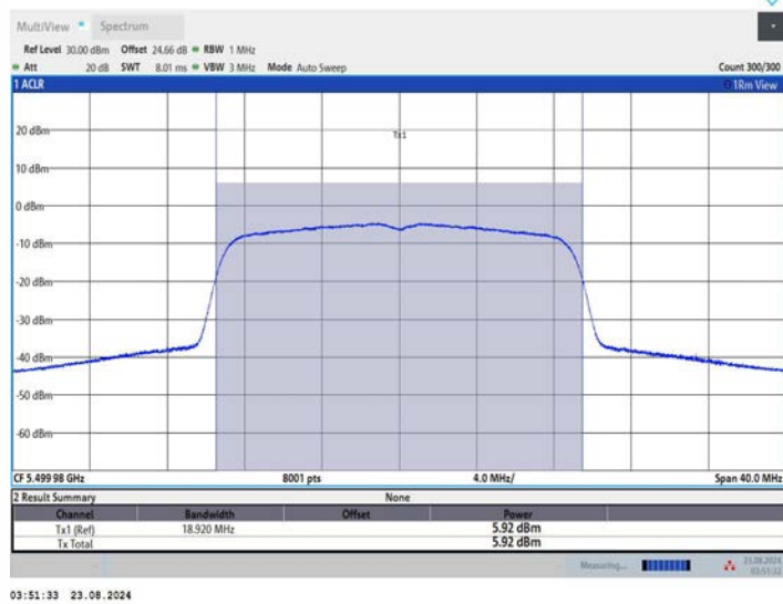
11AC20MIMO_Ant3_5500
