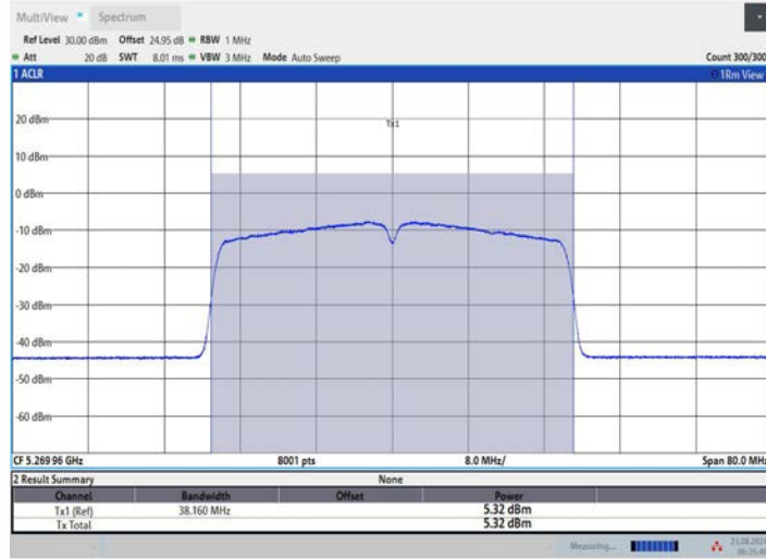
11AC40MIMO_Ant2_5270
