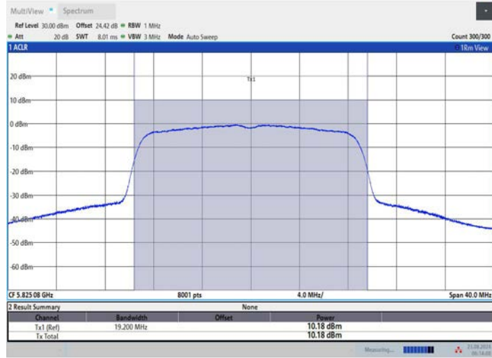
11AC20MIMO_Ant3_5825
