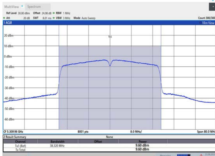
11AC40MIMO_Ant3_5310
