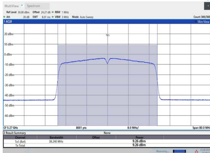
11N40MIMO_Ant3_5270
