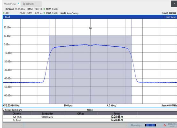
11AC20MIMO_Ant2_5260
