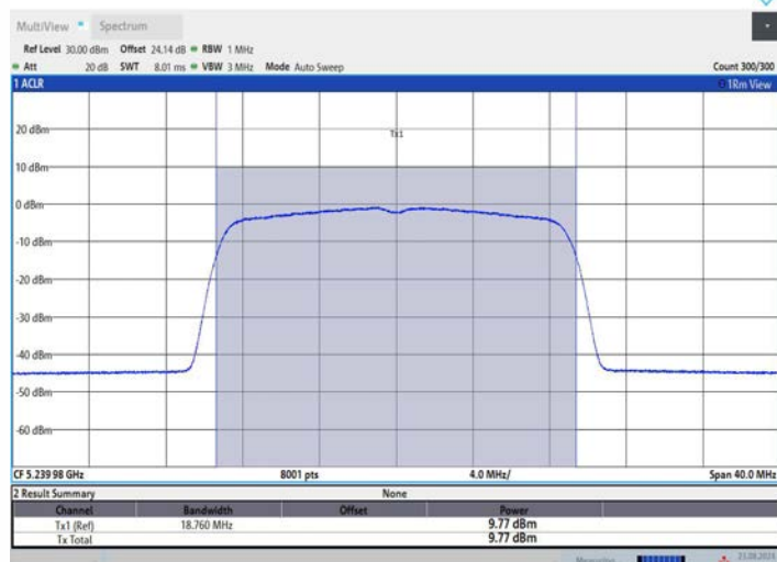
11AC20MIMO_Ant3_5240
