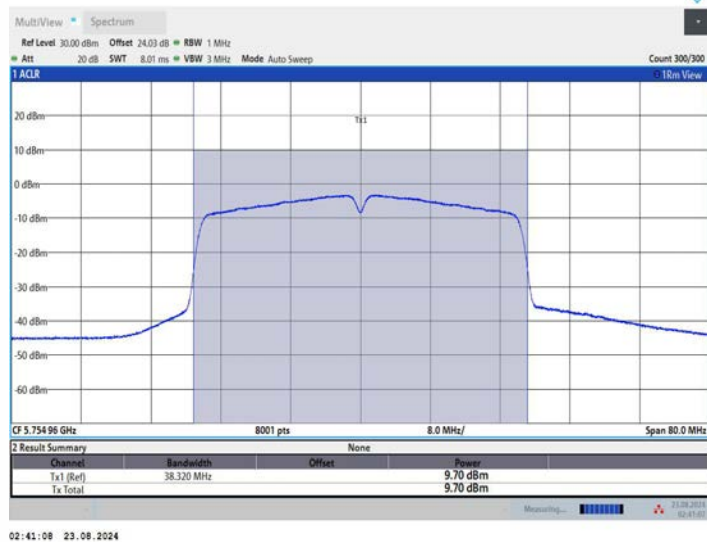
11N40MIMO_Ant3_5755
