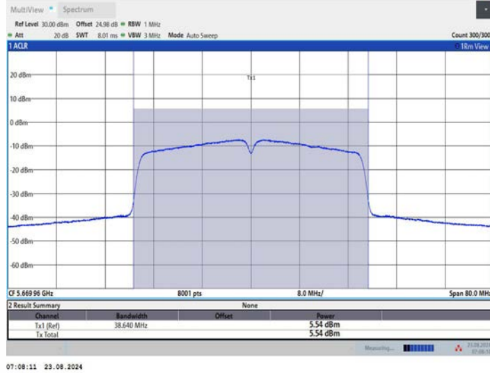
11AC40MIMO_Ant1_5670
