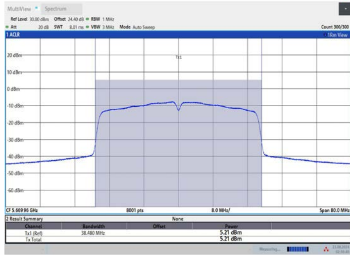
11N40MIMO_Ant3_5670
