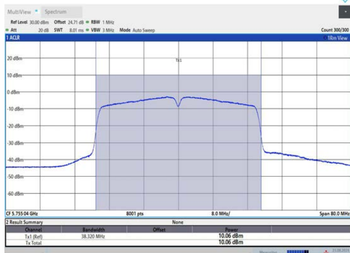
11AC40MIMO_Ant3_5755
