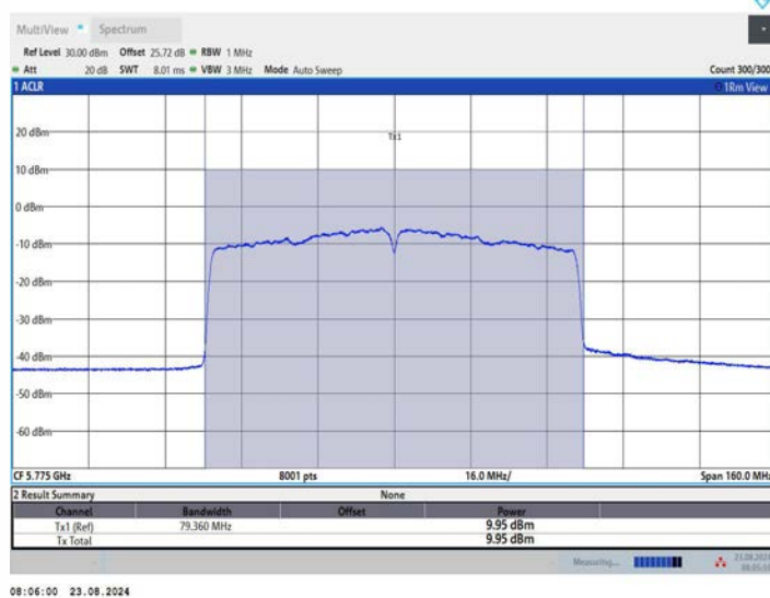
11AC80MIMO_Ant2_5775
