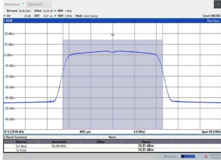
11A_Ant3_5280
