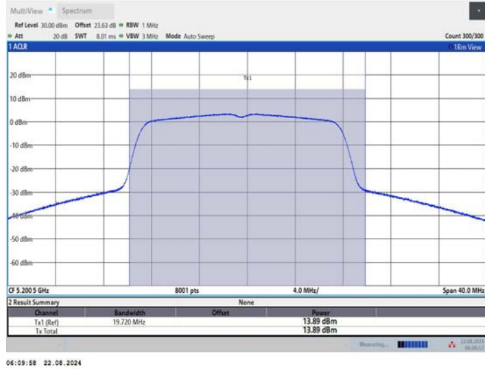
11A_Ant3_5200
