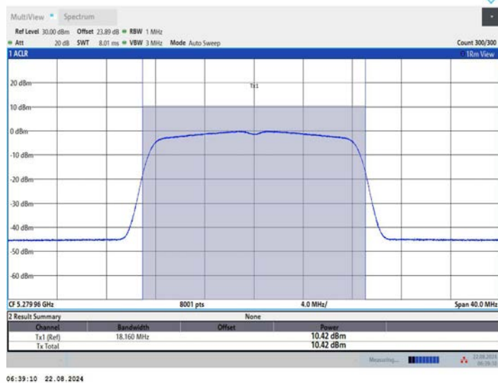
11A_Ant3_5280
