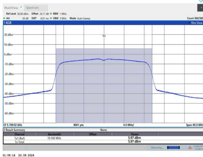
11N20MIMO_Ant2_5700
