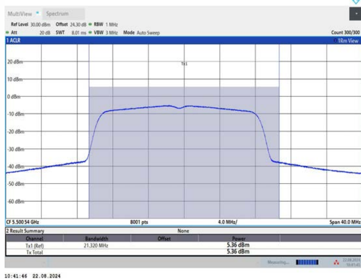
11N20MIMO_Ant2_5500
