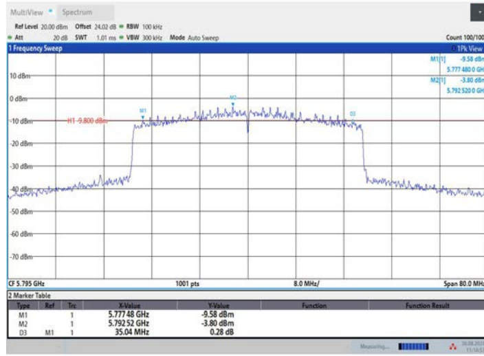
11BE40MIMO_Ant2_5795
