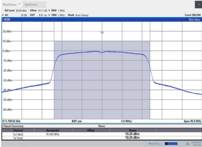
11N20MIMO_Ant3_5700
