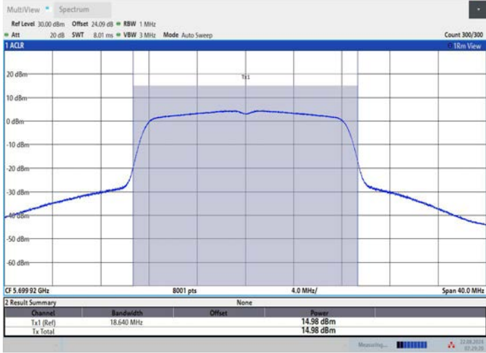
11A_Ant3_5700
