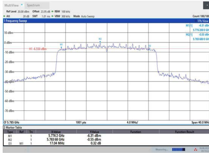
11BE20MIMO_Ant3_5785
