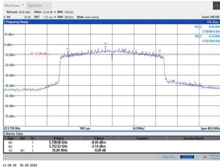
11BE40MIMO_Ant3_5755
