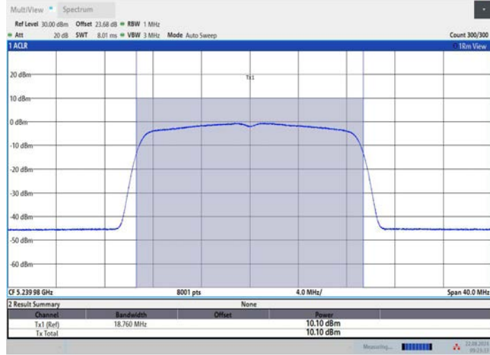
11N20MIMO_Ant2_5240
