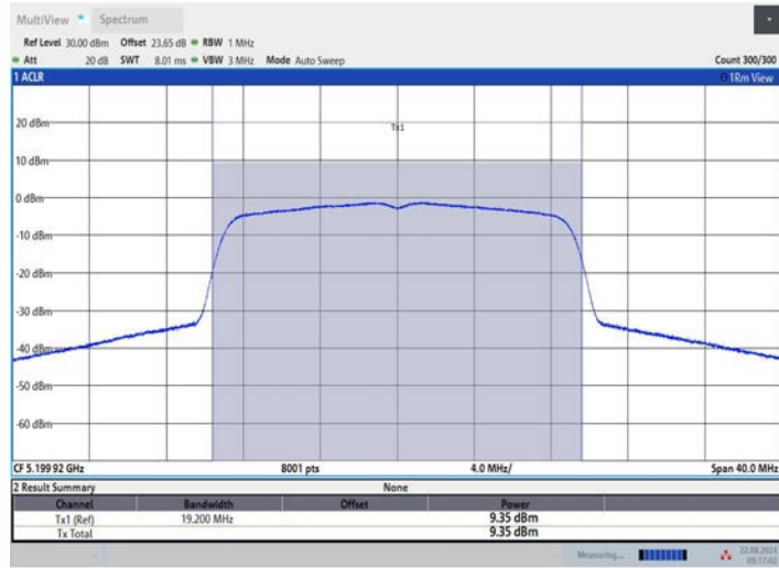
11N20MIMO_Ant3_5200
