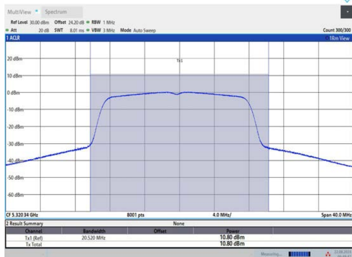
11A_Ant1_5320
