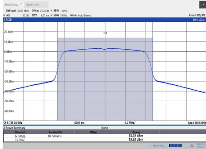
11A_Ant2_5785
