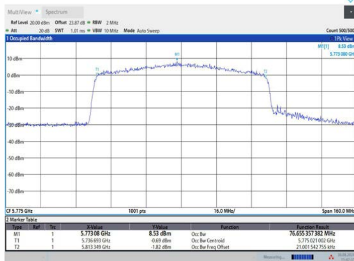
11BE80MIMO_Ant3_5775
