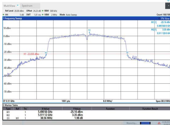
11N40MIMO_Ant3_5510
