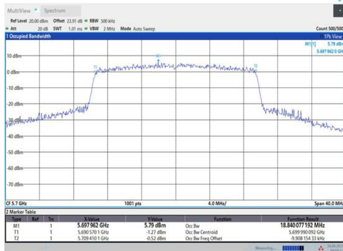
11BE20MIMO_Ant2_5700
