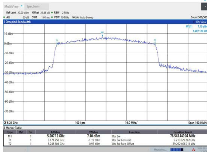
11BE80MIMO_Ant3_5210
