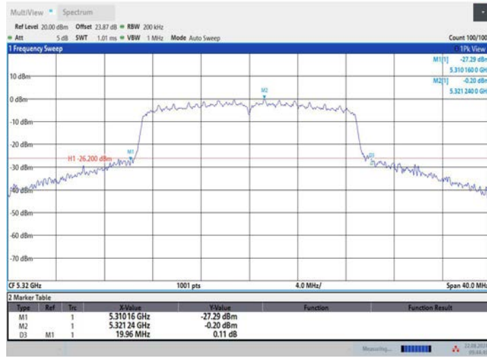
11N20MIMO_Ant3_5320
