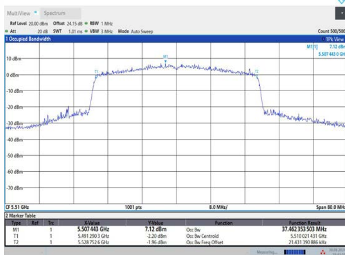
11BE40MIMO_Ant2_5510
