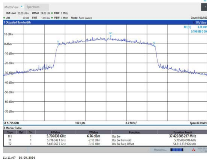
11BE40MIMO_Ant2_5795
