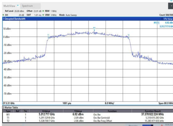
11BE40MIMO_Ant3_5310
