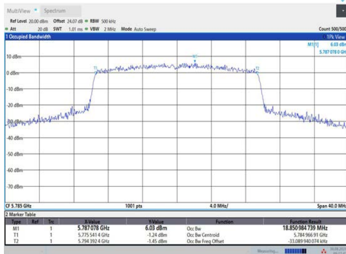
11BE20MIMO_Ant2_5785
