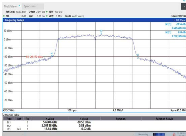
11A_Ant3_5700
