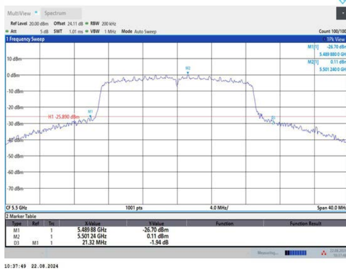
11N20MIMO_Ant3_5500
