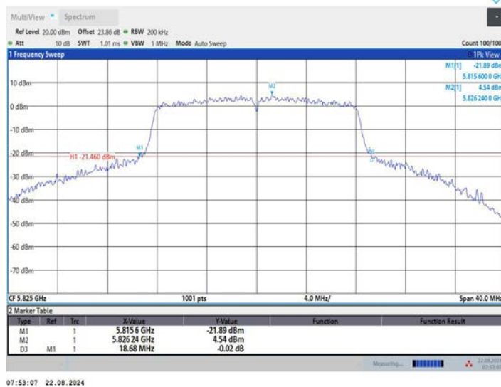
11A_Ant2_5825
