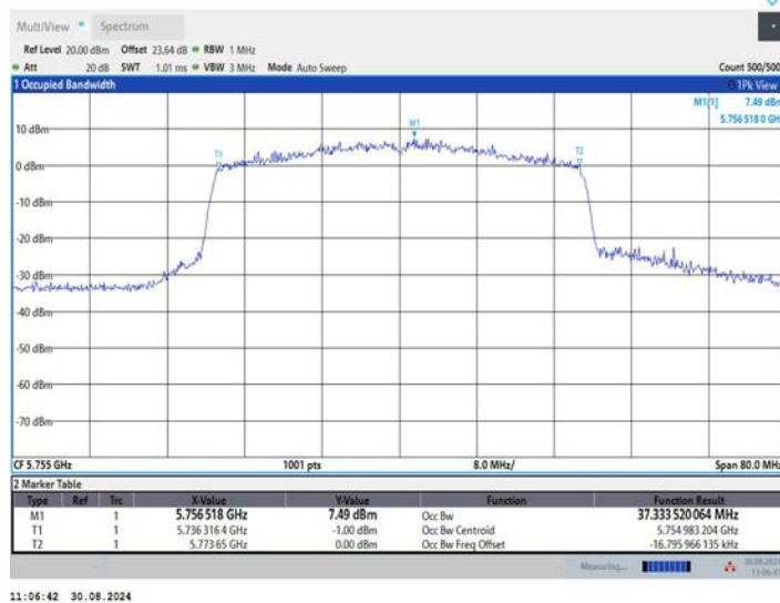
11BE40MIMO_Ant3_5755
