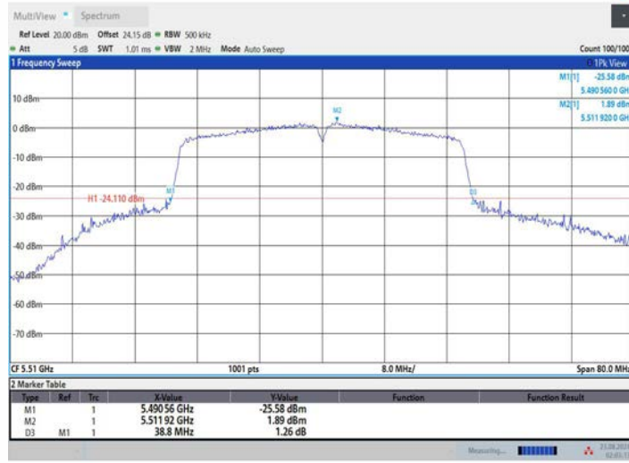
11N40MIMO_Ant2_5510
