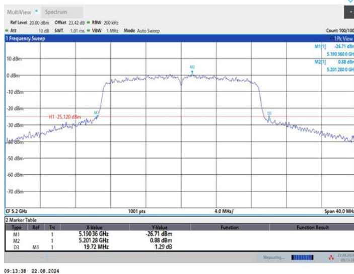
11N20MIMO_Ant2_5200
