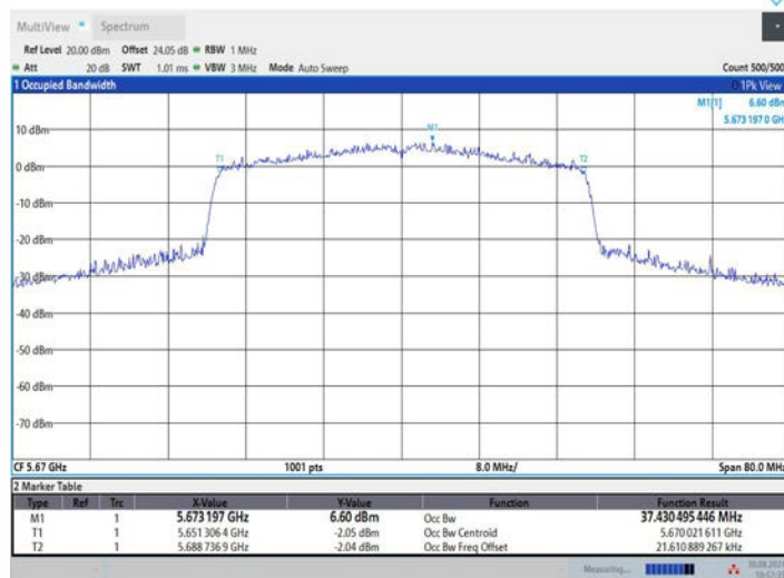
11BE40MIMO_Ant2_5670
