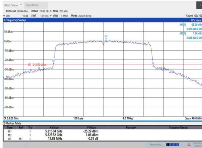
11AX20MIMO_Ant2_5825
