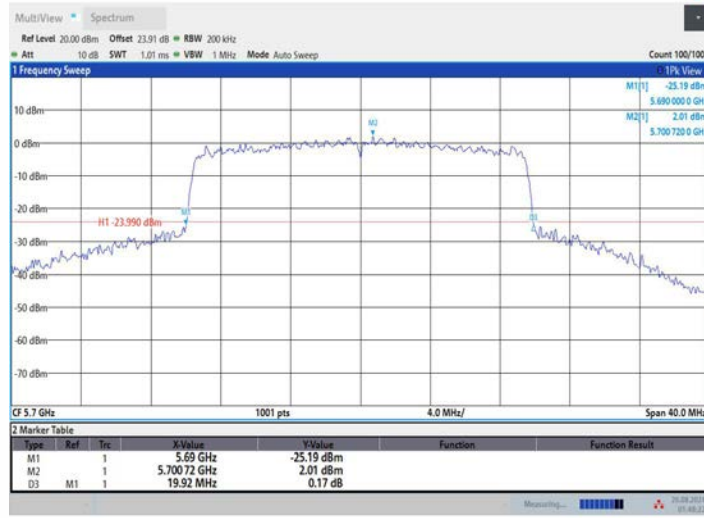
11AX20MIMO_Ant3_5700
