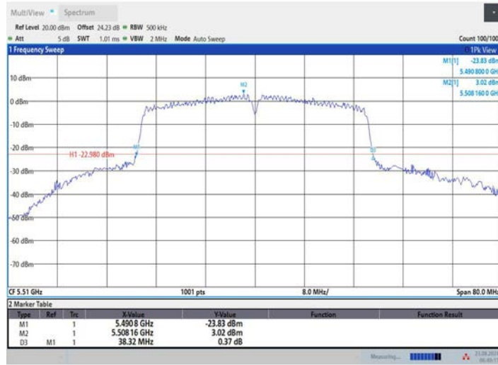
11AC40MIMO_Ant3_5510
