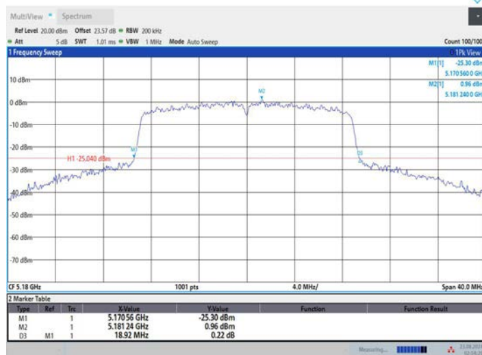
11AC20MIMO_Ant2_5180
