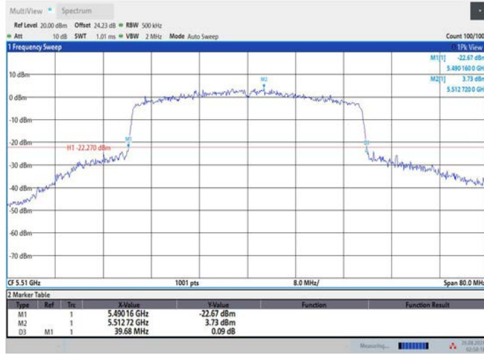
11AX40MIMO_Ant3_5510
