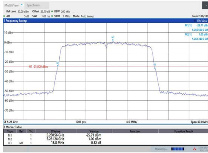
11AC20MIMO_Ant2_5260
