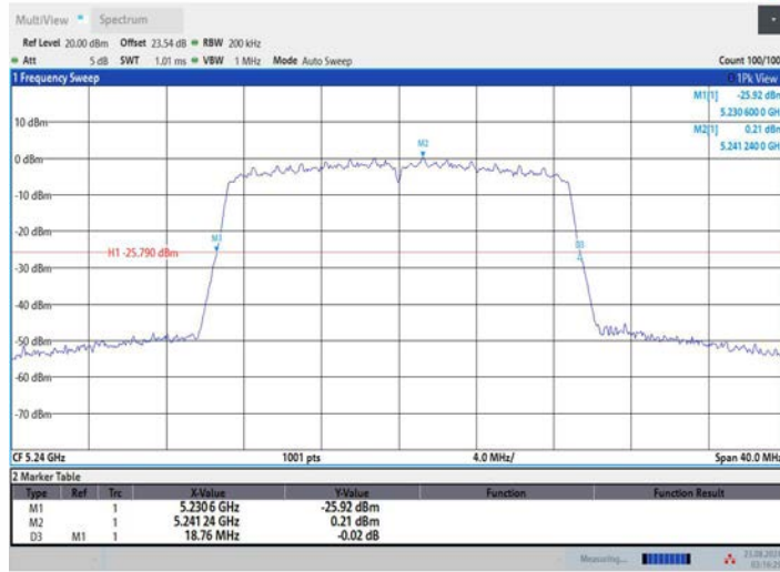
11AC20MIMO_Ant3_5240
