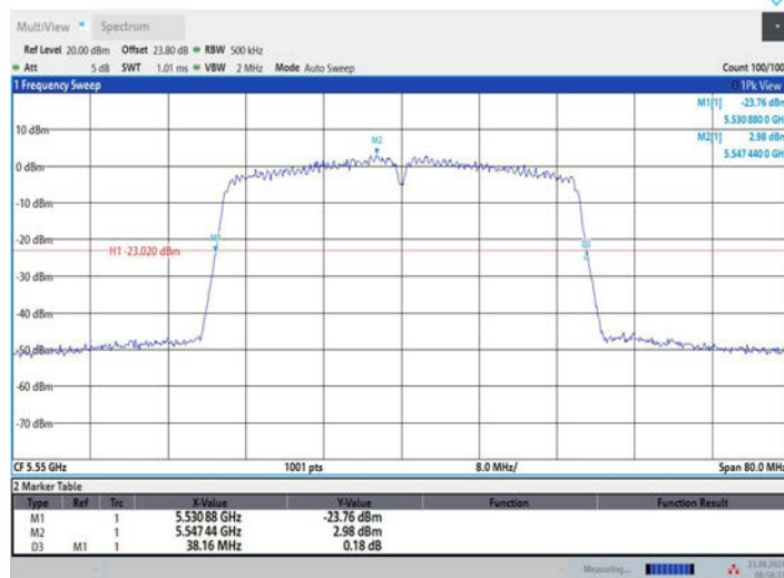
11AC40MIMO_Ant3_5550
