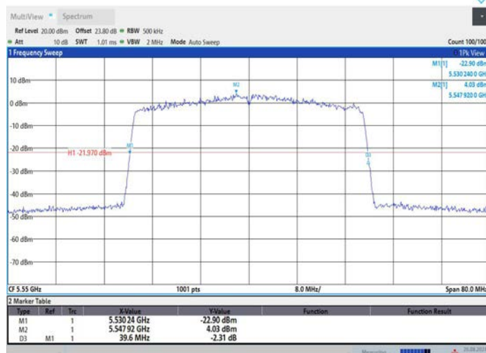
11AX40MIMO_Ant3_5550
