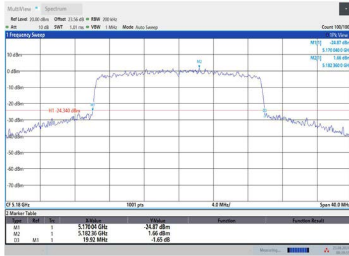
11AX20MIMO_Ant3_5180
