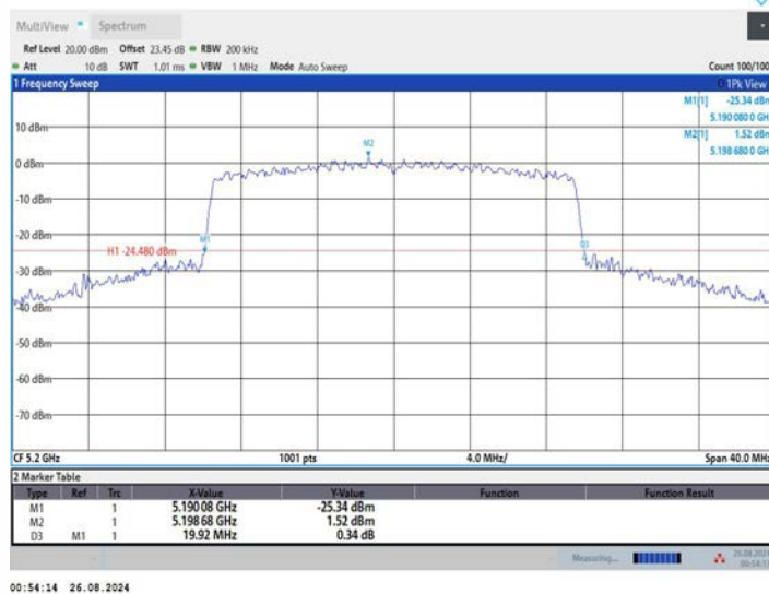
11AX20MIMO_Ant3_5200
