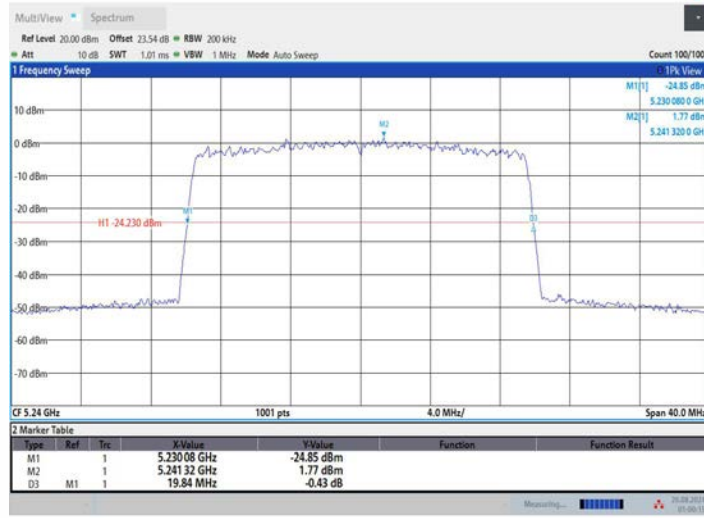
11AX20MIMO_Ant3_5240
