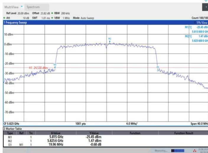
11AX20MIMO_Ant3_5825
