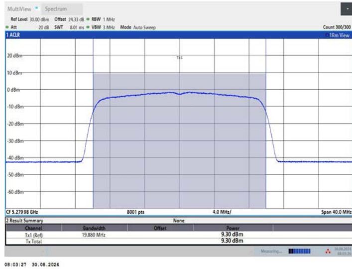
11BE20MIMO_Ant3_5280
