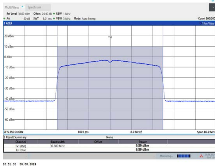
11BE40MIMO_Ant2_5550
