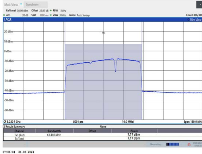
11BE80MIMO_Ant2_5290_484+242_OFDMA_4
