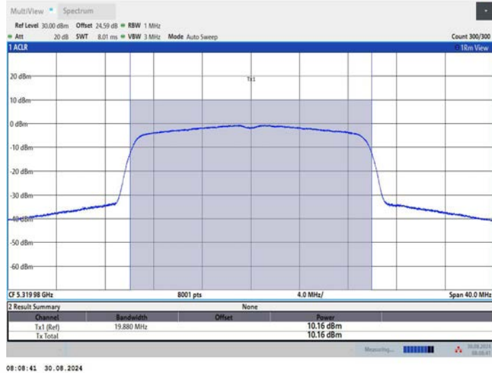
11BE20MIMO_Ant2_5320
