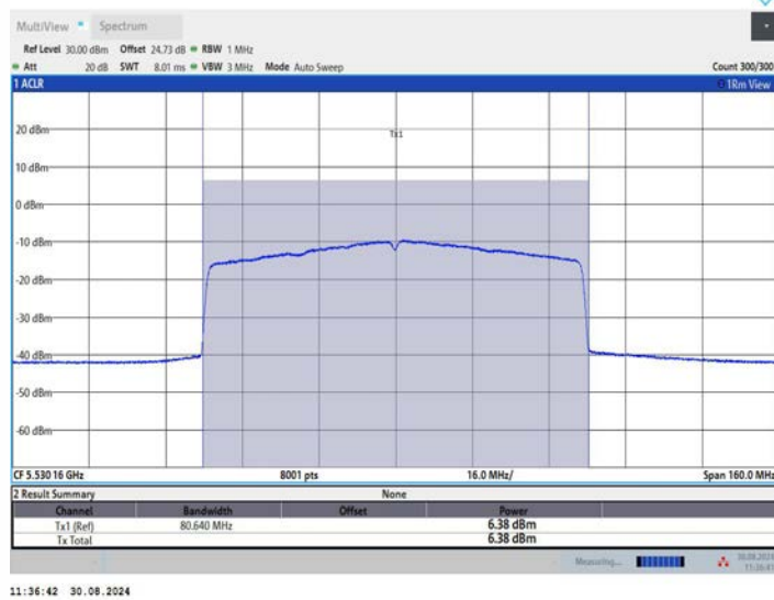
11BE80MIMO_Ant3_5530
