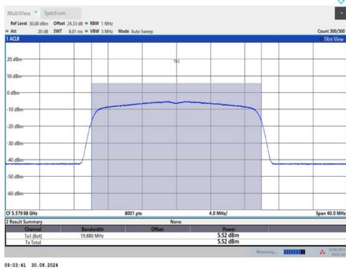
11BE20MIMO_Ant3_5580
