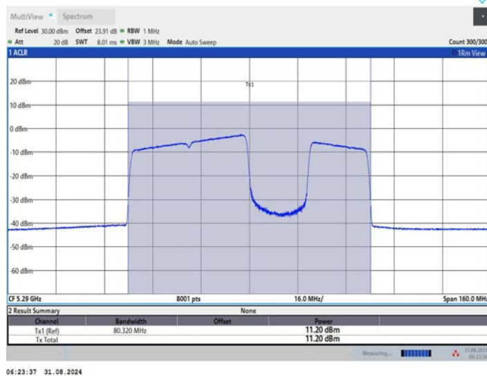
11BE80MIMO_Ant2_5290_484+242_OFDMA_4
