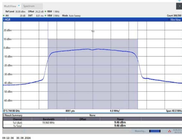
11BE20MIMO_Ant2_5745
