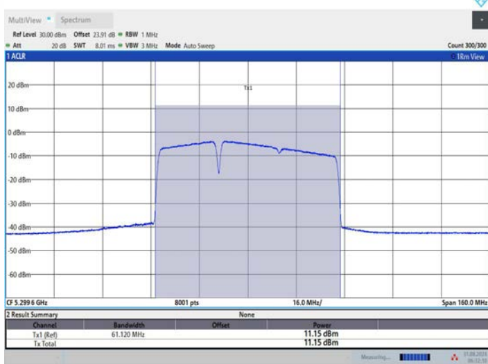
11BE80MIMO_Ant2_5290_484+242_OFDMA_2
