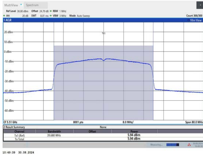
11BE40MIMO_Ant3_5510
