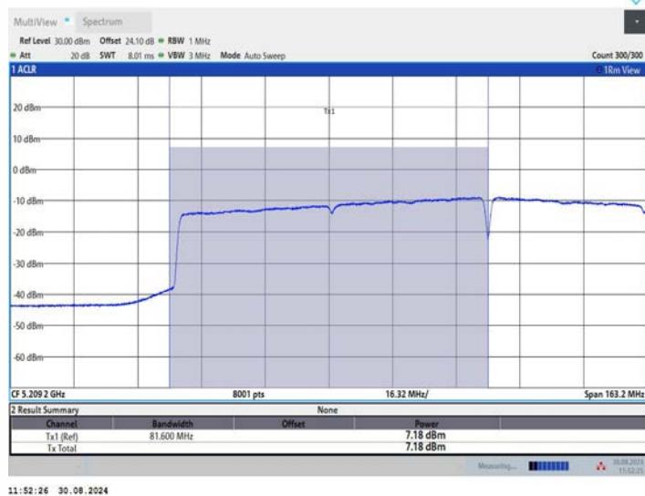
11BE160MIMO_Ant2_5250_UNII-1
