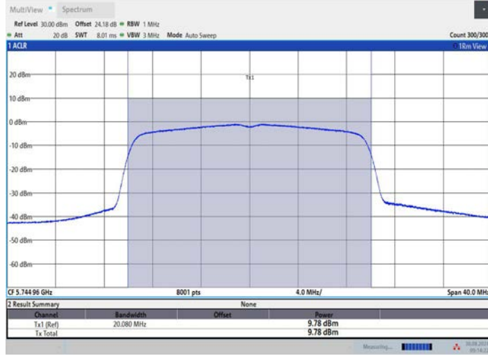
11BE20MIMO_Ant3_5745
