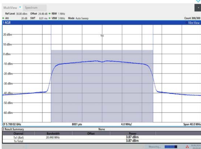
11BE20MIMO_Ant1_5700
