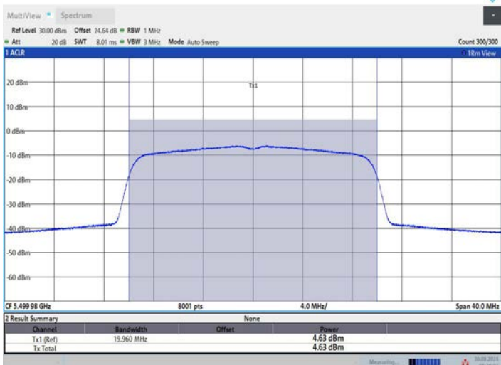
11BE20MIMO_Ant1_5500
