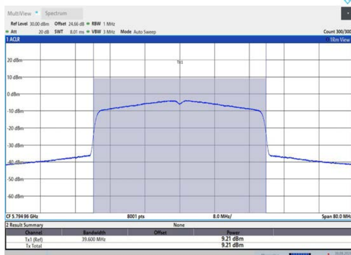
11BE40MIMO_Ant2_5795
