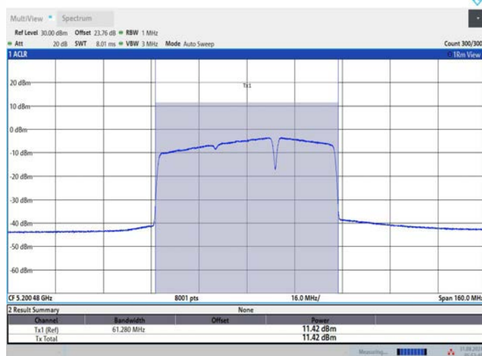
11BE80MIMO_Ant3_5210_484+242_OFDMA_1
