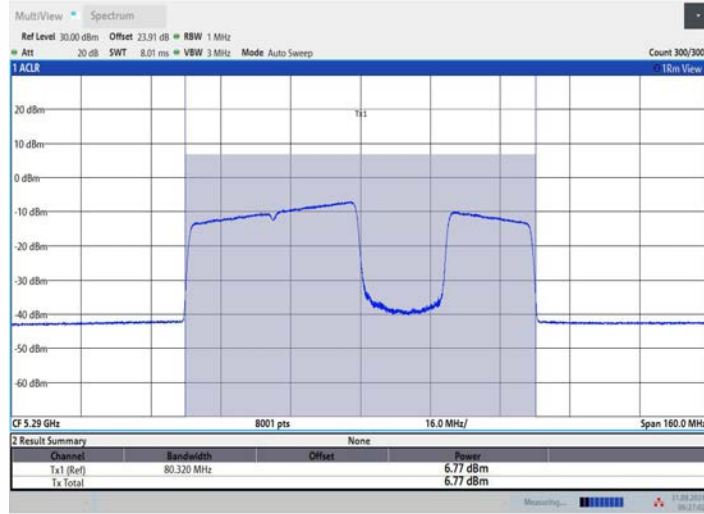
11BE80MIMO_Ant2_5290_484+242_OFDMA_3
