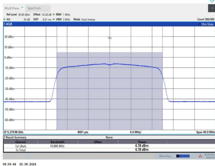
11BE20MIMO_Ant3_5280
