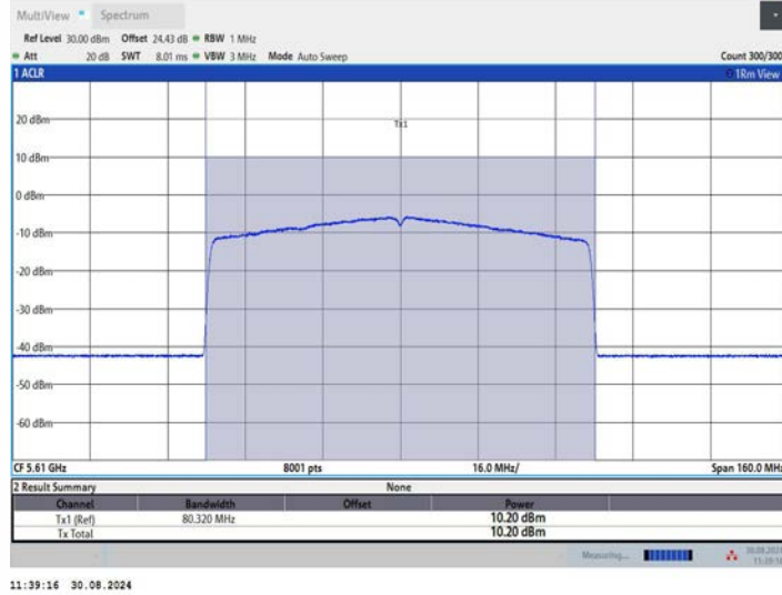
11BE80MIMO_Ant2_5610
