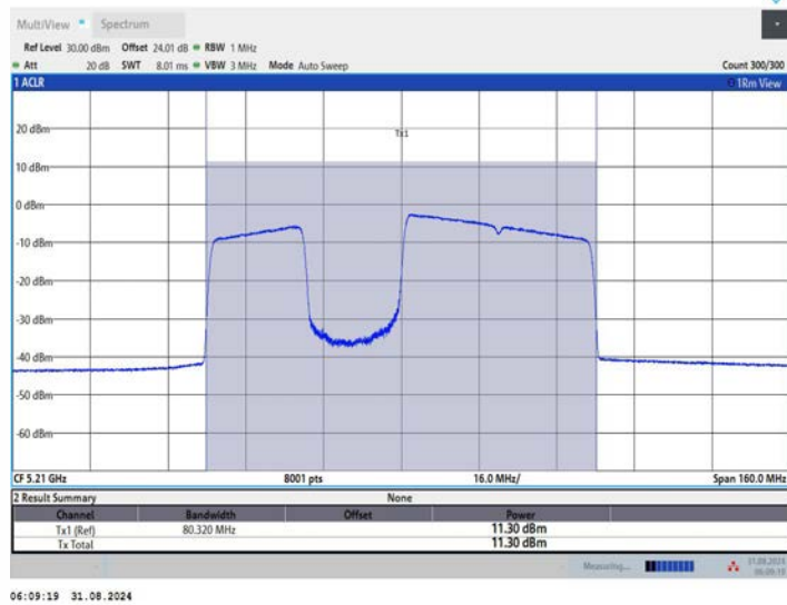
11BE80MIMO_Ant2_5210_484+242_OFDMA_3
