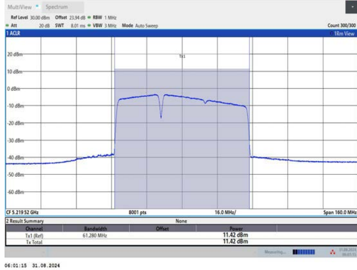
11BE80MIMO_Ant2_5210_484+242_OFDMA_2
