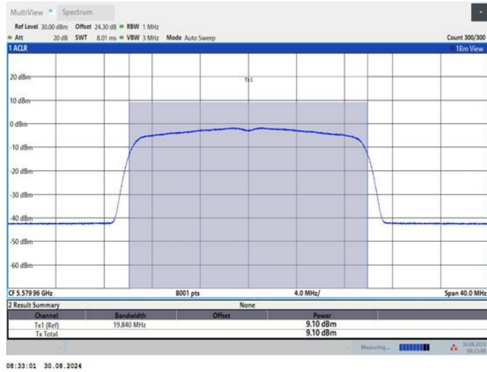
11BE20MIMO_Ant3_5580
