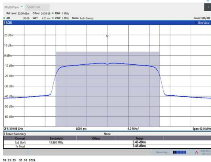
11BE20MIMO_Ant1_5320
