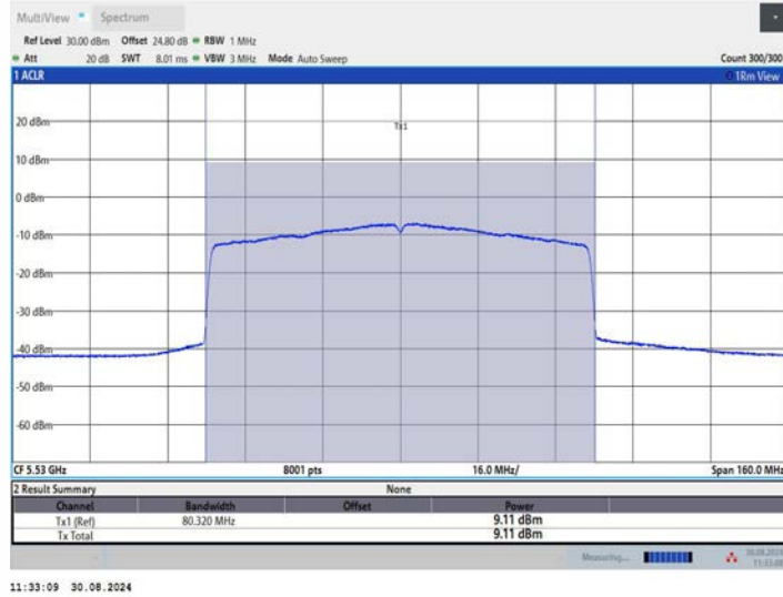
11BE80MIMO_Ant3_5530
