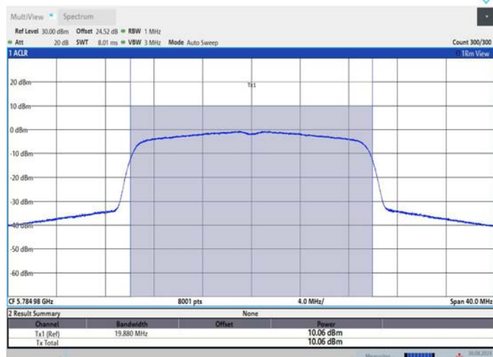
11BE20MIMO_Ant3_5785
