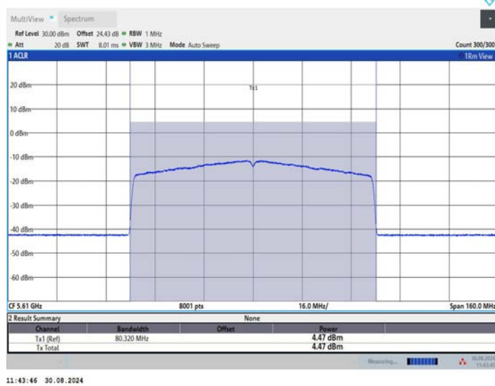
11BE80MIMO_Ant1_5610
