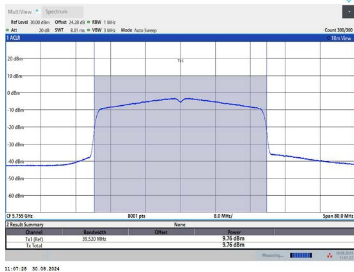
11BE40MIMO_Ant3_5755
