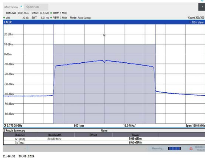
11BE80MIMO_Ant2_5775
