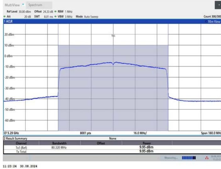
11BE80MIMO_Ant2_5290
