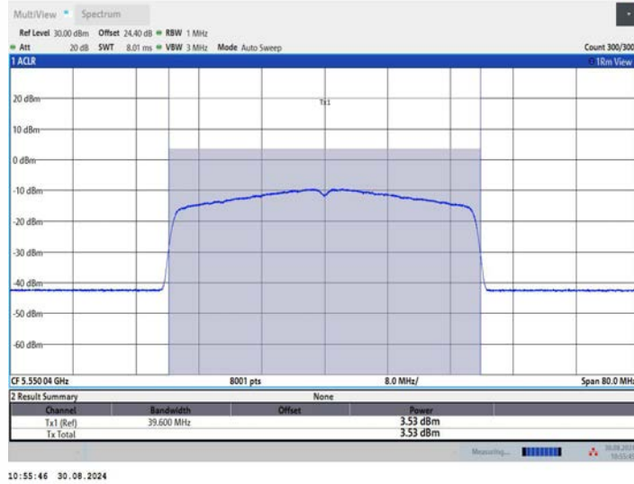
11BE40MIMO_Ant1_5550
