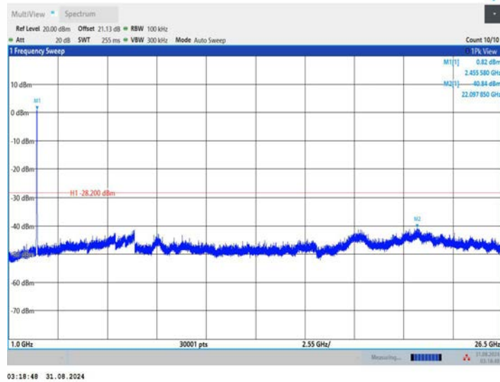
11BE40MIMO_Ant2_2452_0~Reference
