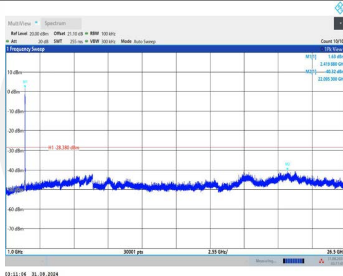
11BE40MIMO_Ant2_2422_0~Reference
