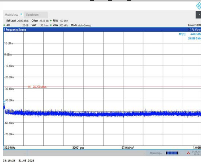
11BE40MIMO_Ant1_2452_30~1000
