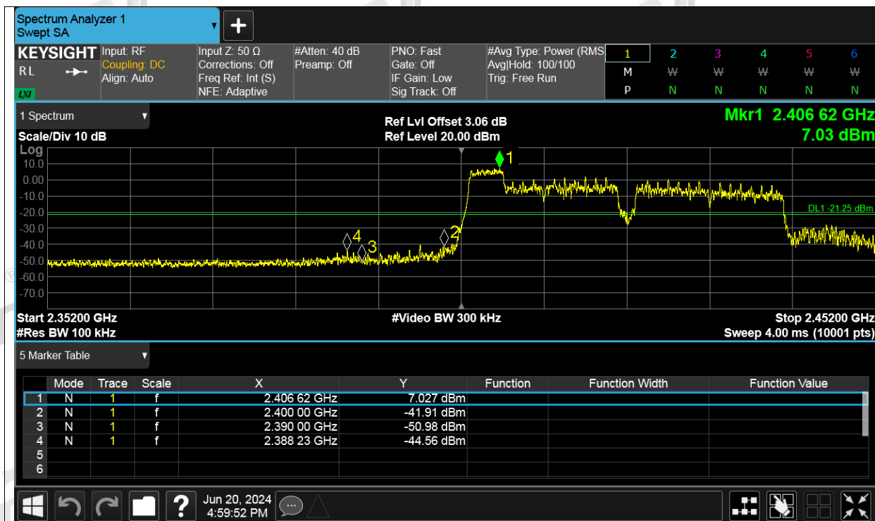
Band Edge NVNT ax40 52RU Index 37 2422MHz Ant2 Ref
