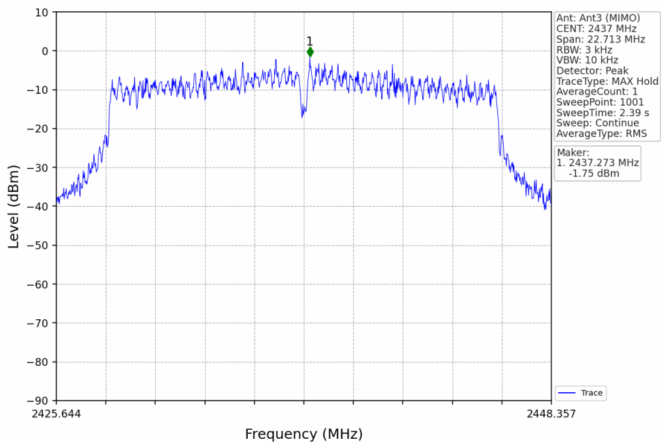
802.11n(HT20)_MCH_2437MHz_Ant3 (MIMO)_NTNV
