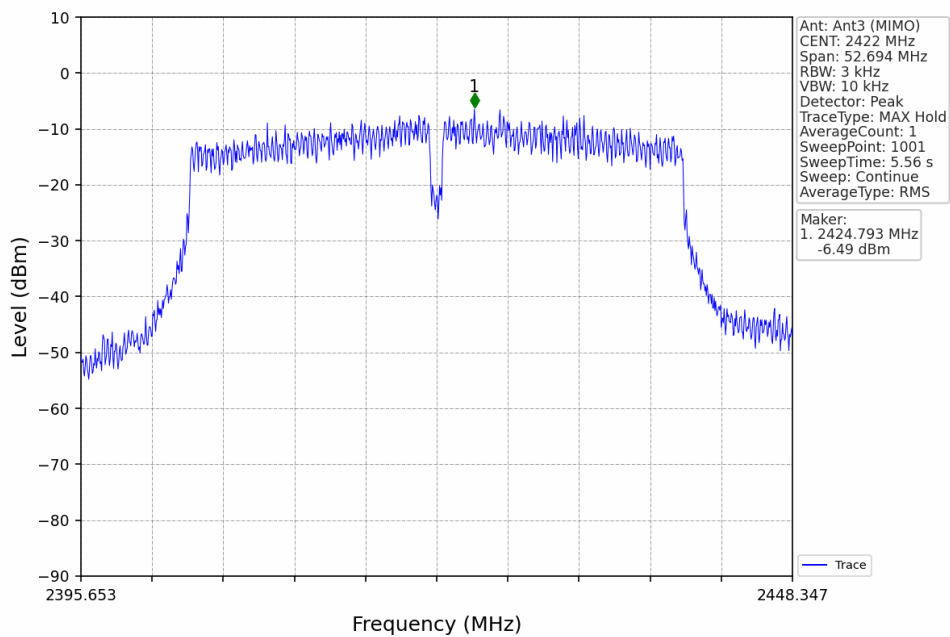
802.11n(HT40)_LCH_2422MHz_Ant3 (MIMO)_NTNV
