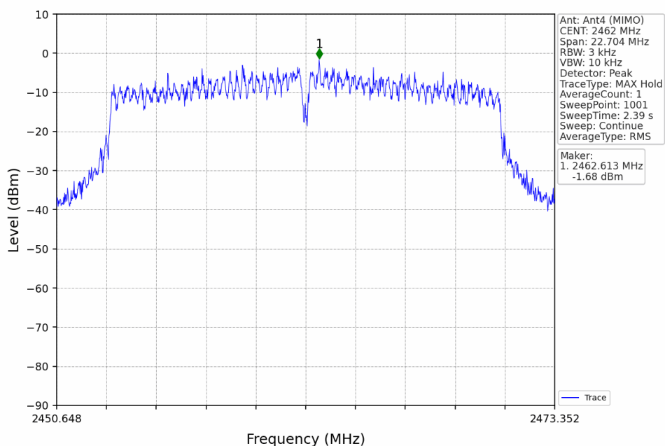
802.11n(HT20)_HCH_2462MHz_Ant4 (MIMO)_NTNV
