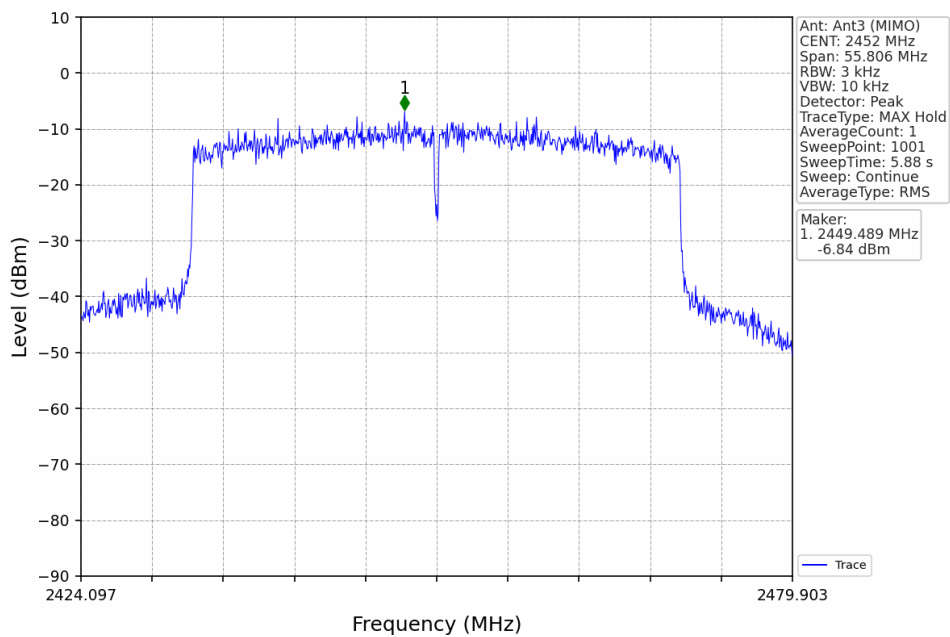
802.11ax(HEW40)_HCH_2452MHz_RU484_Left_Ant3 (MIMO)_NTNV
