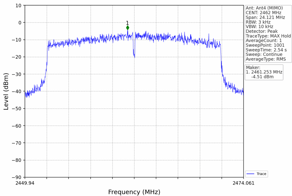
802.11ax(HEW20)_HCH_2462MHz_RU242_Left_Ant4 (MIMO)_NTNV
