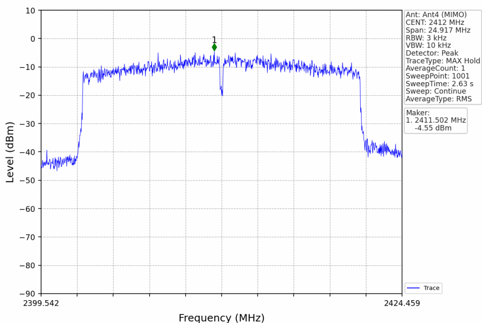
802.11ax(HEW20)_LCH_2412MHz_RU242_Left_Ant4 (MIMO)_NTNV
