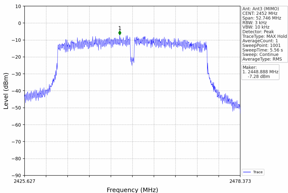
802.11n(HT40)_HCH_2452MHz_Ant3 (MIMO)_NTNV
