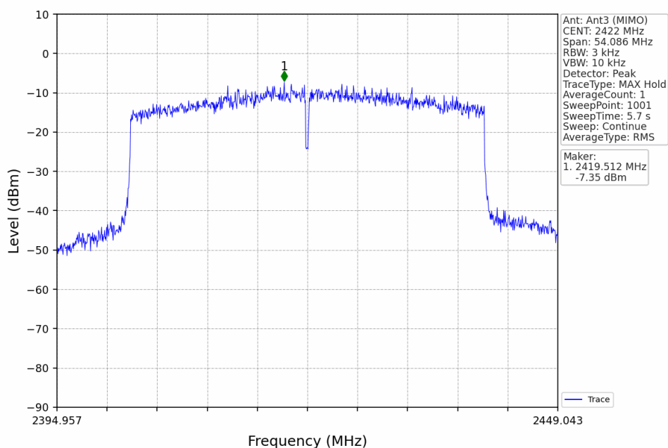
802.11ax(HEW40)_LCH_2422MHz_RU484_Left_Ant3 (MIMO)_NTNV
