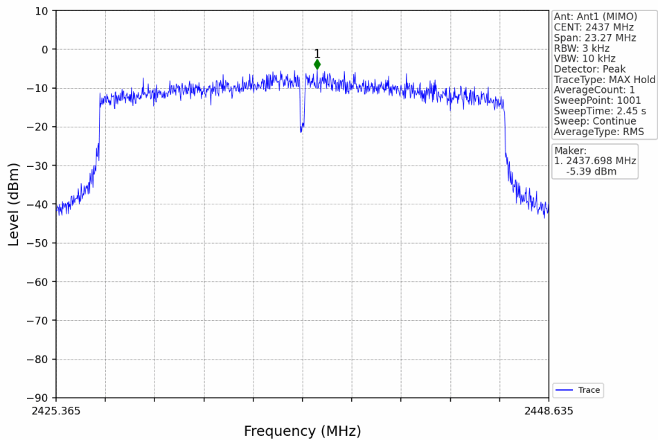
802.11ax(HEW20)_MCH_2437MHz_RU242_Left_Ant1 (MIMO)_NTNV
