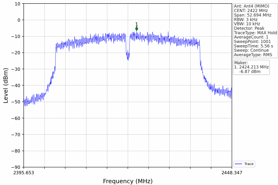
802.11n(HT40)_LCH_2422MHz_MIMO_NTNV
