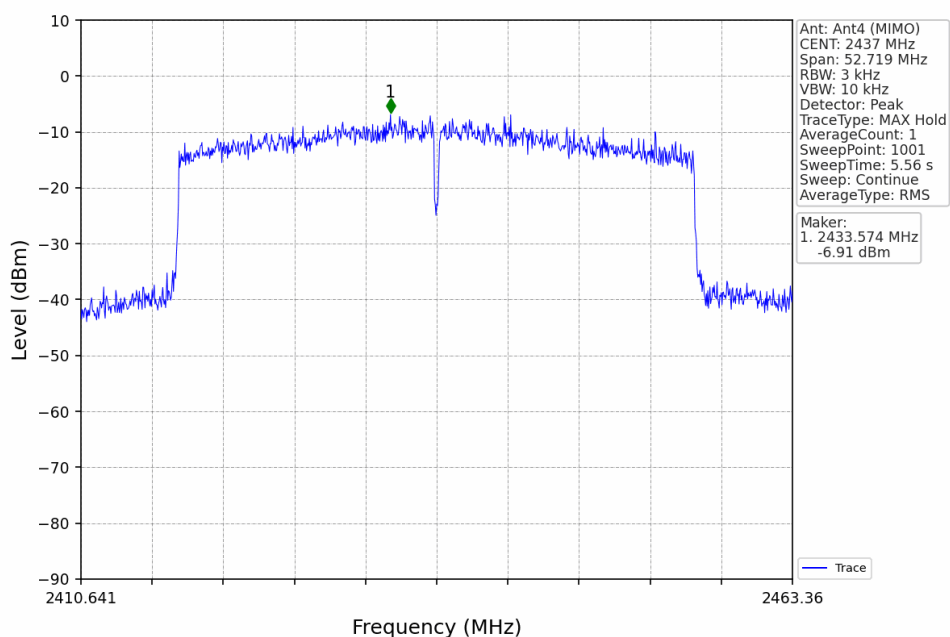
802.11ax(HEW40)_MCH_2437MHz_RU484_Left_Ant4 (MIMO)_NTNV
