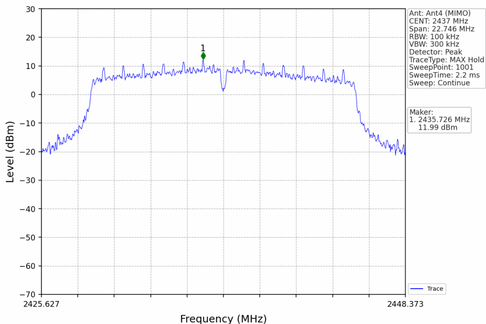
802.11g_MCH_2437MHz_Ant4 (MIMO)_NTNV
