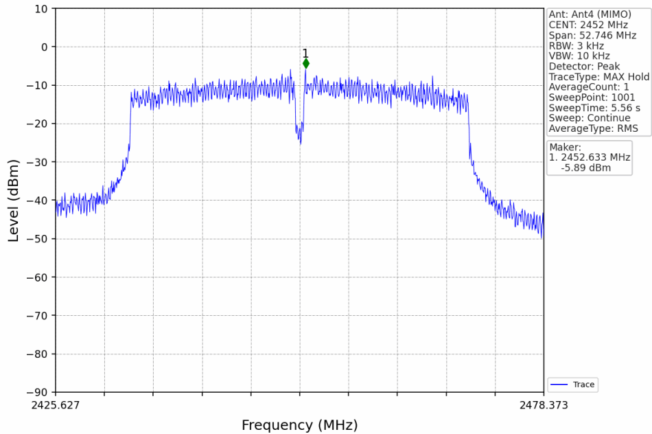
802.11n(HT40)_HCH_2452MHz_MIMO_NTNV
