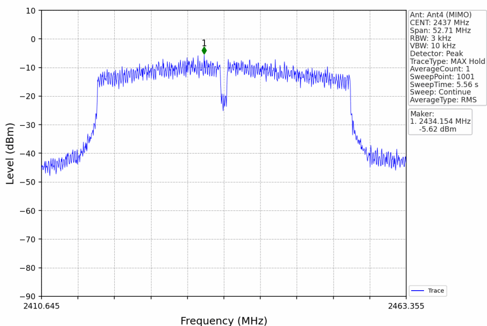
802.11n(HT40)_MCH_2437MHz_Ant4 (MIMO)_NTNV
