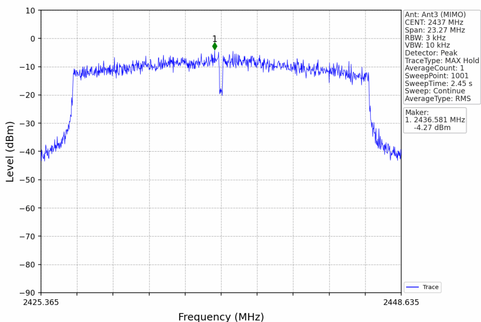
802.11ax(HEW20)_MCH_2437MHz_RU242_Left_Ant3 (MIMO)_NTNV
