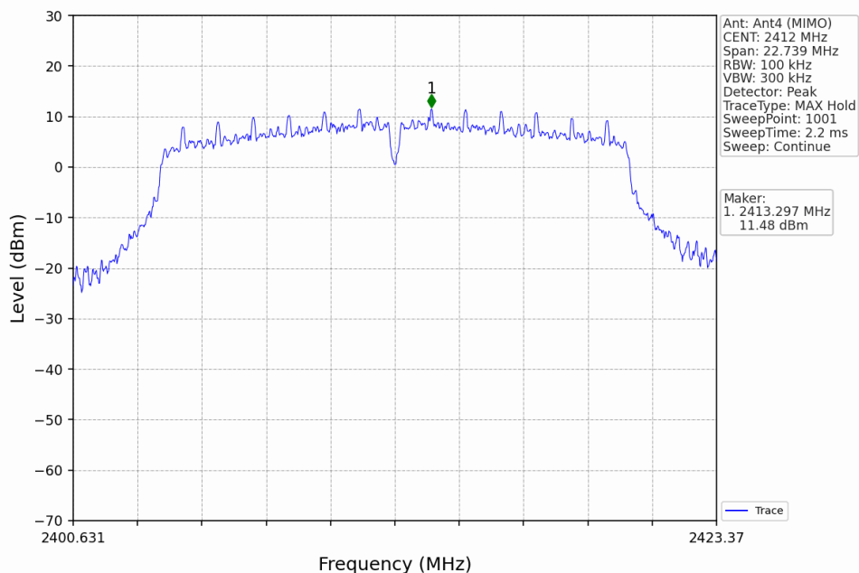
802.11g_LCH_2412MHz_Ant4 (MIMO)_NTNV
