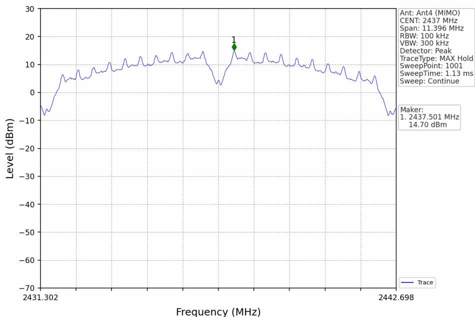
802.11b_MCH_2437MHz_Ant4 (MIMO)_NTNV
