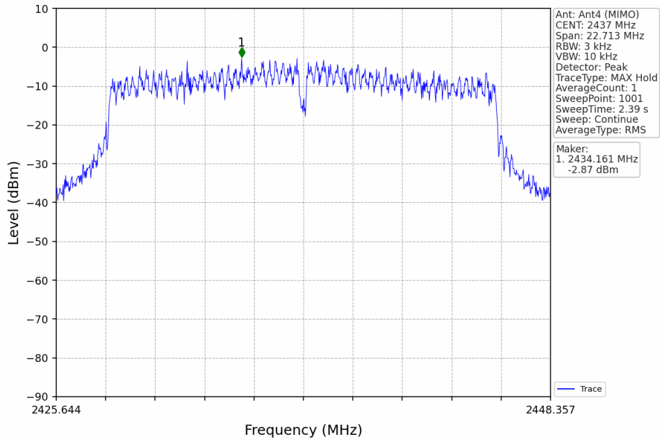
802.11n(HT20)_MCH_2437MHz_MIMO_NTNV
