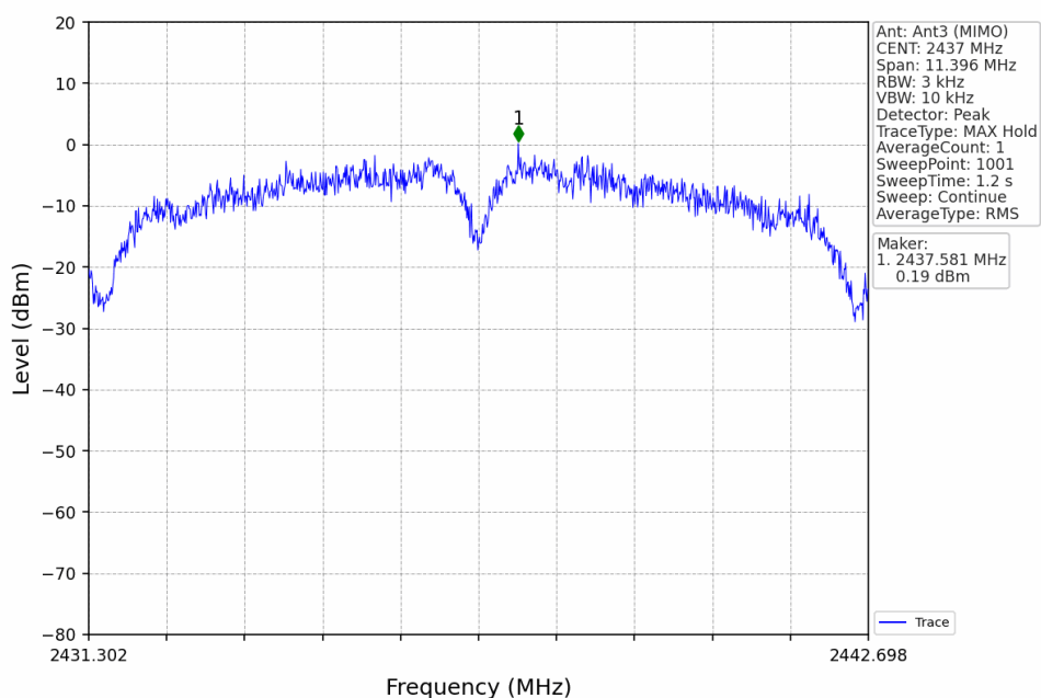
802.11b_MCH_2437MHz_Ant3 (MIMO)_NTNV
