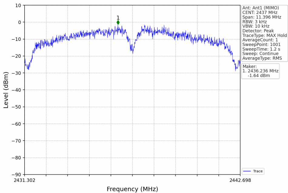
802.11b_MCH_2437MHz_Ant1 (MIMO)_NTNV
