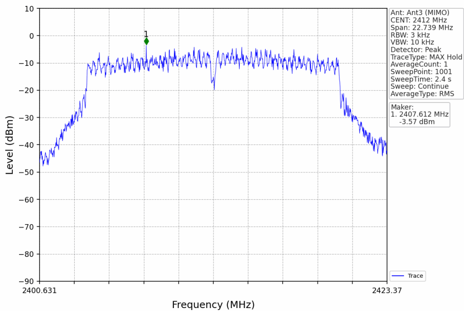
802.11g_LCH_2412MHz_Ant3 (MIMO)_NTNV
