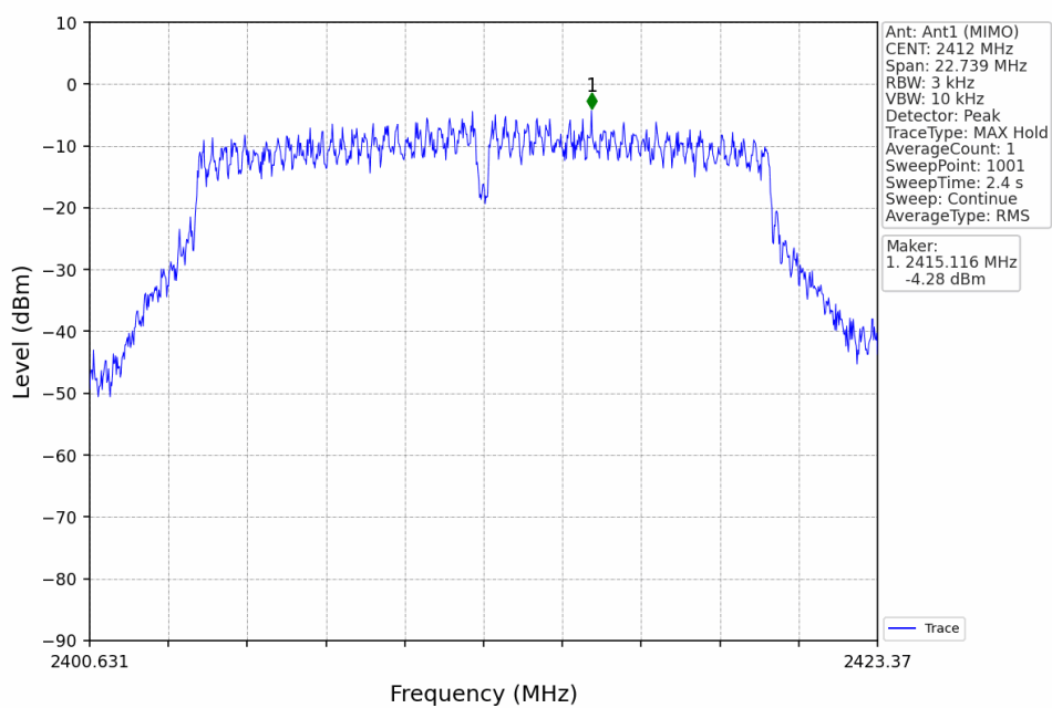
802.11g_LCH_2412MHz_Ant1 (MIMO)_NTNV
