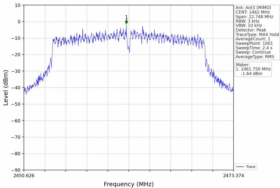
802.11g_HCH_2462MHz_Ant3 (MIMO)_NTNV
