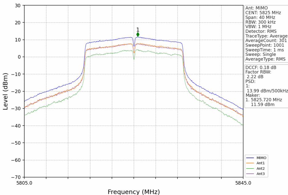
802.11n(HT20)_HCH_5825MHz_MIMO_NTNV
