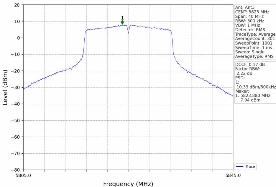
802.11a_HCH_5825MHz_MIMO_NTNV
