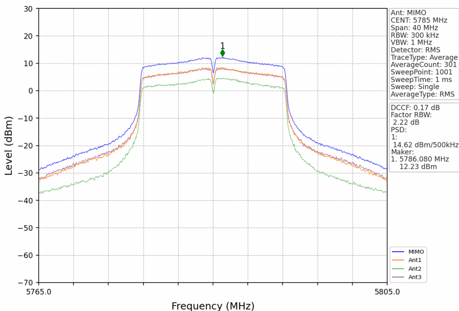
802.11a_MCH_5785MHz_MIMO_NTNV
