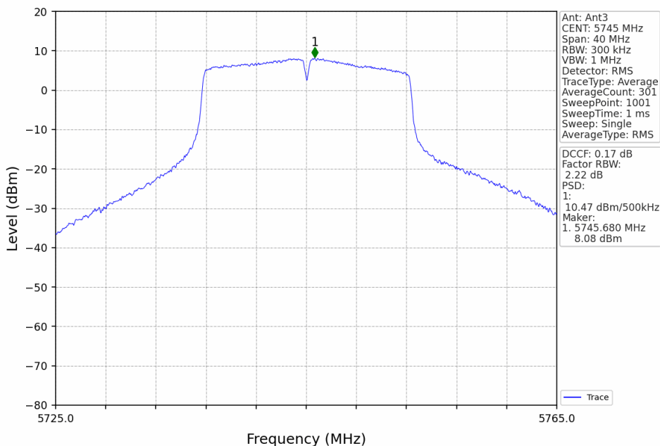
802.11a_LCH_5745MHz_MIMO_NTNV
