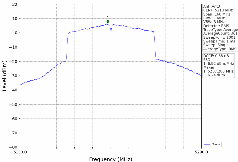
802.11ac(VHT80)_MCH_5210MHz_MIMO_NTNV
