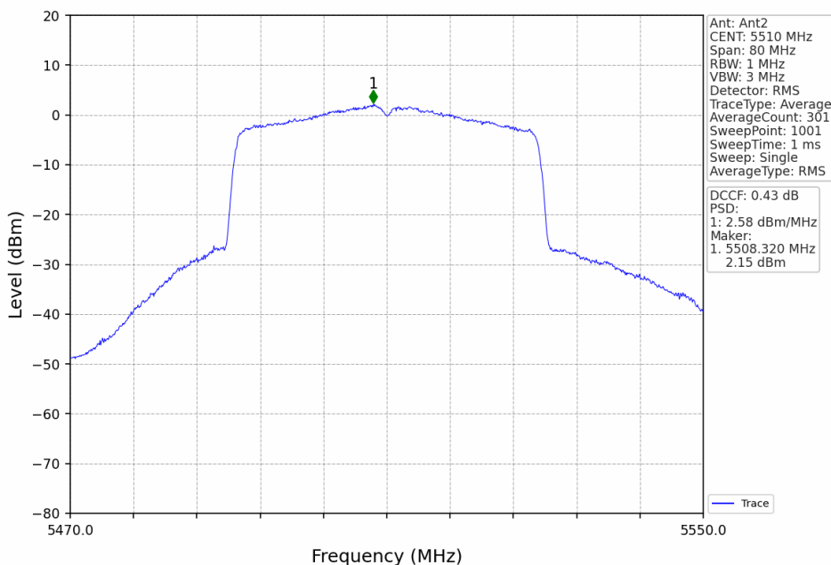
802.11ax(HEW40)_LCH_5510MHz_RU484_Left_Ant2_NTNV
