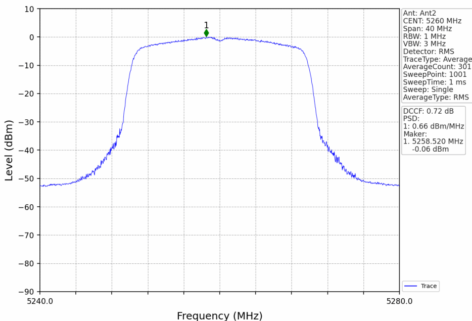
802.11ax(HEW20)_LCH_5260MHz_RU242_Left_Ant2_NTNV
