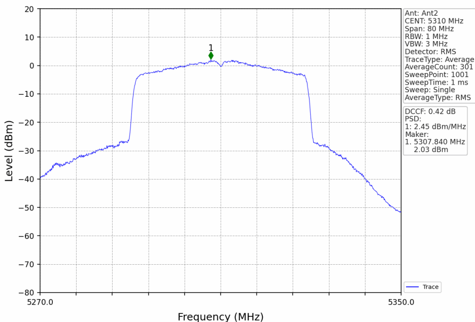
802.11ax(HEW40)_HCH_5310MHz_RU484_Left_Ant2_NTNV
