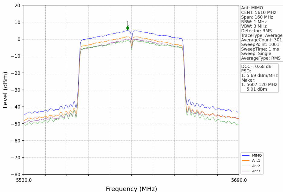
802.11ac(VHT80)_HCH_5610MHz_MIMO_NTNV
