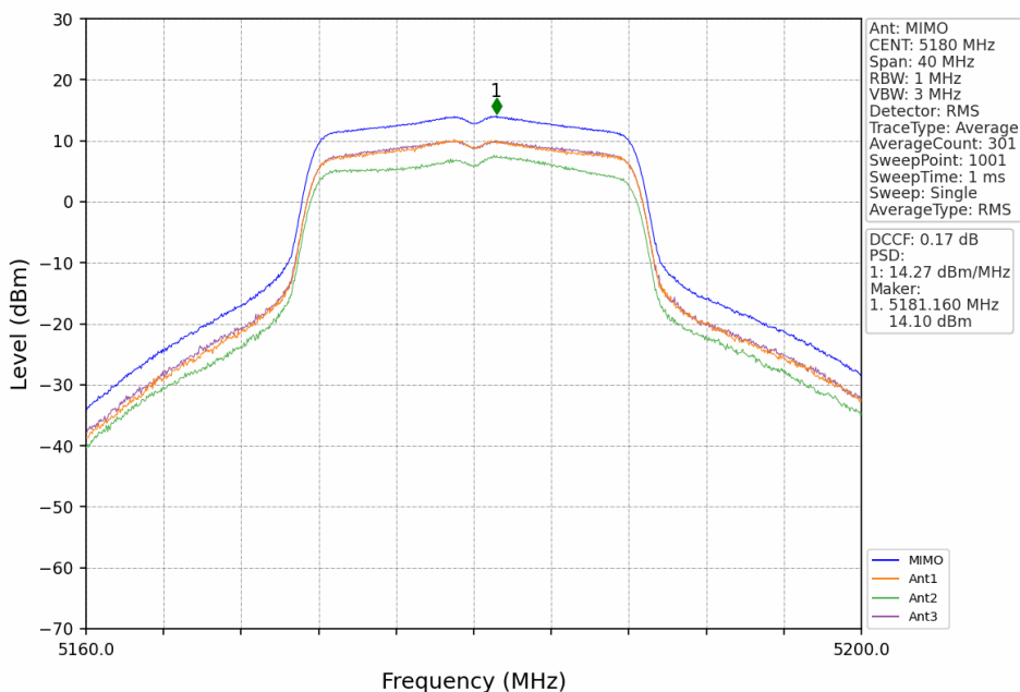
802.11a_LCH_5180MHz_MIMO_NTNV
