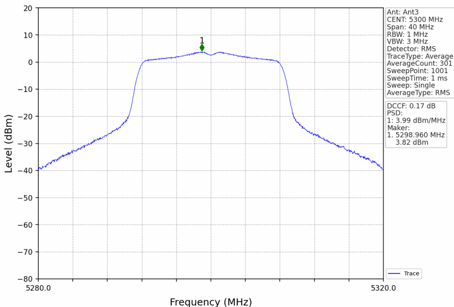
802.11a_MCH_5300MHz_MIMO_NTNV
