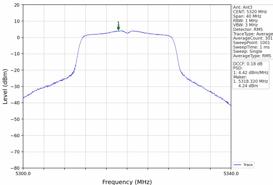
802.11n(HT20)_HCH_5320MHz_MIMO_NTNV
