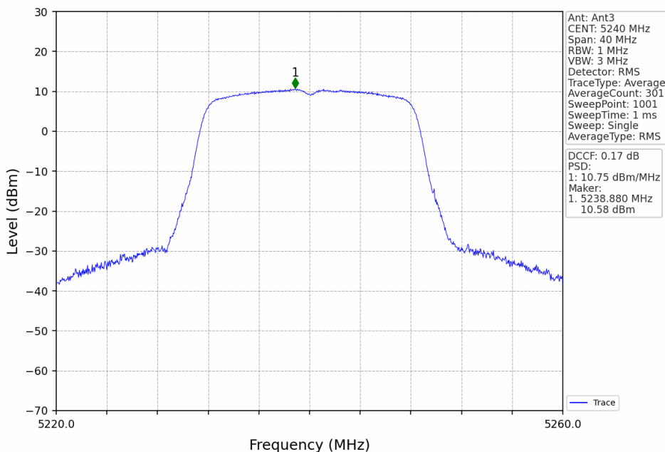
802.11a_HCH_5240MHz_MIMO_NTNV
