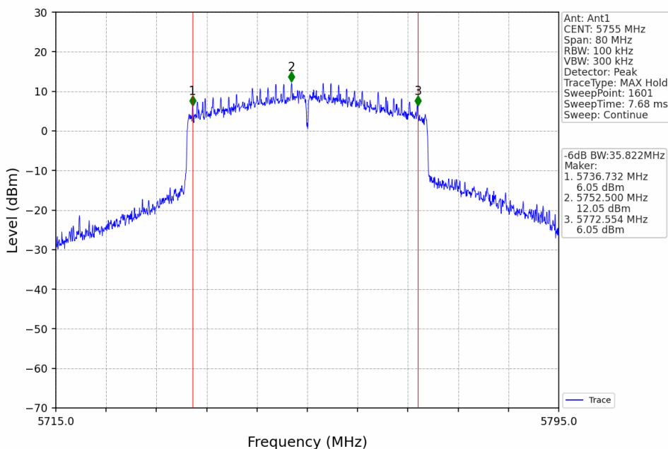
802.11ax(HEW40)_LCH_5755MHz_RU484_Left_Ant1_NTNV
