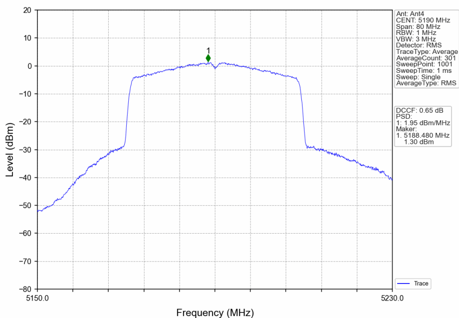
802.11ax(HEW40)_LCH_5190MHz_RU484_Left_Ant4_NTNV
