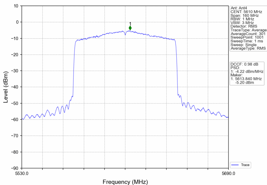
802.11ax(HEW80)_HCH_5610MHz_RU996_Left_Ant4_NTNV
