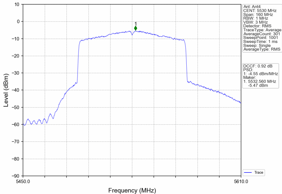
802.11ax(HEW80)_LCH_5530MHz_RU996_Left_MIMO_NTNV
