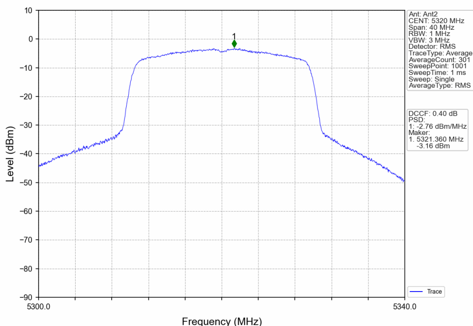
802.11ax(HEW20)_HCH_5320MHz_RU242_Left_Ant2_NTNV
