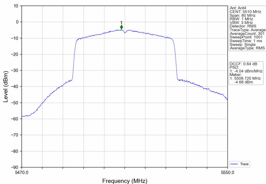
802.11ax(HEW40)_LCH_5510MHz_RU484_Left_Ant4_NTNV
