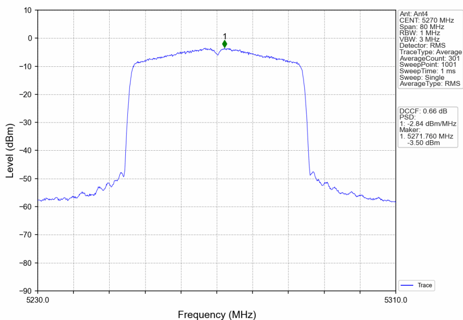
802.11ax(HEW40)_LCH_5270MHz_RU484_Left_Ant4_NTNV
