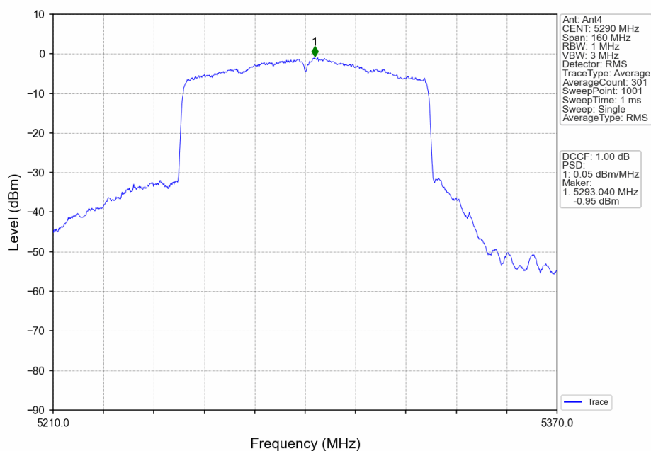
802.11ax(HEW80)_MCH_5290MHz_RU996_Left_Ant4_NTNV
