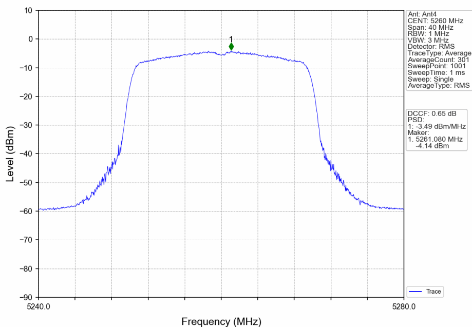
802.11ax(HEW20)_LCH_5260MHz_RU242_Left_Ant4_NTNV
