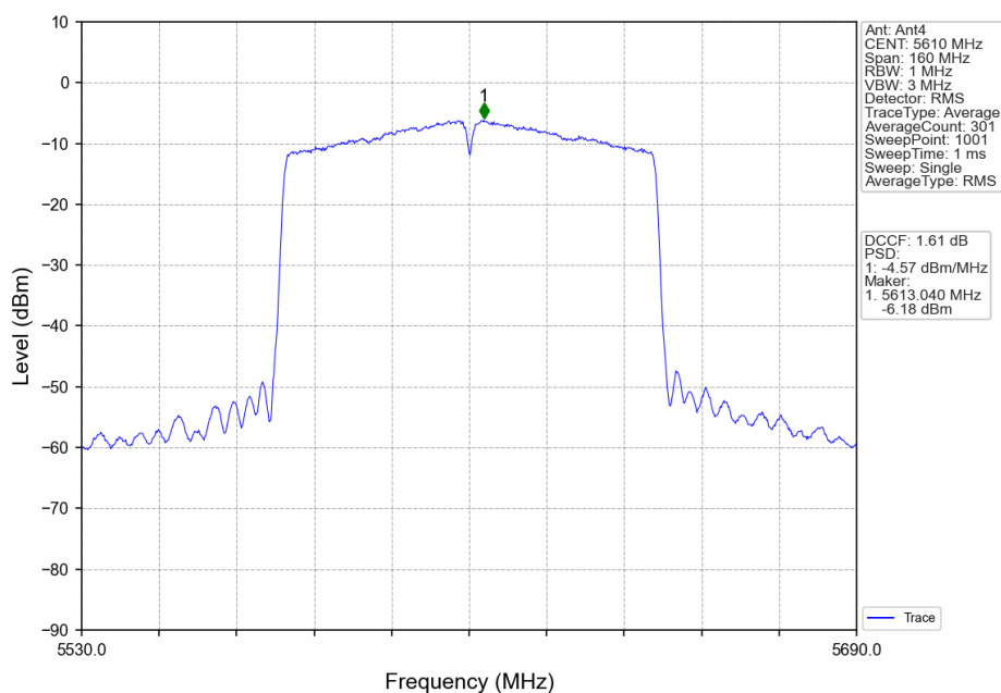
802.11ac(VHT80)_HCH_5610MHz_Ant4_NTNV
