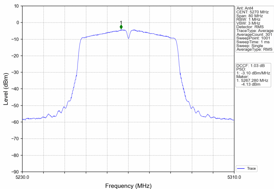
802.11ac(VHT40)_LCH_5270MHz_Ant4_NTNV
