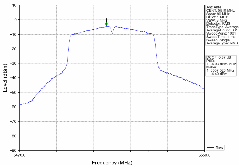
802.11n(HT40)_LCH_5510MHz_Ant4_NTNV
