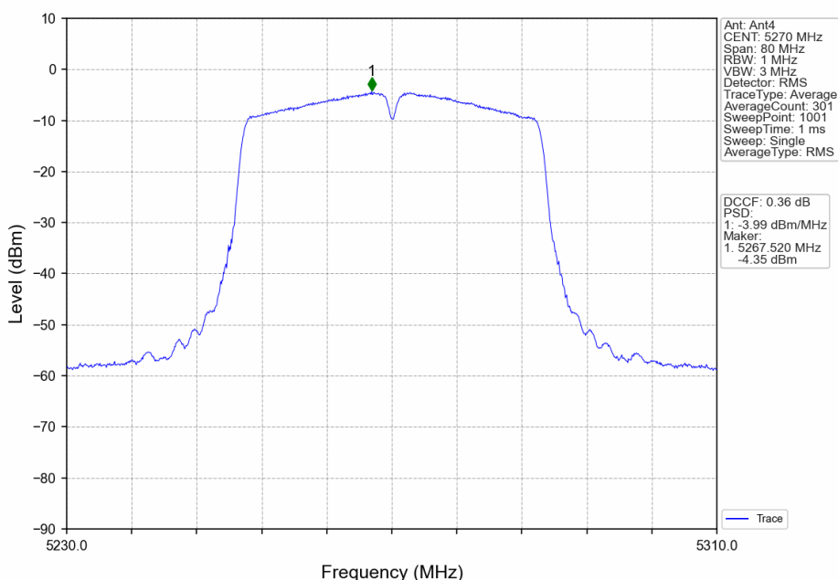
802.11n(HT40)_LCH_5270MHz_Ant4_NTNV
