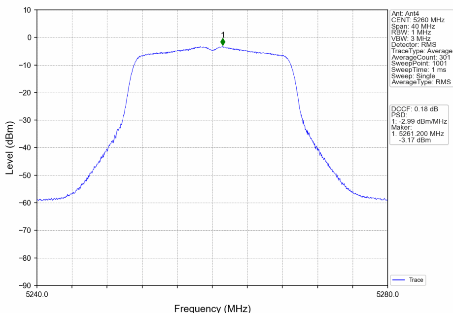
802.11n(HT20)_LCH_5260MHz_Ant4_NTNV
