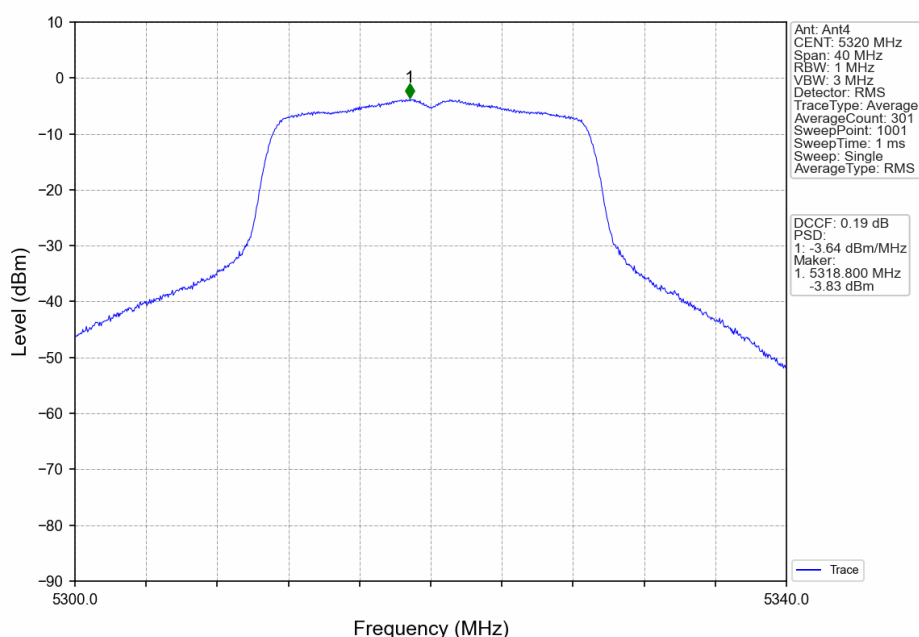
802.11n(HT20)_HCH_5320MHz_Ant4_NTNV
