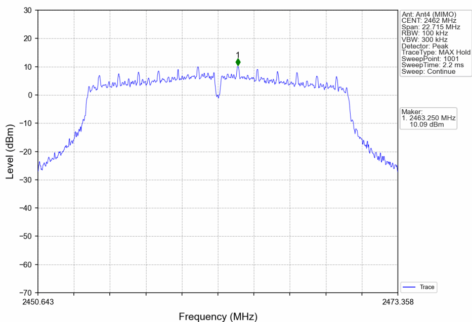
802.11g_HCH_2462MHz_Ant4 (MIMO)_NTNV
