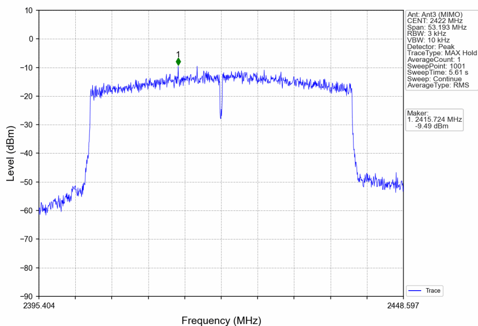
802.11ax(HEW40)_LCH_2422MHz_RU484_Left_Ant3 (MIMO)_NTNV
