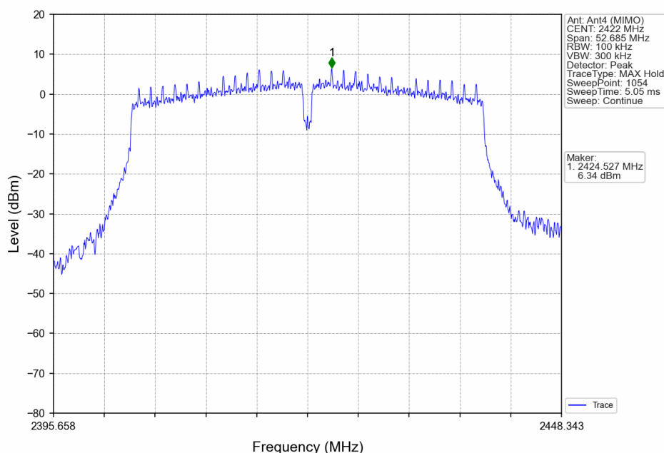
802.11n(HT40)_LCH_2422MHz_Ant4 (MIMO)_NTNV
