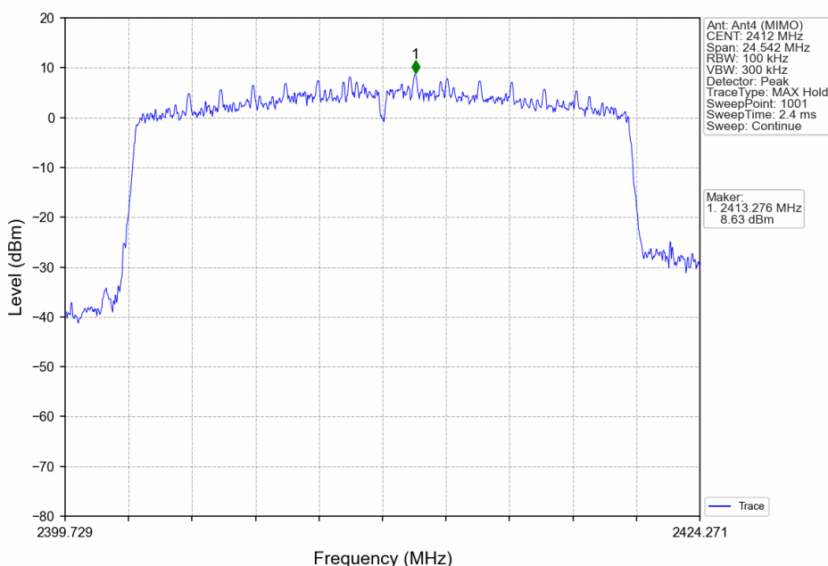
802.11ax(HEW20)_LCH_2412MHz_RU242_Left_Ant4 (MIMO)_NTNV
