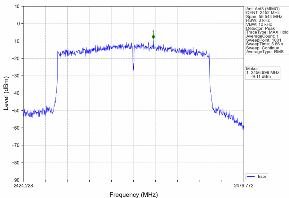
802.11ax(HEW40)_HCH_2452MHz_RU484_Left_Ant3 (MIMO)_NTNV
