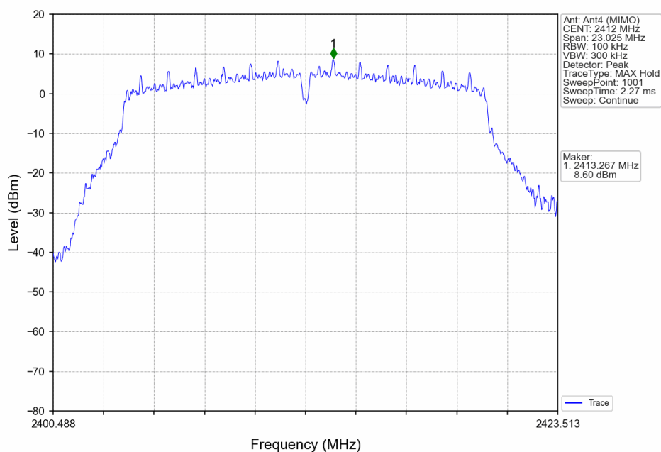
802.11g_LCH_2412MHz_Ant4 (MIMO)_NTNV
