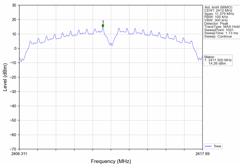
802.11b_LCH_2412MHz_Ant4 (MIMO)_NTNV
