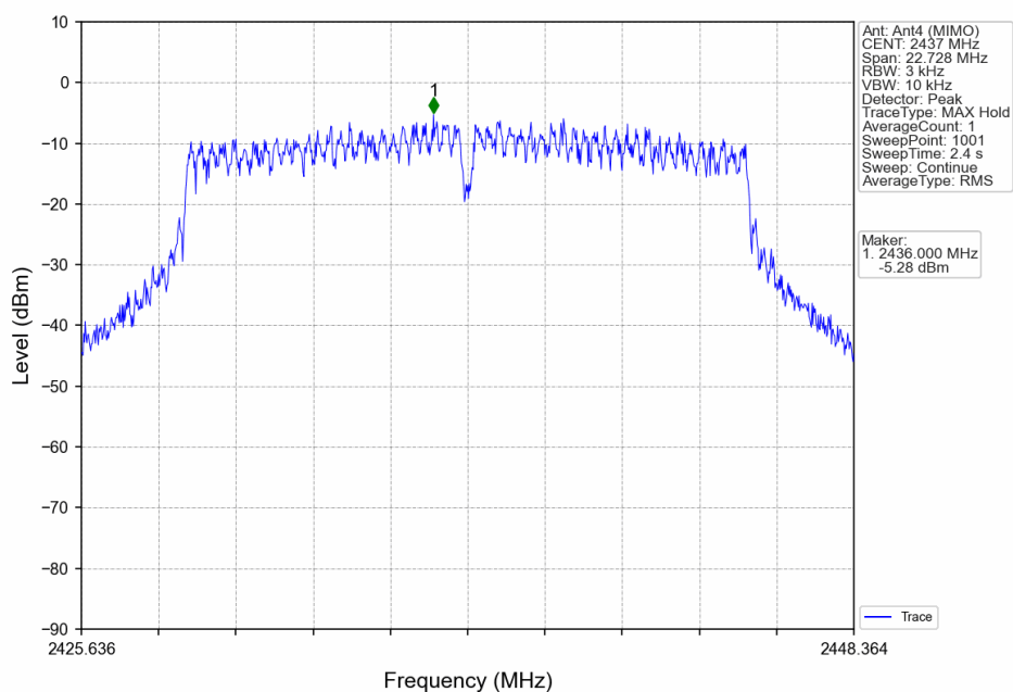
802.11g_MCH_2437MHz_Ant4 (MIMO)_NTNV
