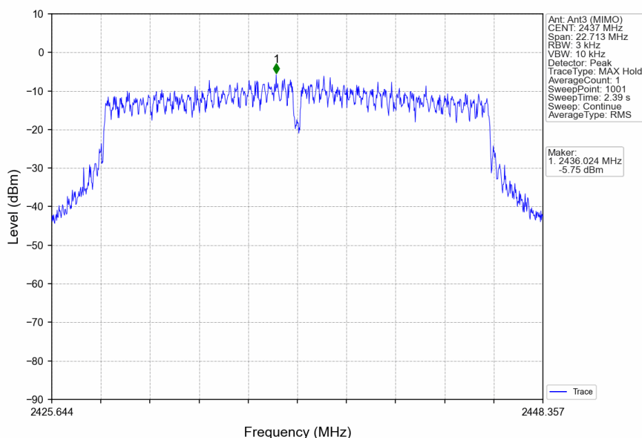
802.11n(HT20)_MCH_2437MHz_Ant3 (MIMO)_NTNV
