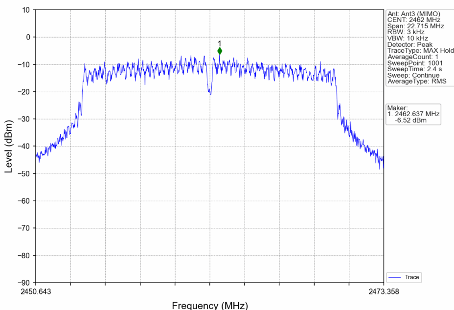
802.11g_HCH_2462MHz_Ant3 (MIMO)_NTNV
