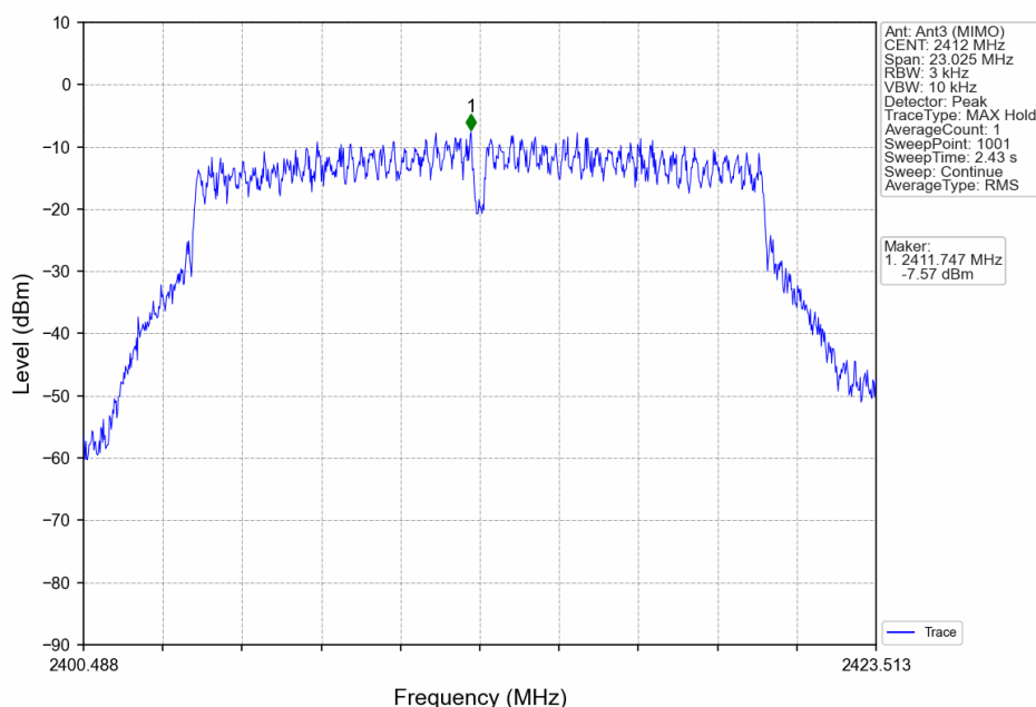
802.11g_LCH_2412MHz_Ant3 (MIMO)_NTNV
