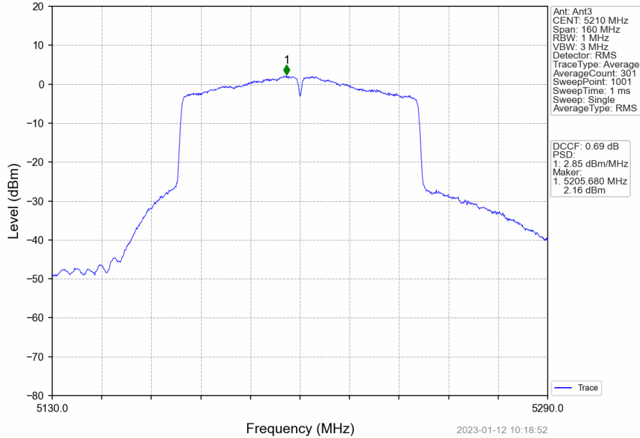
802.11ac(VHT80)_MCH_5210MHz_MIMO_NTNV
