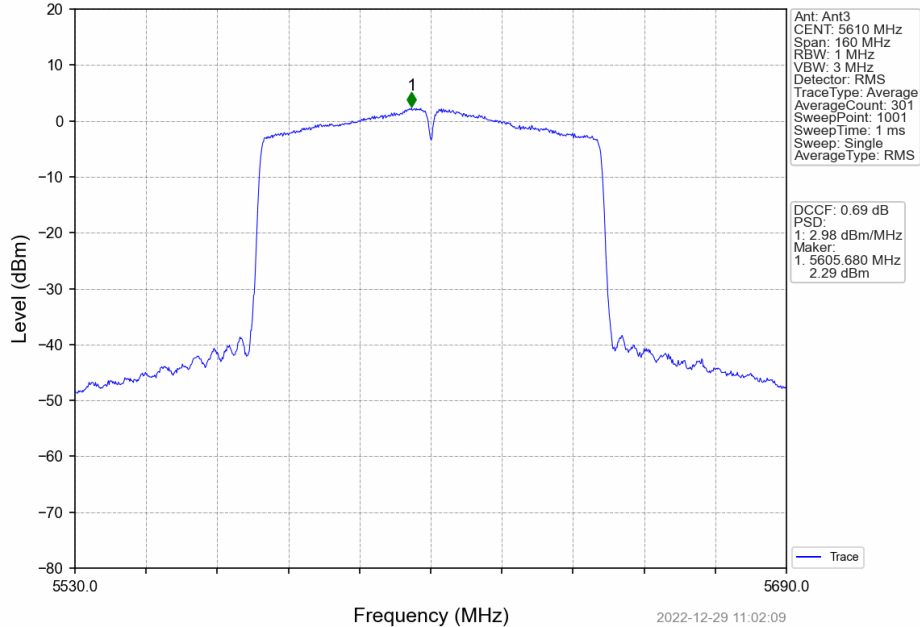
802.11ac(VHT80)_HCH_5610MHz_MIMO_NTNV
