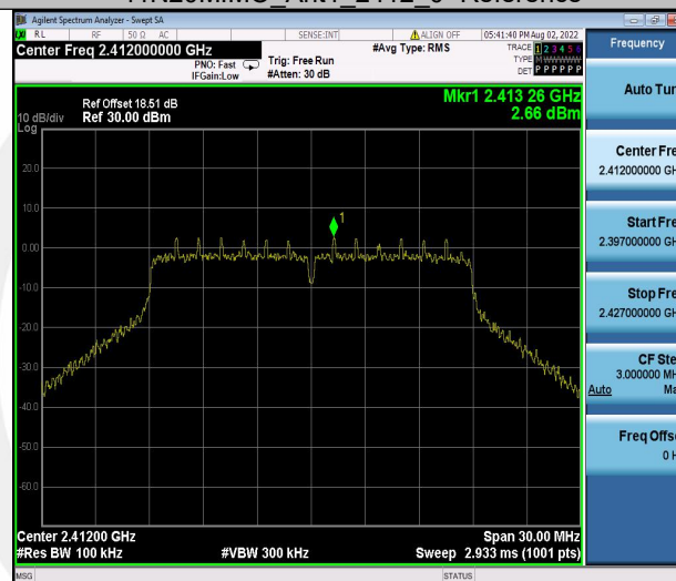
11N20MIMO_Ant1_2412_0~Reference
