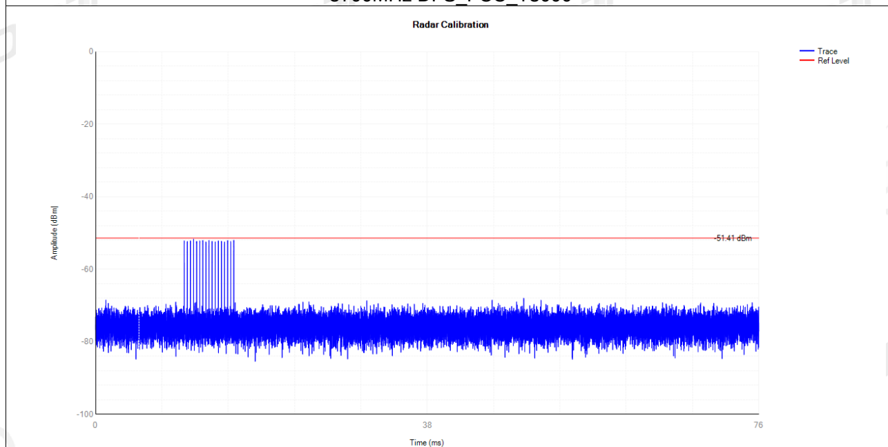
5700MHz DFS_FCC_T4000
