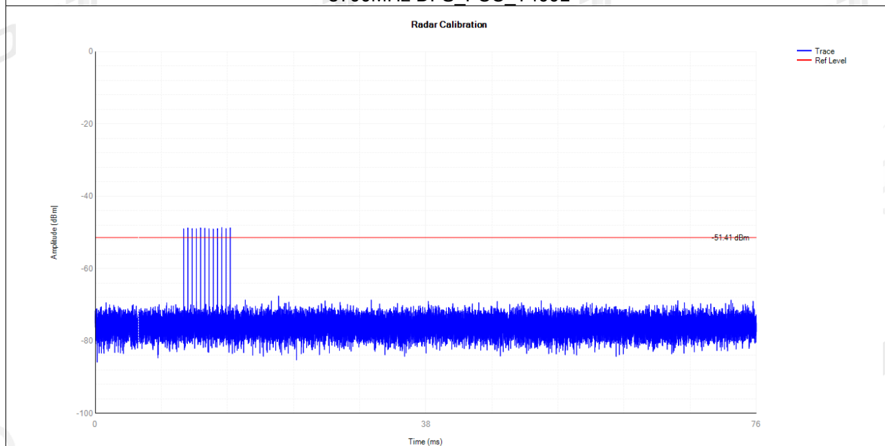
5700MHz DFS_FCC_T5000
