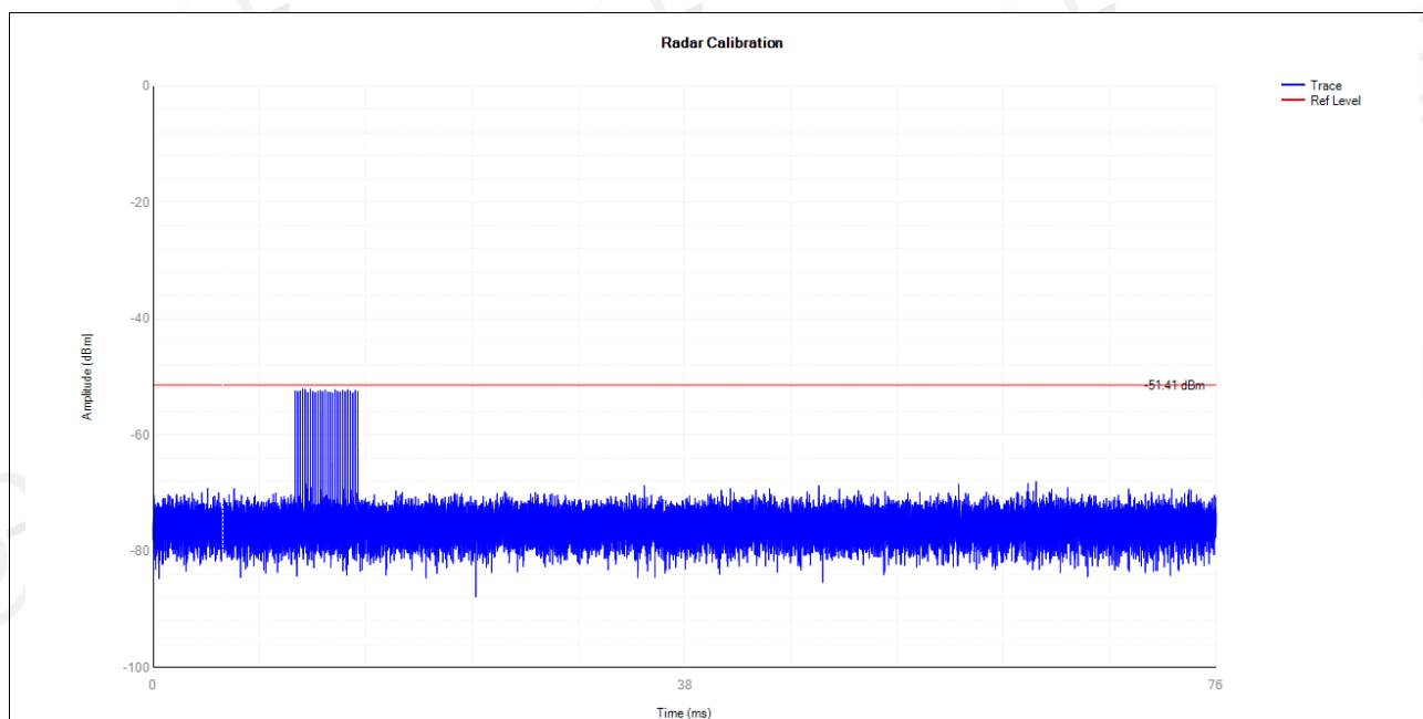
5700MHz DFS_FCC_T3000
