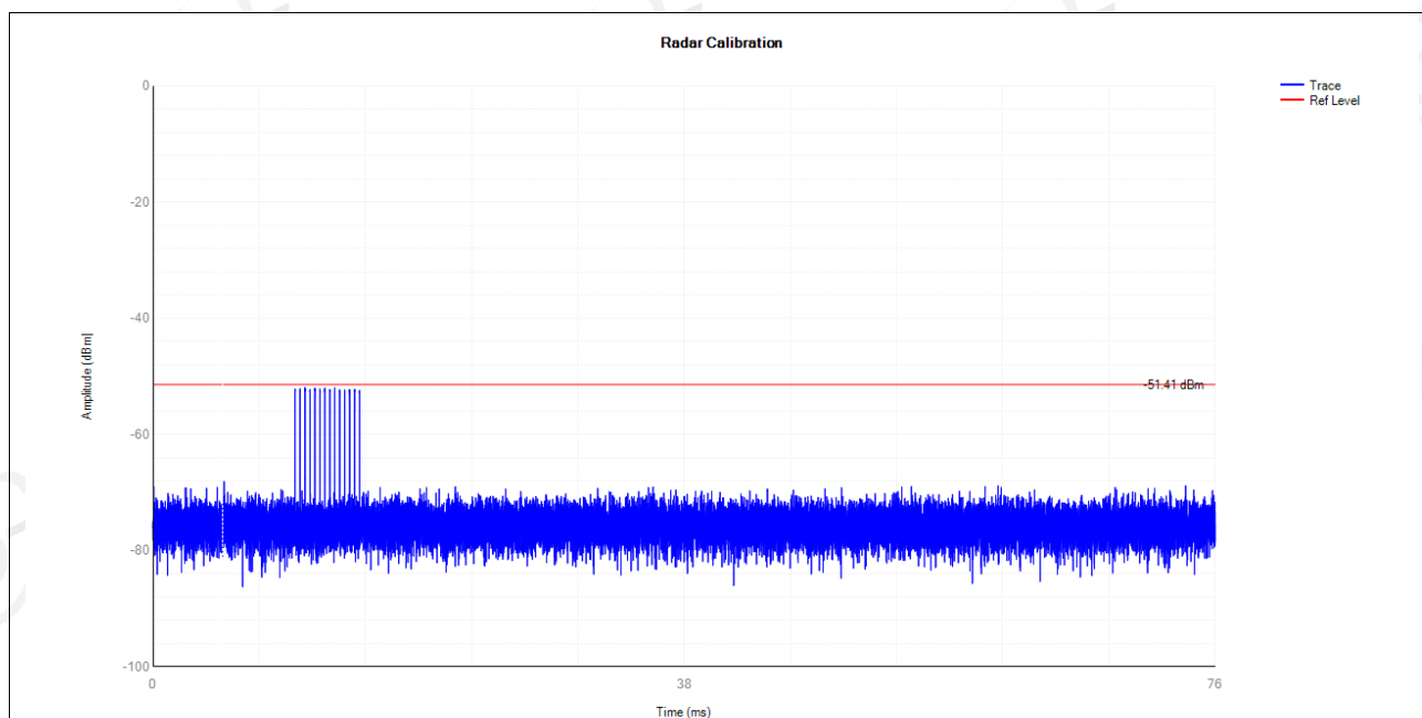
5700MHz DFS_FCC_T4001
