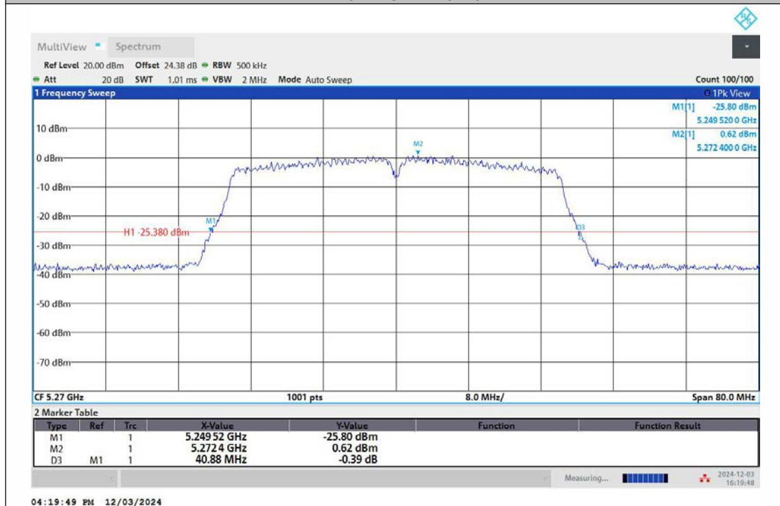
11N40MIMO-Ant2-5270
