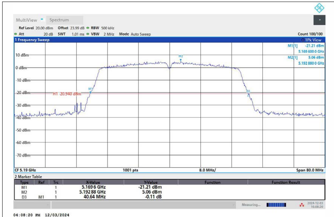
11N40MIMO-Ant1-5190
