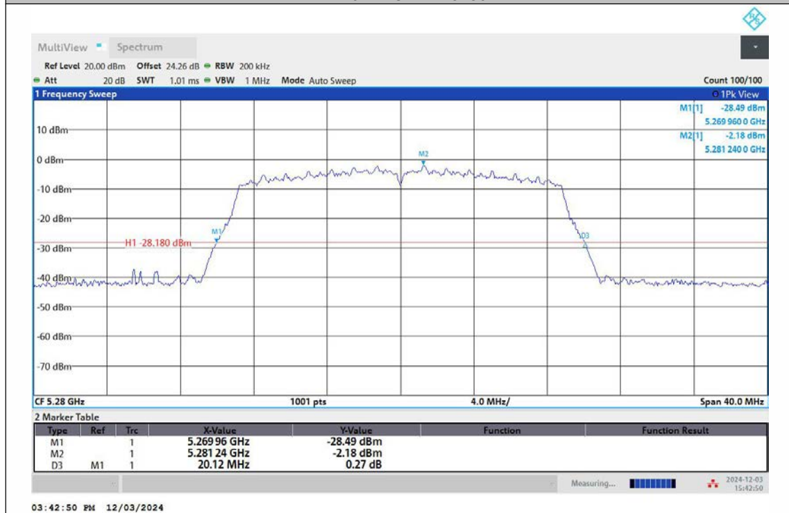
11N20MIMO-Ant2-5280
