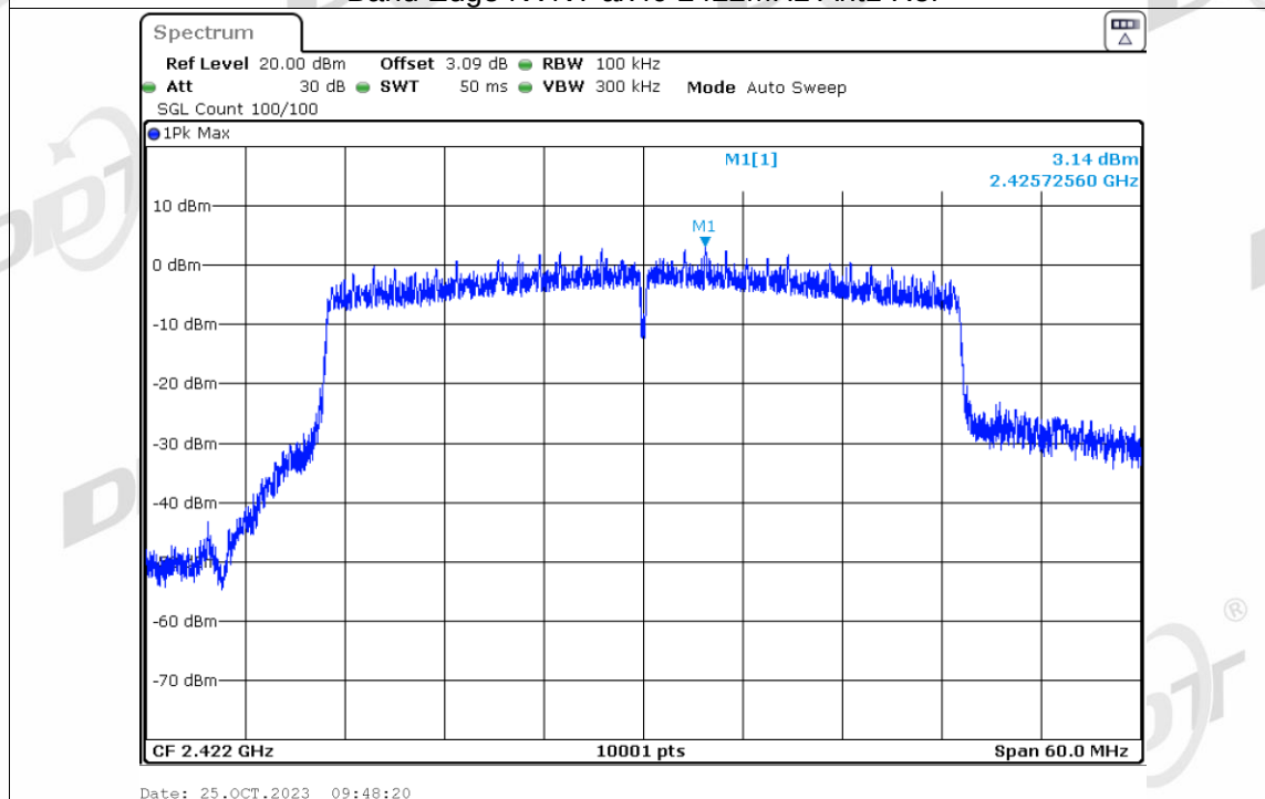
Band Edge NVNT ax40 2422MHz Ant1 Emission
