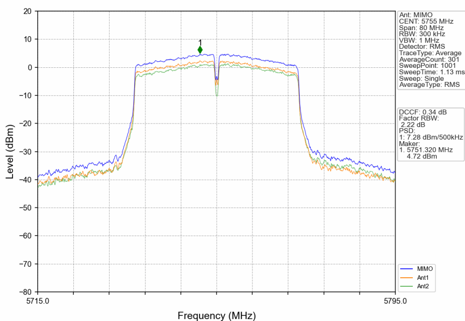
802.11ac(VHT40)_LCH_5755MHz_MIMO_NTNV
