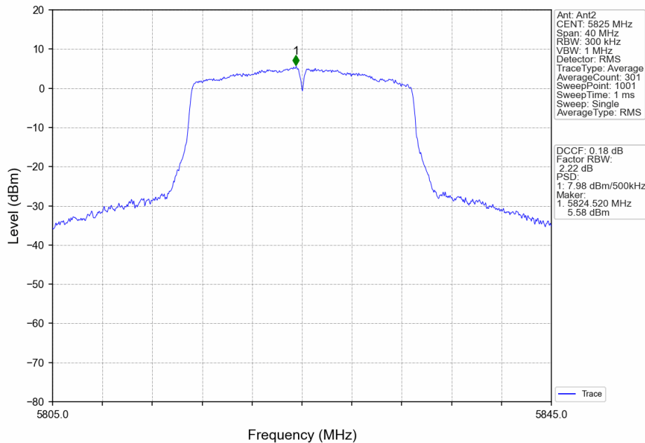
802.11n(HT20)_HCH_5825MHz_MIMO_NTNV
