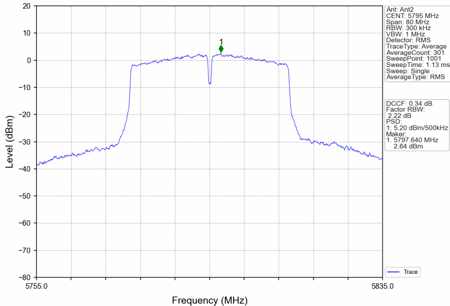
802.11n(HT40)_HCH_5795MHz_MIMO_NTNV
