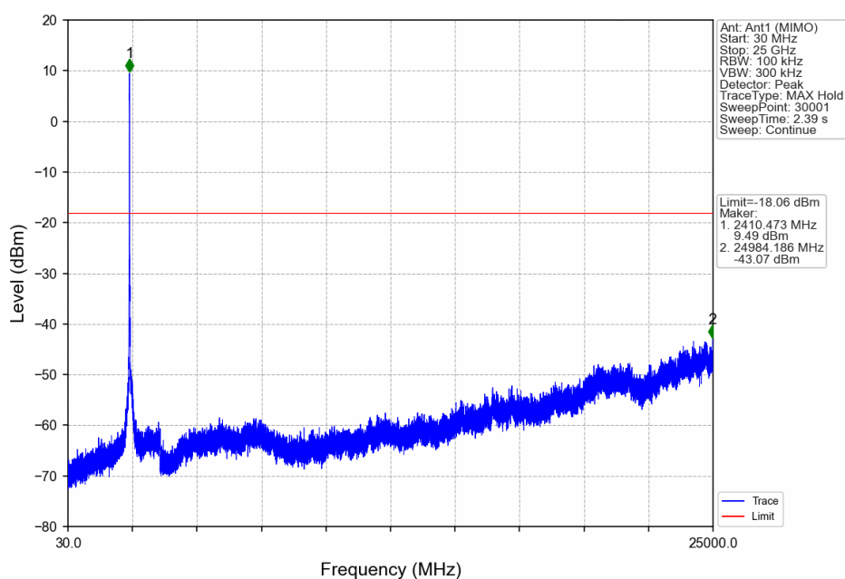
802.11g_LCH_2412MHz_Ant1 (MIMO)_NTNV
