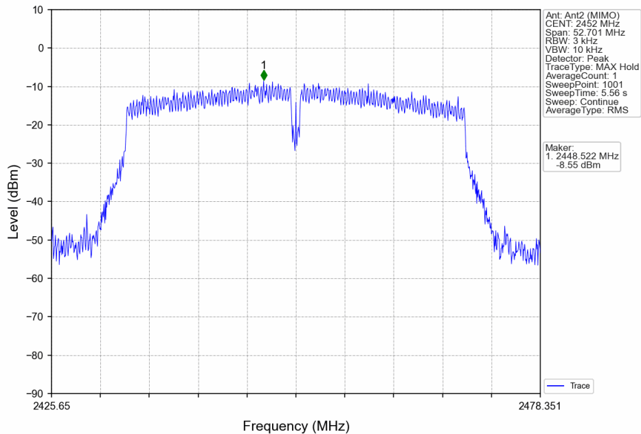
802.11n(HT40)_HCH_2452MHz_MIMO_NTNV
