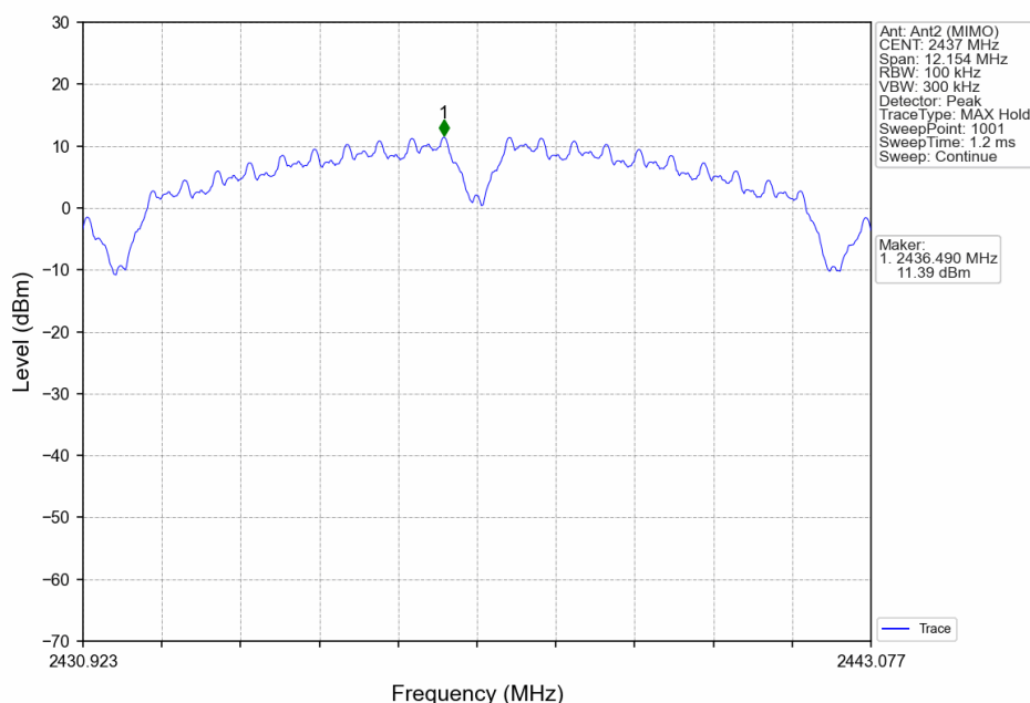
802.11b_MCH_2437MHz_Ant2 (MIMO)_NTNV
