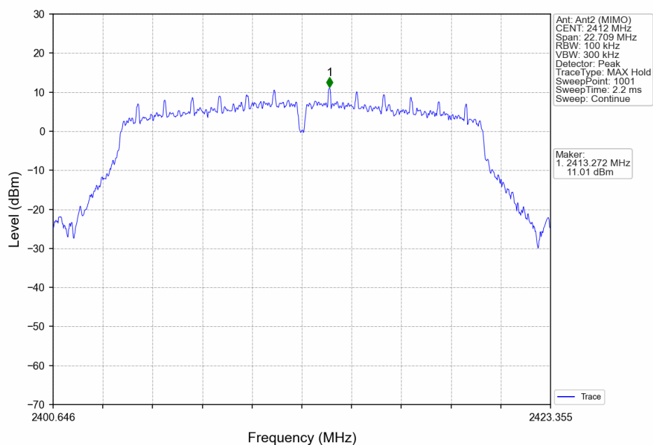
802.11g_LCH_2412MHz_Ant2 (MIMO)_NTNV
