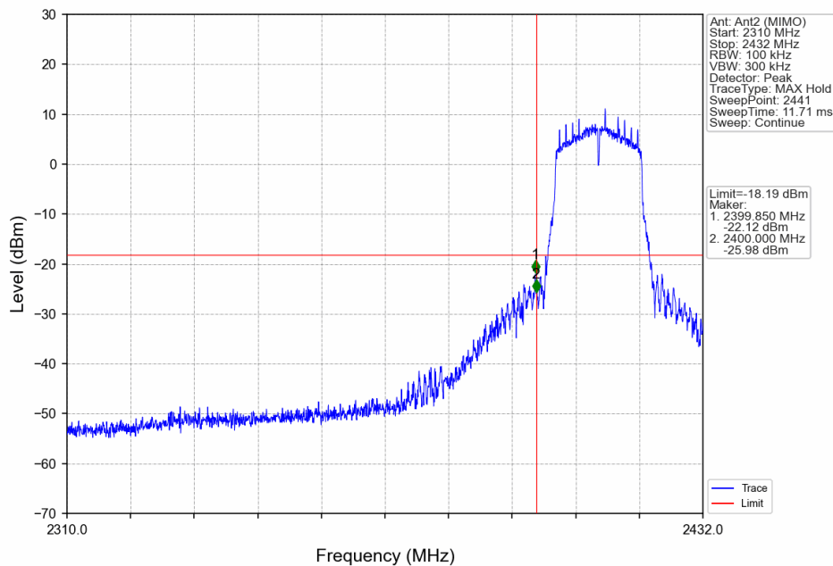
802.11g_LCH_2412MHz_Ant2 (MIMO)_NTNV
