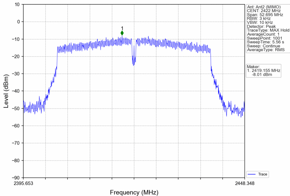
802.11n(HT40)_LCH_2422MHz_MIMO_NTNV
