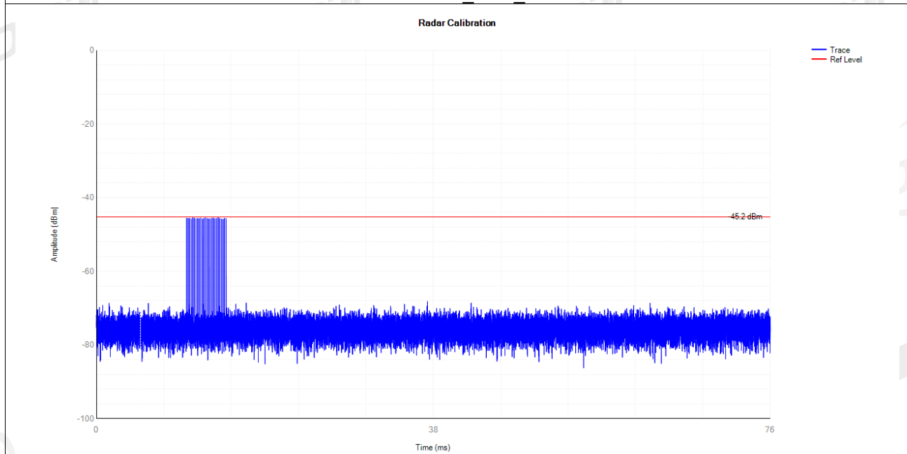
5700MHz DFS_FCC_T3000
