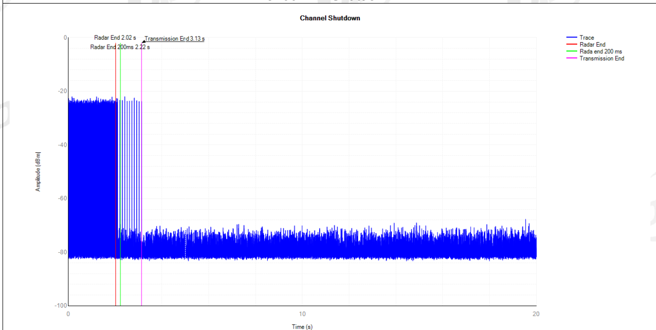
5700MHz Shutdown
