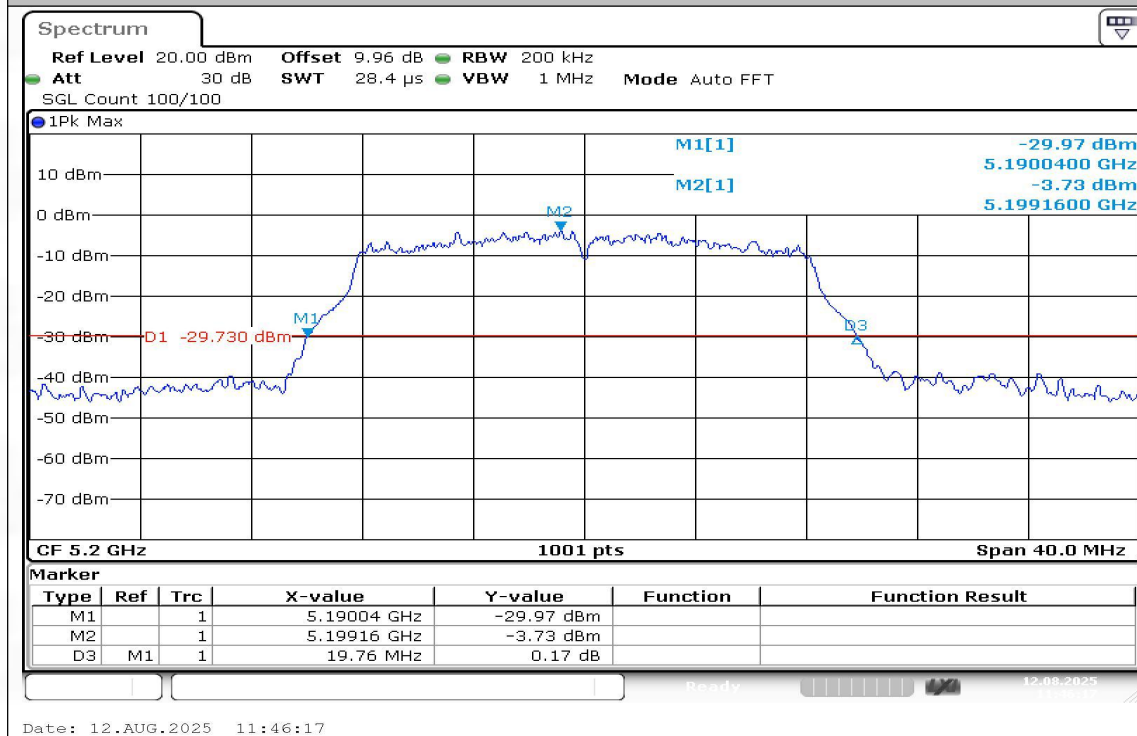
11A-Ant1-5200
