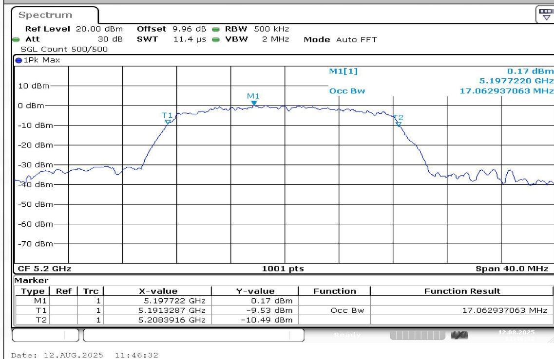
11A-Ant1-5200
