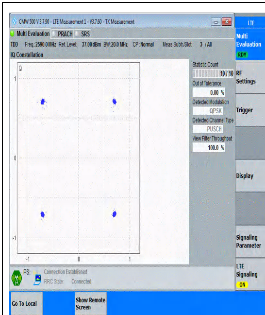
Band41(2535-2655)-20MHz-QPSK-40590-100RB #0-PASS
