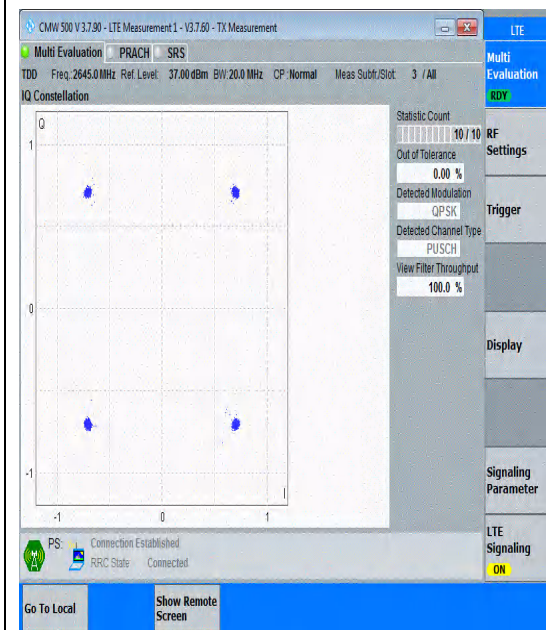
Band41(2535-2655)-20MHz-QPSK-41140-100RB #0-PASS
