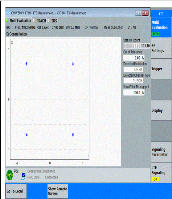
Band25-3MHz-QPSK-26365-15RB#0-PASS
