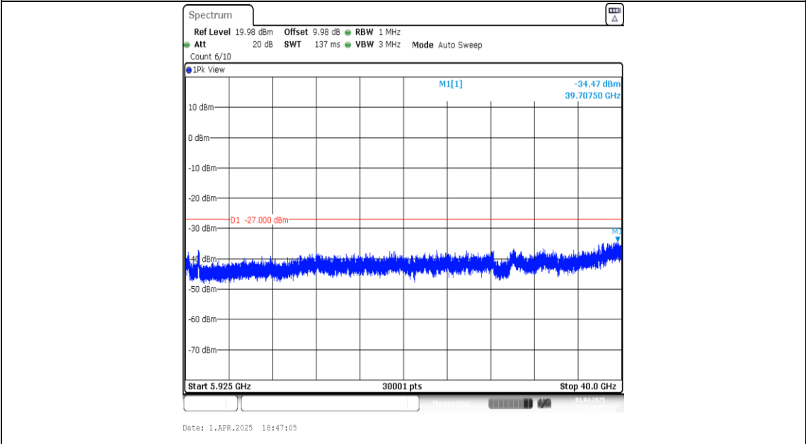
11AC80SISO-Ant1-5775-5925~40000-PASS
