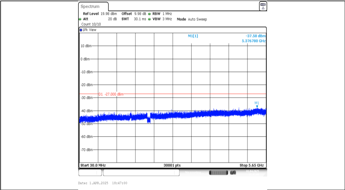
11AC80SISO-Ant1-5775-30~5650-PASS
