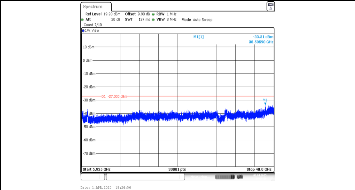
11AC20SISO-Ant1-5785-5925~40000-PASS
