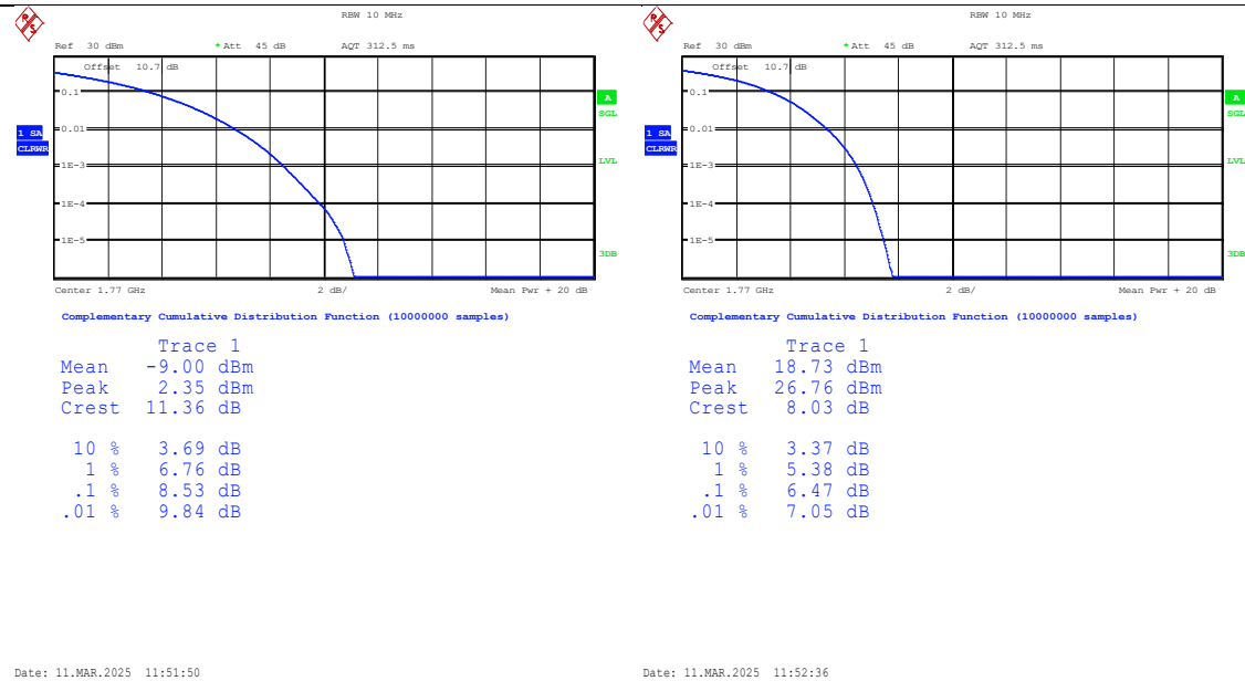
Band66-20MHz-QPSK-132572-1RB#0-PASS
