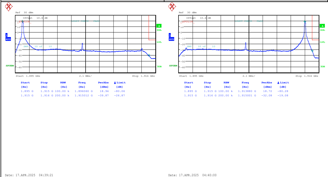
Band25-20MHz-QPSK-26590-1RB#99-PASS
