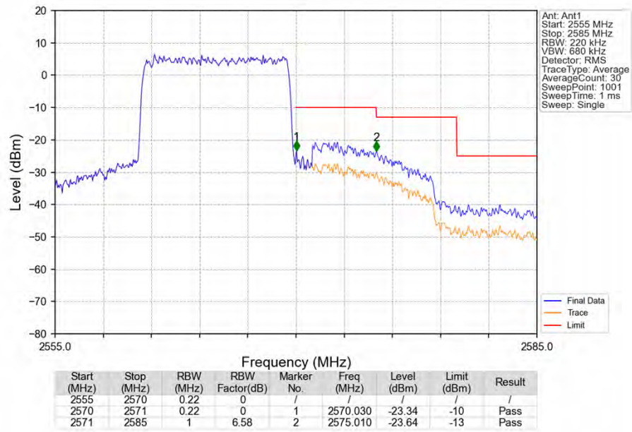
Band7_10MHz_QPSK_HCH_2565MHz_RB_50_0_NTNV
