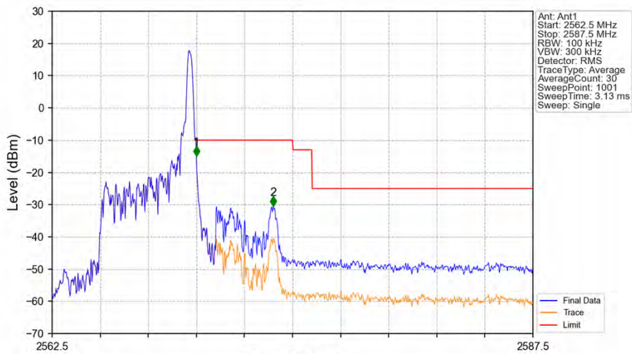
Band7_5MHz_QPSK_HCH_2567.5MHz_RB_1_24_NTNV
