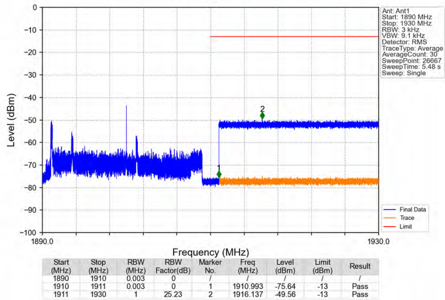
Band2_20MHz_QPSK_HCH_1900MHz_RB_1_99_NTNV
