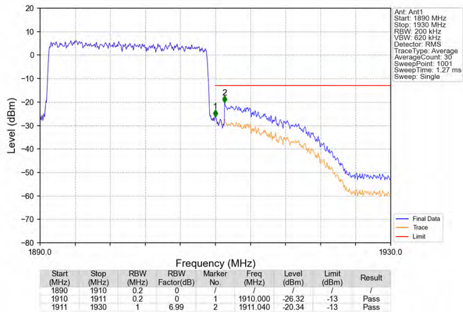
Band2_20MHz_QPSK_HCH_1900MHz_RB_100_0_NTNV
