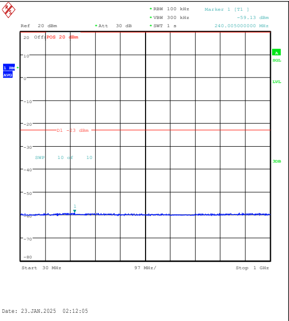
Band25-20MHz-16QAM-26365-1RB#0-30~1000-P ASS
