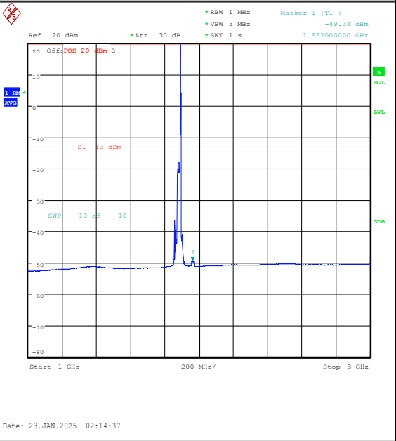
Band25-20MHz-16QAM-26365-1RB#99-1000~3000-PASS
