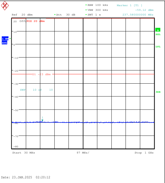
Band25-20MHz-QPSK-26590-1RB#99-30~1000-P ASS
