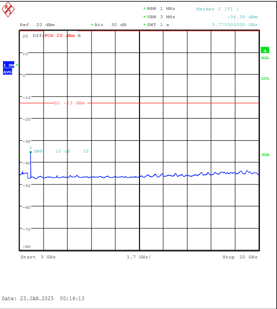
Band25-10MHz-QPSK-26365-1RB#49-3000~2000 0-PASS
