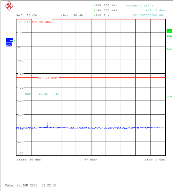
Band25-20MHz-QPSK-26590-100RB#0-30~1000 -PASS
