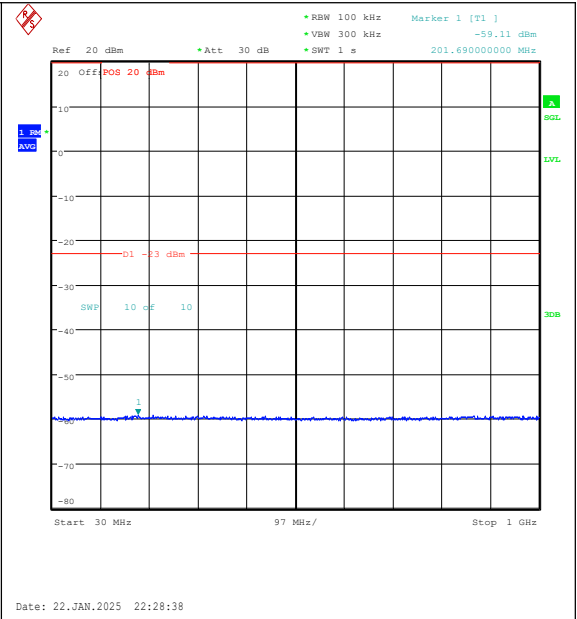
Band25-3MHz-16QAM-26675-15RB#0-30~1000-P ASS
