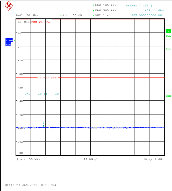
Band25-15MHz-QPSK-26115-75RB#0-30~1000-P ASS
