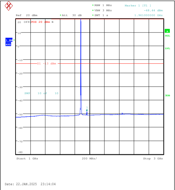
Band25-5MHz-QPSK-26365-1RB#0-1000~3000-P ASS
