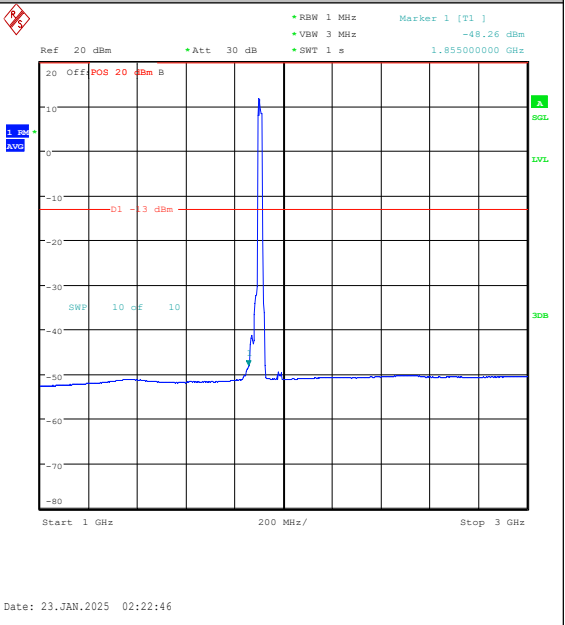
Band25-20MHz-QPSK-26590-100RB#0-1000~300 0-PASS
