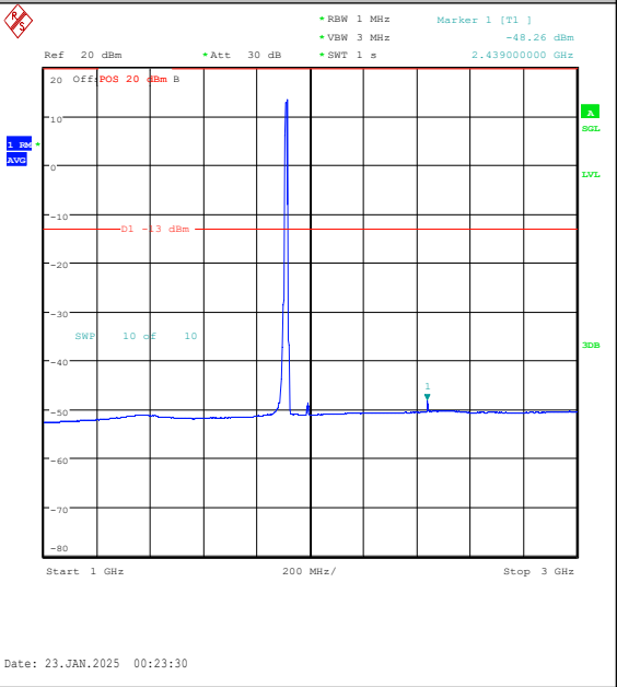
Band25-10MHz-QPSK-26640-50RB#0-1000~3000 -PASS
