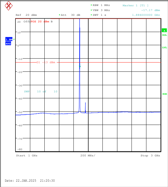
Band25-1.4MHz-QPSK-26365-1RB#5-1000~3000 -PASS
