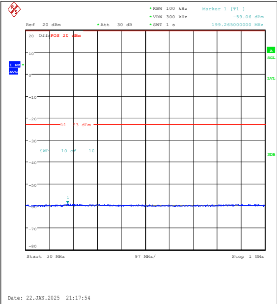
Band25-1.4MHz-QPSK-26365-1RB#0-30~1000-P ASS
