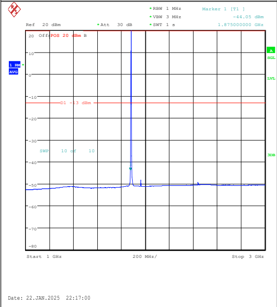
Band25-3MHz-16QAM-26365-1RB#0-1000~3000 -PASS
