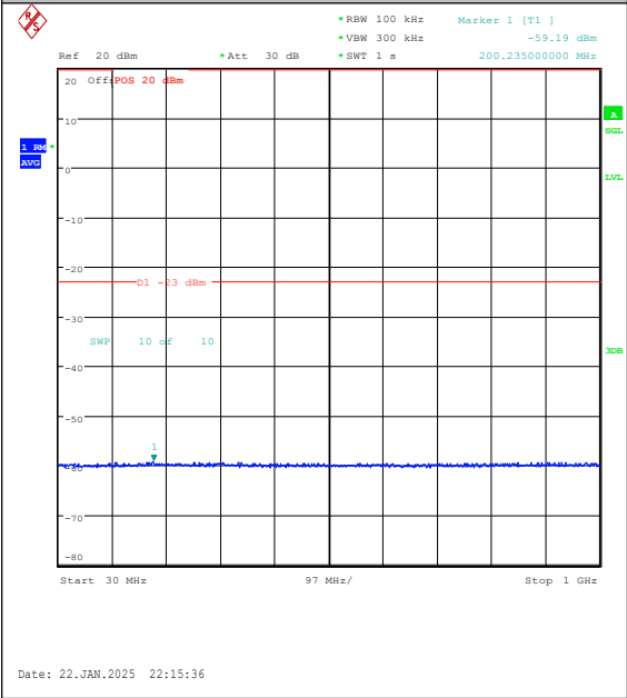
Band25-3MHz-QPSK-26365-1RB#0-30~1000-PA
