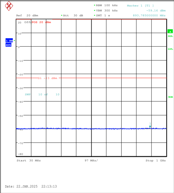
Band25-3MHz-QPSK-26055-15RB#0-30~1000-P ASS
