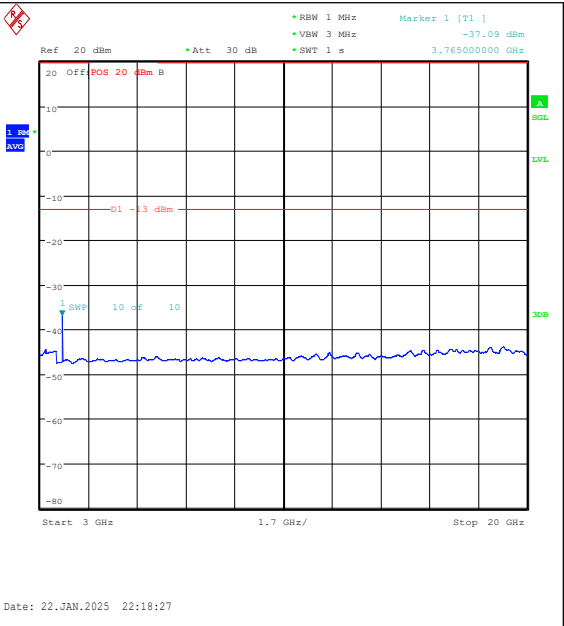
Band25-3MHz-QPSK-26365-1RB#14-3000~20000 -PASS
