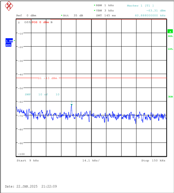
Band25-1.4MHz-QPSK-26365-6RB#0-0.009~0.15 -PASS
