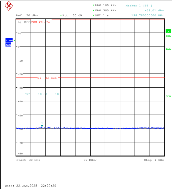
Band25-3MHz-QPSK-26365-15RB#0-30~1000-P ASS
