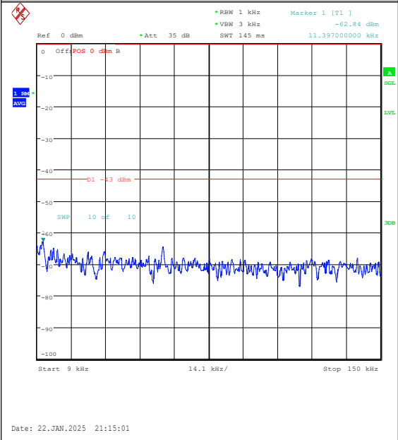
Band25-1.4MHz-QPSK-26047-6RB#0-0.009~0.15 -PASS
