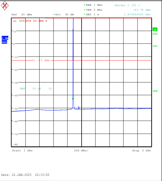
Band25-3MHz-QPSK-26365-1RB#0-1000~3000-P
