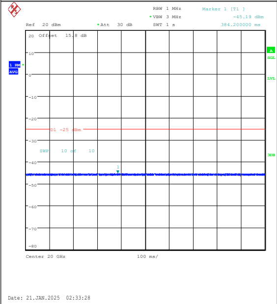
Band7-10MHz-QPSK-20800-50RB#0-20000~270 00-PASS
