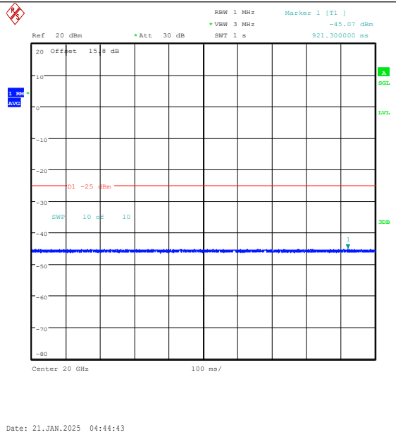
Band7-20MHz-QPSK-20850-1RB#99-20000~2700 0-PASS
