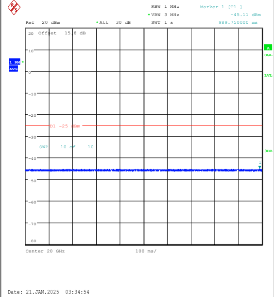
Band7-15MHz-QPSK-20825-1RB#0-20000~2700 0-PASS
