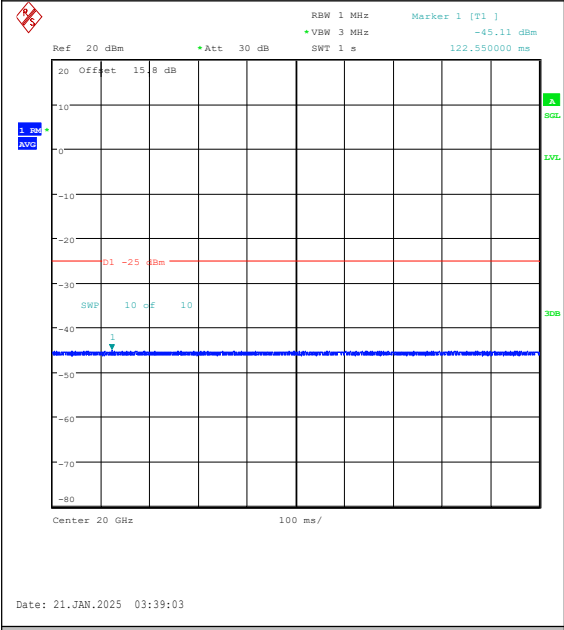
Band7-15MHz-16QAM-20825-1RB#74-20000~27000-PASS
