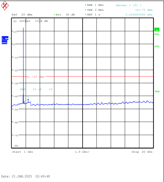
Band7-10MHz-QPSK-21400-50RB#0-1000~20000 -PASS
