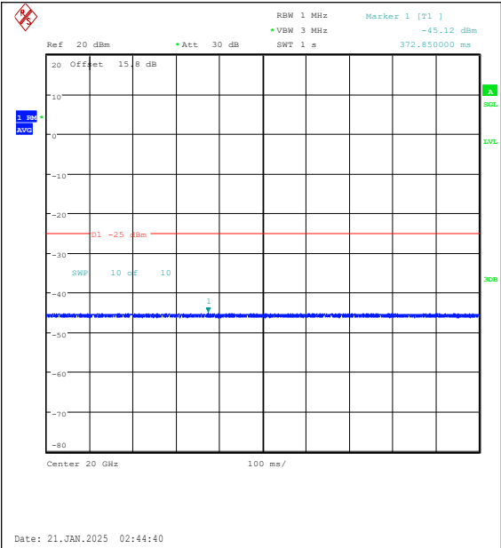
Band7-10MHz-QPSK-21400-1RB#0-20000~2700 0-PASS
