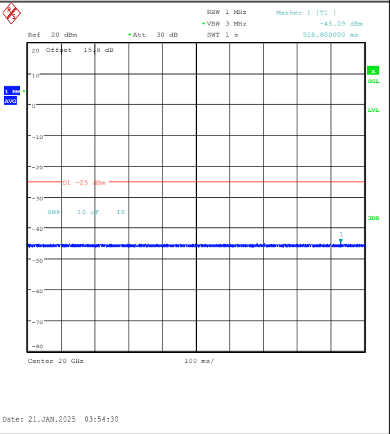
Band7-15MHz-QPSK-21375-1RB#74-20000~2700 0-PASS
