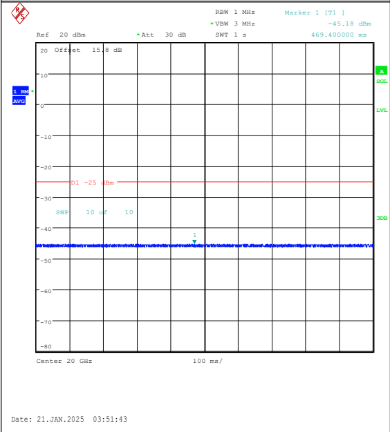
Band7-15MHz-QPSK-21375-1RB#0-20000~2700 0-PASS
