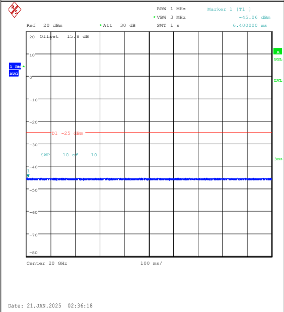
Band7-10MHz-QPSK-21100-1RB#0-20000~2700 0-PASS
