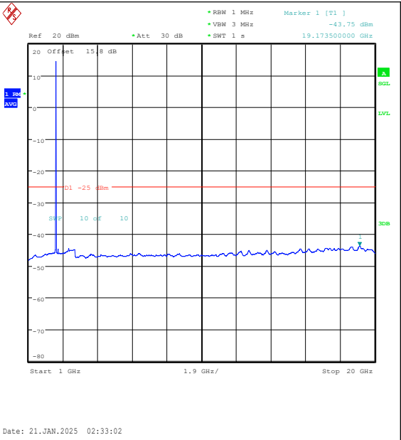
Band7-10MHz-QPSK-20800-50RB#0-1000~20000 -PASS
