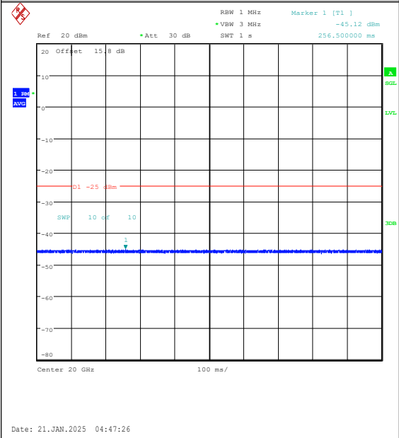
Band7-20MHz-QPSK-20850-100RB#0-20000~27000-PASS
